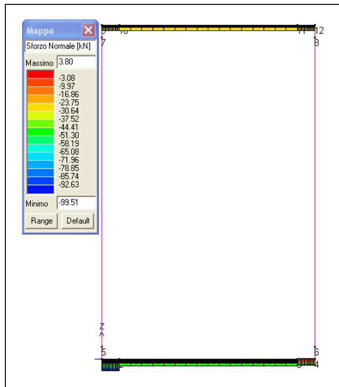
Figura 13-5 Involuppo azione assiale SLU nelle solette
