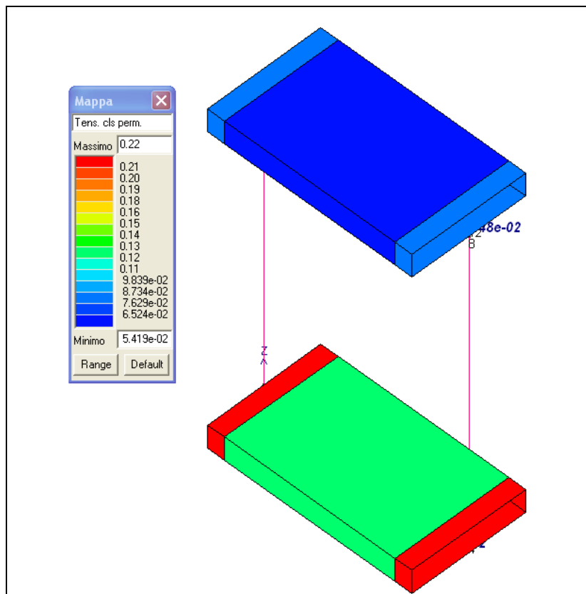
Figura 10-14 Verifica delle tensioni cls in esercizio (permanente)
