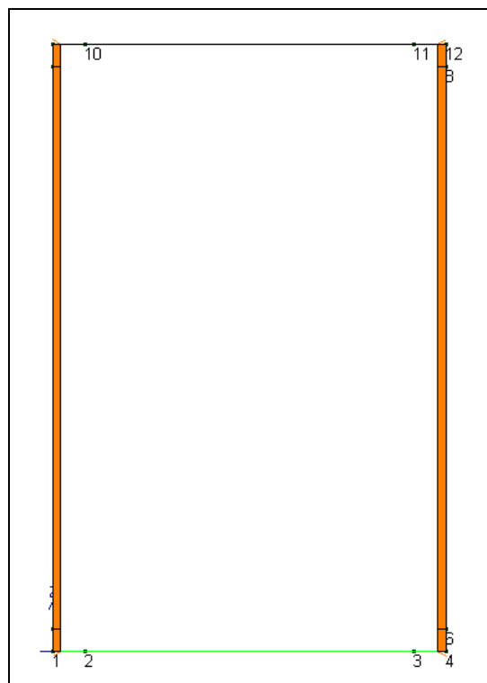
Figura 5-10 Carico veicoli tandem e 9 \text{ kN/m}^2 a tergo del piedritto sx e dx
