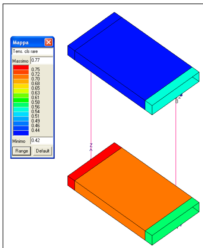
Figura 10-12 Verifica delle tensioni cls in esercizio (rara)
