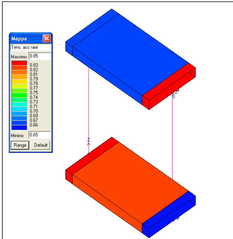
Figura 10-13 Verifica delle tensioni acciaio in esercizio (rara)
