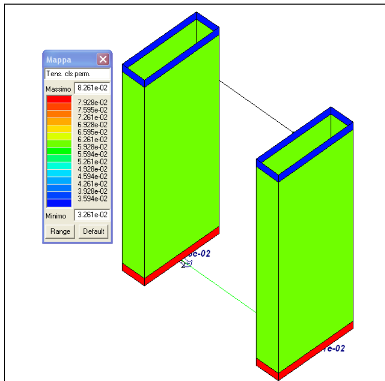
Figura 10-21 Verifica delle tensioni cls in esercizio (permanente)
