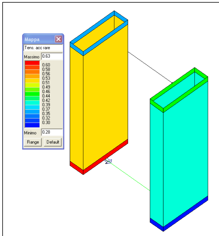
Figura 10-20 Verifica delle tensioni acciaio in esercizio (rara)
