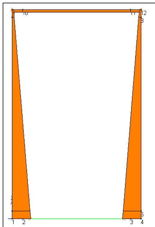
Figura 5-2 Carico permanente portato (rilevato e carreggiata stradale)
