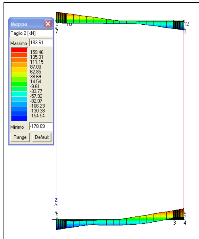
Figura 13-3 Involuppo azione tagliante SLU nelle solette
