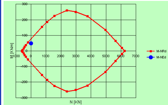
Figura 10-15 SLU pressoflessione piedritto
