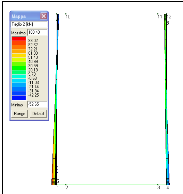
Figura 13-4 Involuppo azione tagliante SLU nei piedritti
