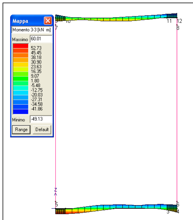
Figura 13-1 Involucro momento flettente SLU nelle solette
