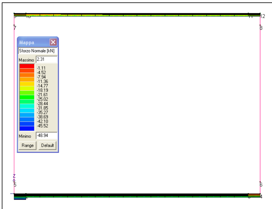
Figura 13-5 Involuppo azione assiale SLU nelle solette
