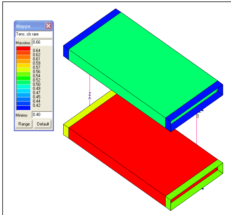
Figura 10-12 Verifica delle tensioni cls in esercizio (rara)
