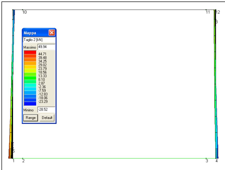
Figura 13-4 Involuppo azione tagliante SLU nei pedritti
