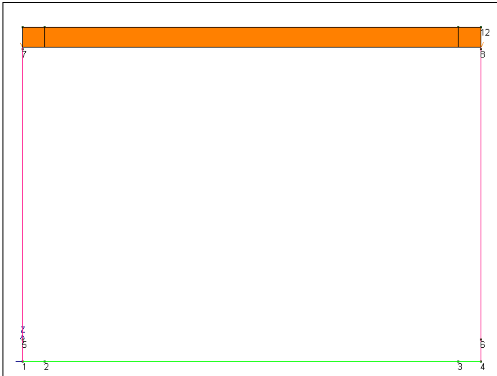
Figura 5-9 Carico veicoli tandem e 9 \text{ kN/m}^2 centrato
