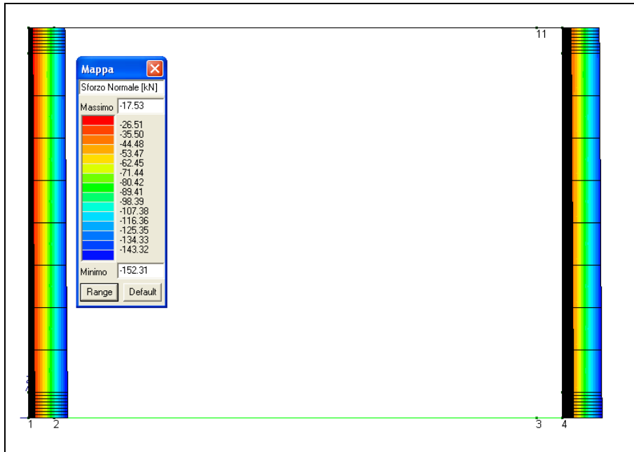
Figura 13-6 Involuppo azione assiale SLU nei piedritti
