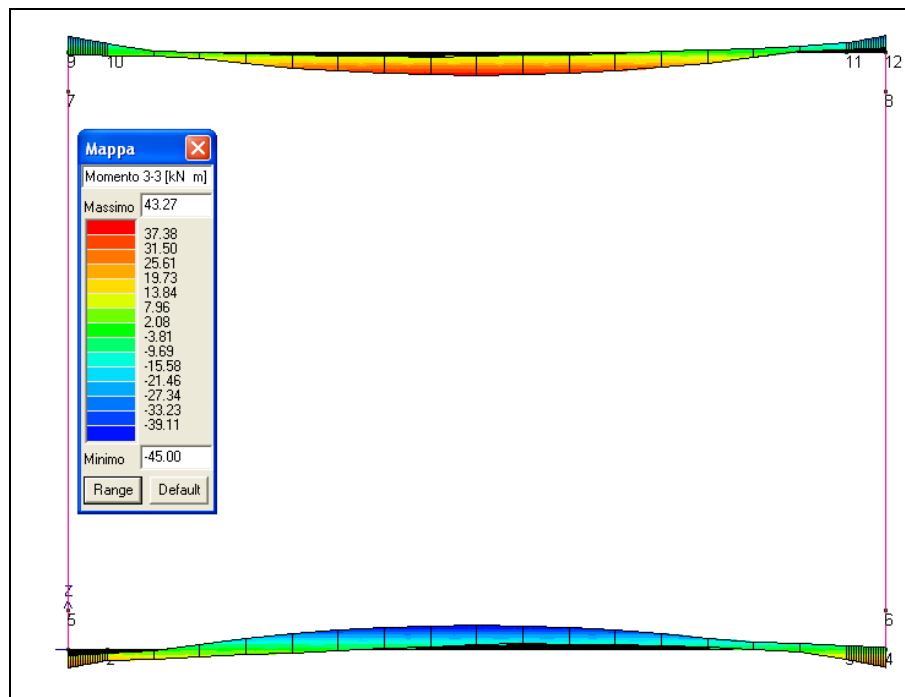
Figura 13-1 Involucro momento flettente SLU nelle solette
