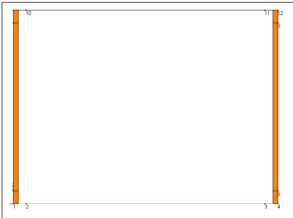
Figura 5-10 Carico veicoli tandem e 9 \text{ kN/m}^2 a tergo del piedritto sx e dx
