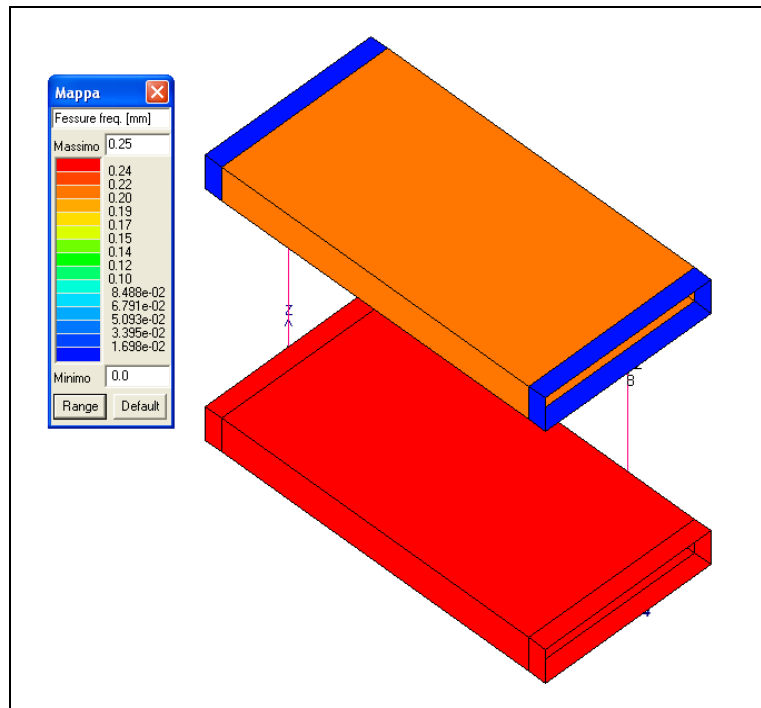
Figura 10-10 Verifica delle fessure nelle solette (frequente)
