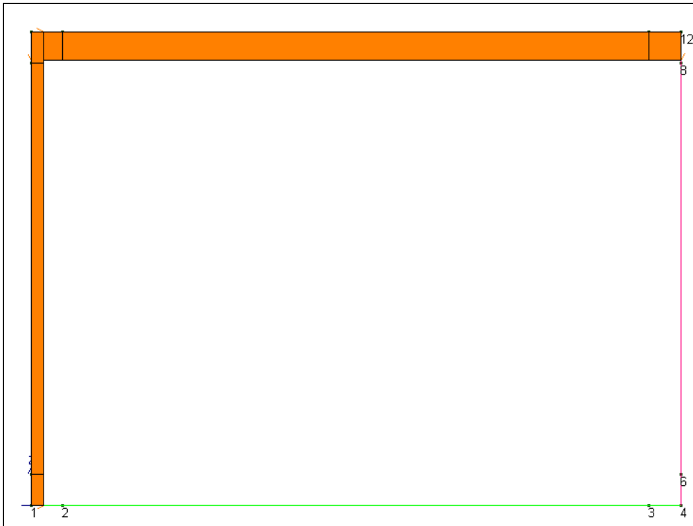
Figura 5-11 Carico veicoli tandem e 9 \text{ kN/m}^2 a tergo del piedritto sx e centrato
