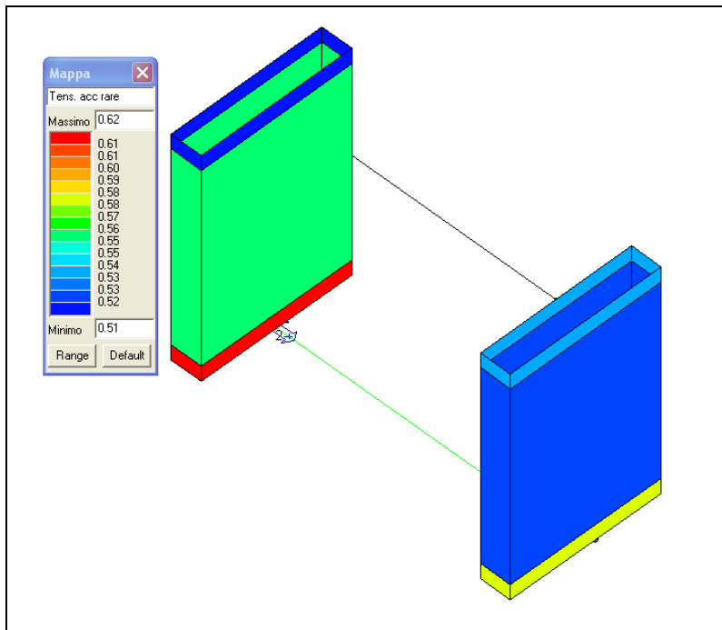
Figura 10-20 Verifica delle tensioni acciaio in esercizio (rara)
