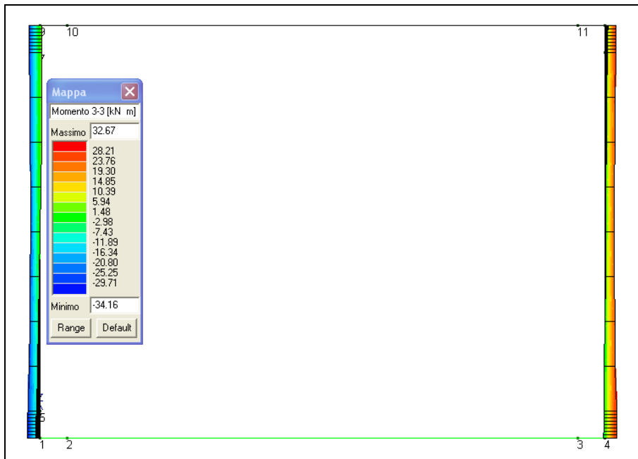
Figura 13-2 Involuppo momento flettente SLU nei piedritti
