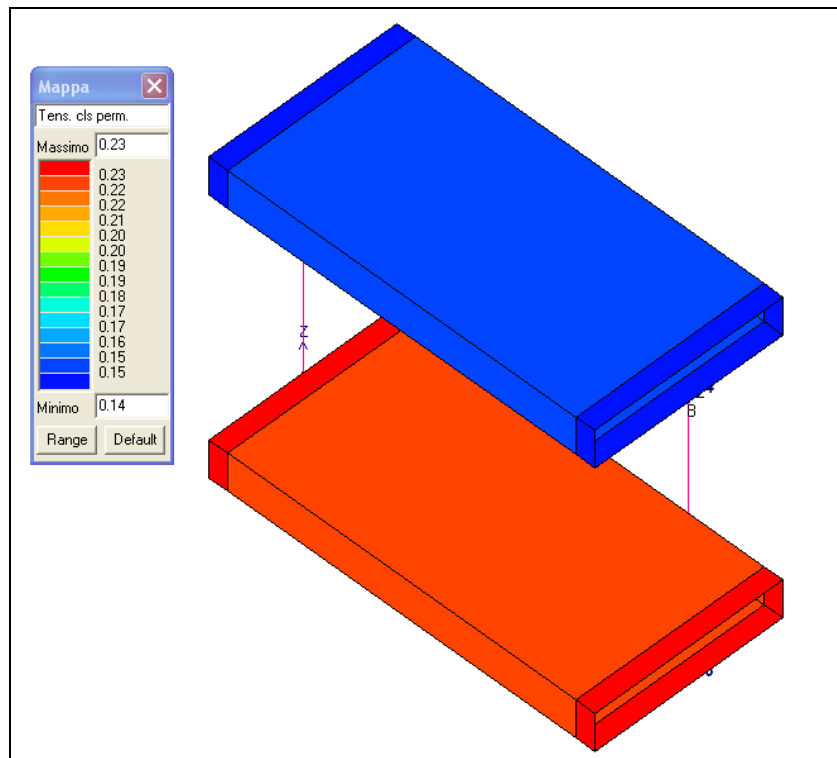
Figura 10-14 Verifica delle tensioni cls in esercizio (permanente)
