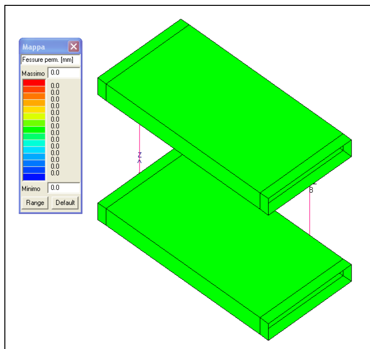
Figura 10-11 Verifica delle fessure nelle solette (quasi permanente)
