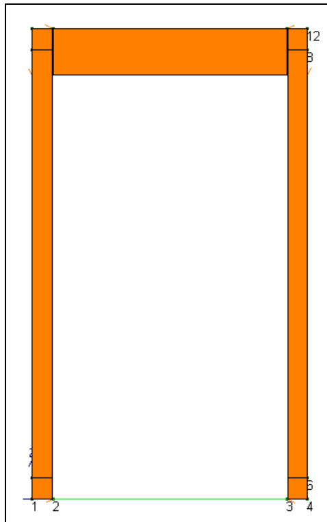
Figura 5-3 Carico veicoli uniforme 20 kN/m 2 (sovraccarico stradale sopra scatolare)
