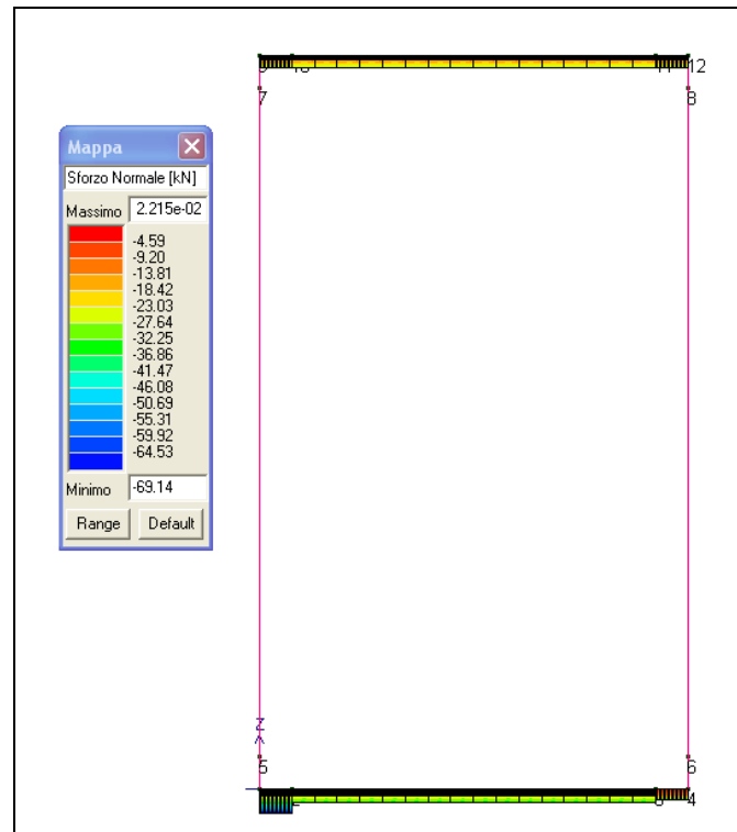
Figura 13-5 Involuppo azione assiale SLU nelle solette
