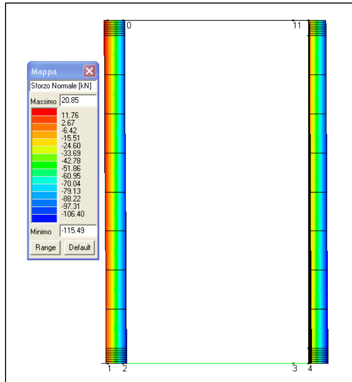
Figura 13-6 Involuppo azione assiale SLU nei piedritti
