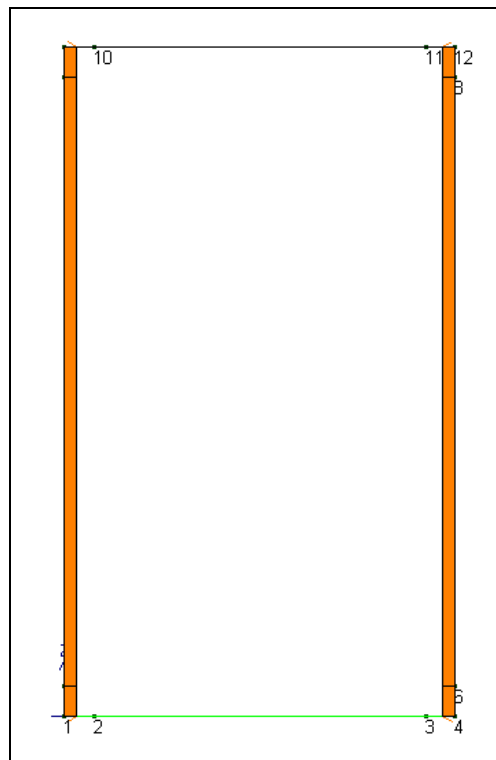
Figura 5-10 Carico veicoli tandem e 9 kN/m 2 a tergo del piedritto sx e dx
