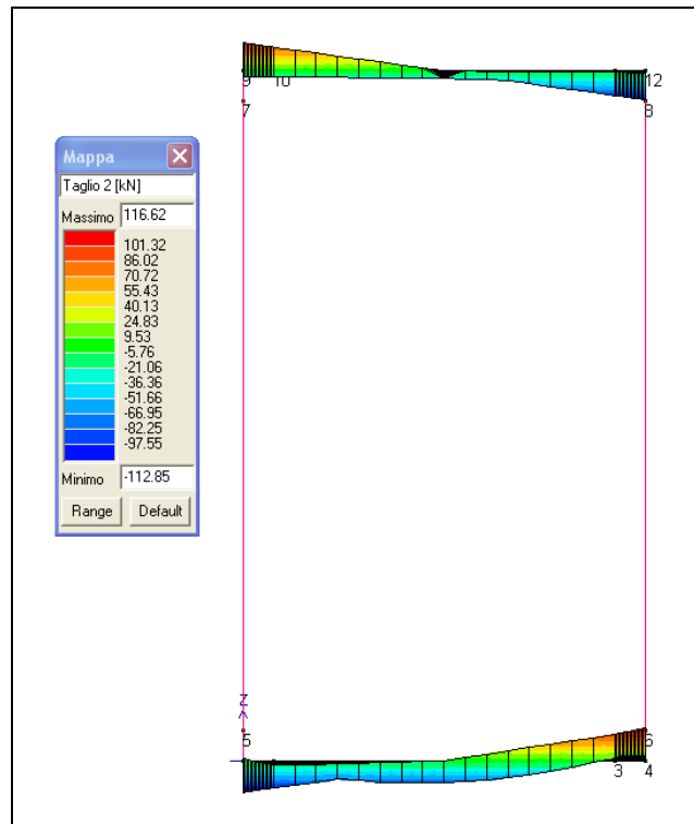
Figura 13-3 Involuppo azione tagliante SLU nelle solette
