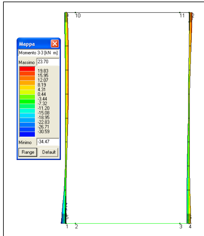
Figura 13-2 Involuppo momento flettente SLU nei piedritti
