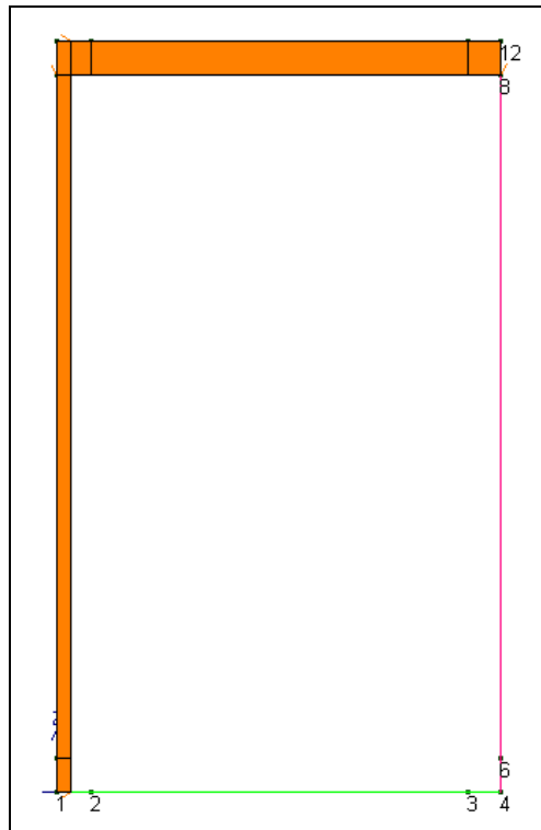
Figura 5-11 Carico veicoli tandem e 9 kN/m 2 a tergo del piedritto sx e centrato
