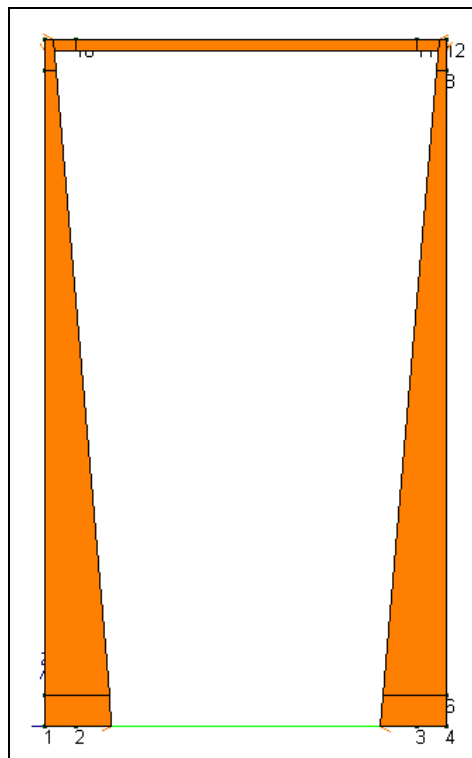
Figura 5-2 Carico permanente portato (rilevato e carreggiata stradale)
