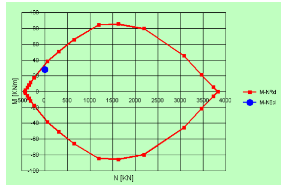
Figura 10-15 SLU pressoflessione piedritto
