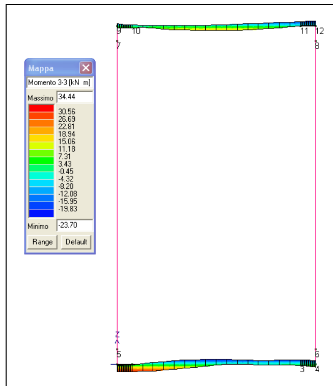
Figura 13-1 Involuppo momento flettente SLU nelle solette
