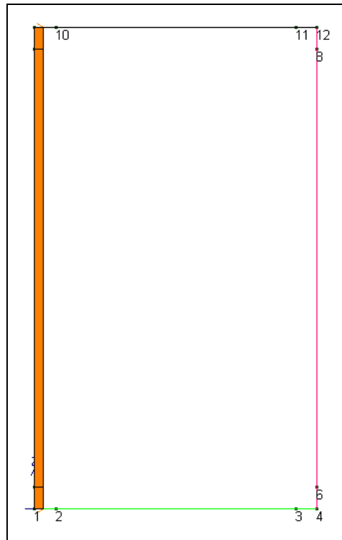
Figura 5-8 Carico veicoli tandem e 9 kN/m 2 a tergo del piedritto sx
