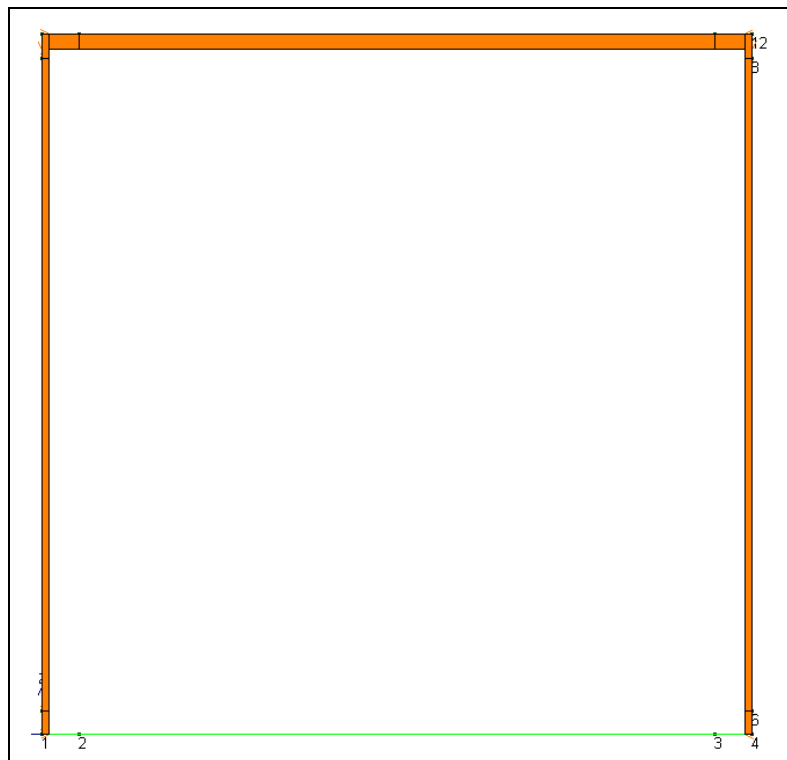
Figura 5-12 Carico veicoli tandem e 9 \text{ kN/m}^2 indefinito
