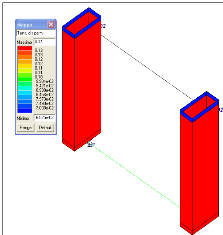
Figura 10-22 Verifica delle tensioni cls in esercizio (permanente)
