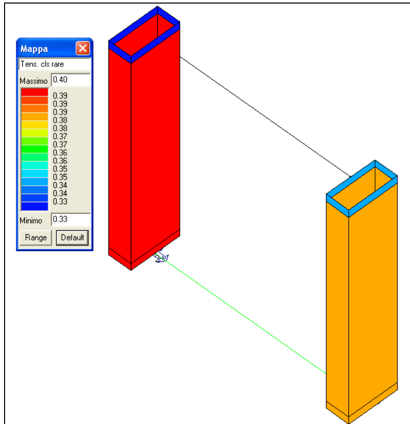
Figura 10-20 Verifica delle tensioni cls in esercizio (rara)
