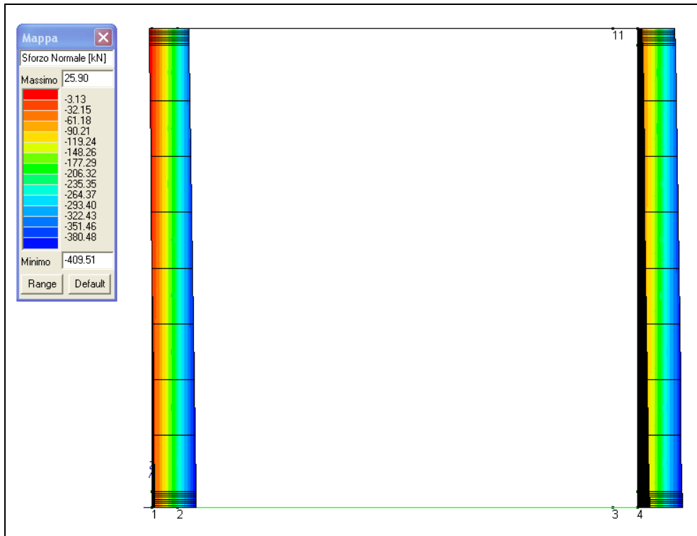
Figura 13-6 Involuppo azione assiale SLU nei piedritti
