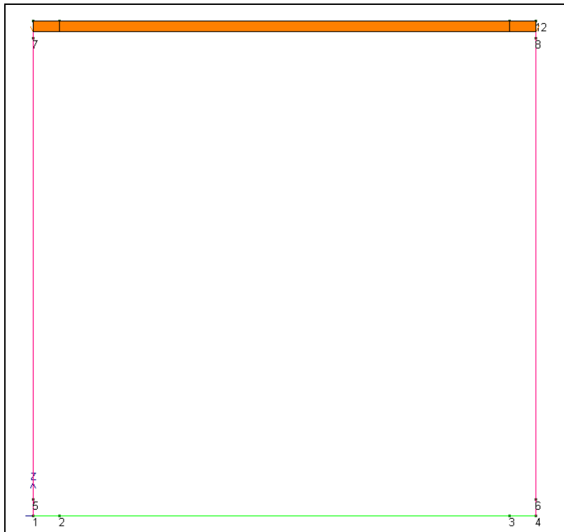
Figura 5-9 Carico veicoli tandem e 9 \text{ kN/m}^2 centrato
