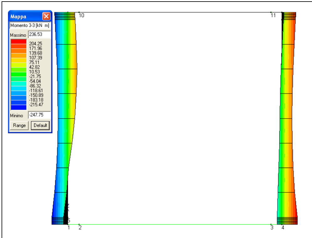
Figura 13-2 Involuppo momento flettente SLU nei pedritti
