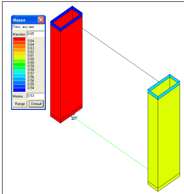
Figura 10-21 Verifica delle tensioni acciaio in esercizio (rara)
