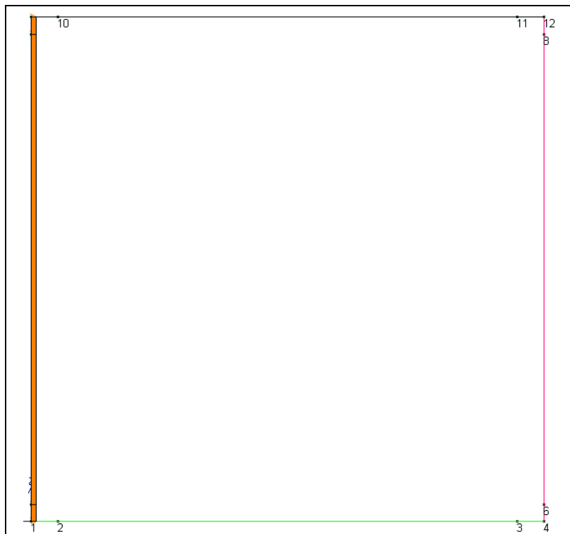
Figura 5-8 Carico veicoli tandem e 9 kN/m 2 a tergo del piedritto sx
