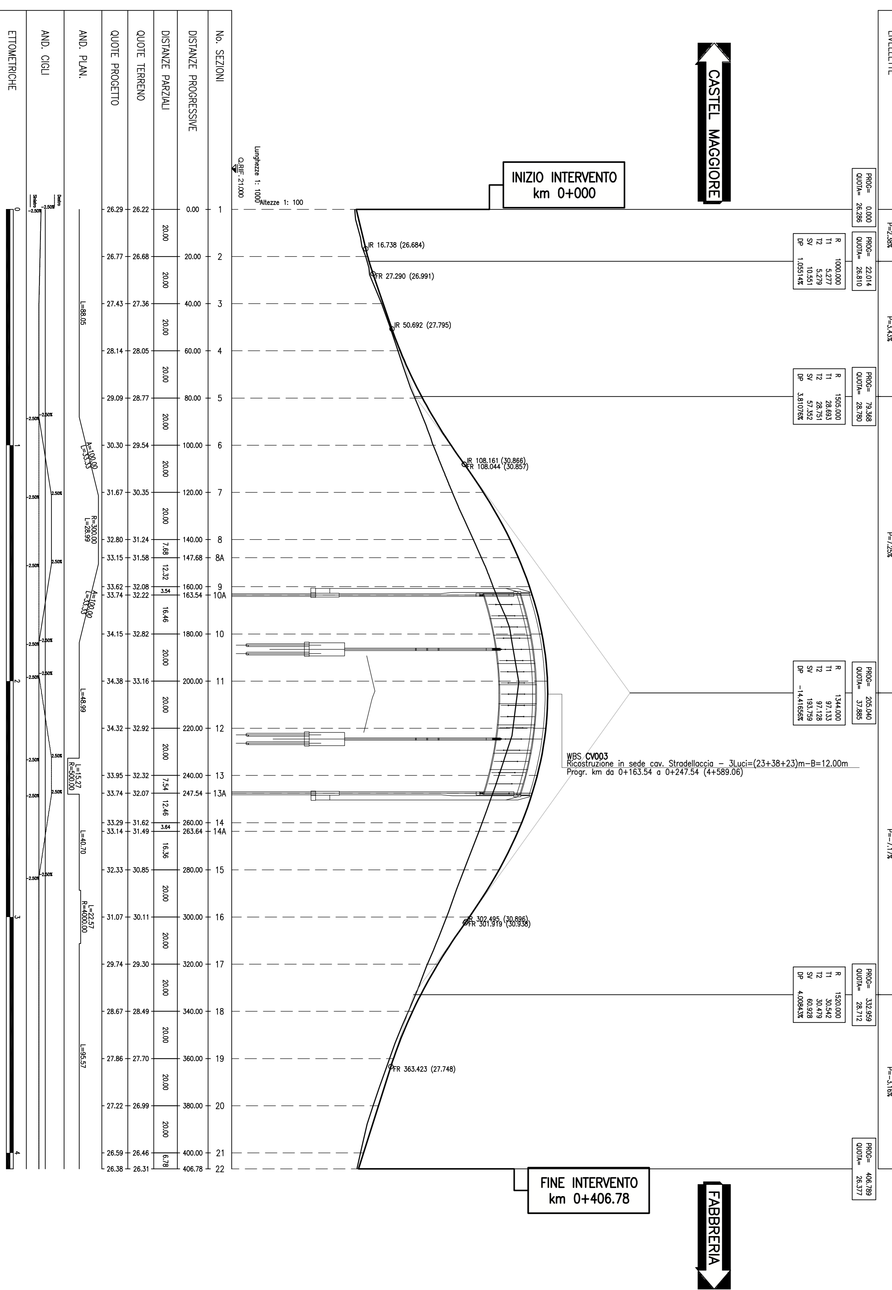
PROFLO LONGITUDINALE – scala 1:1000/100
