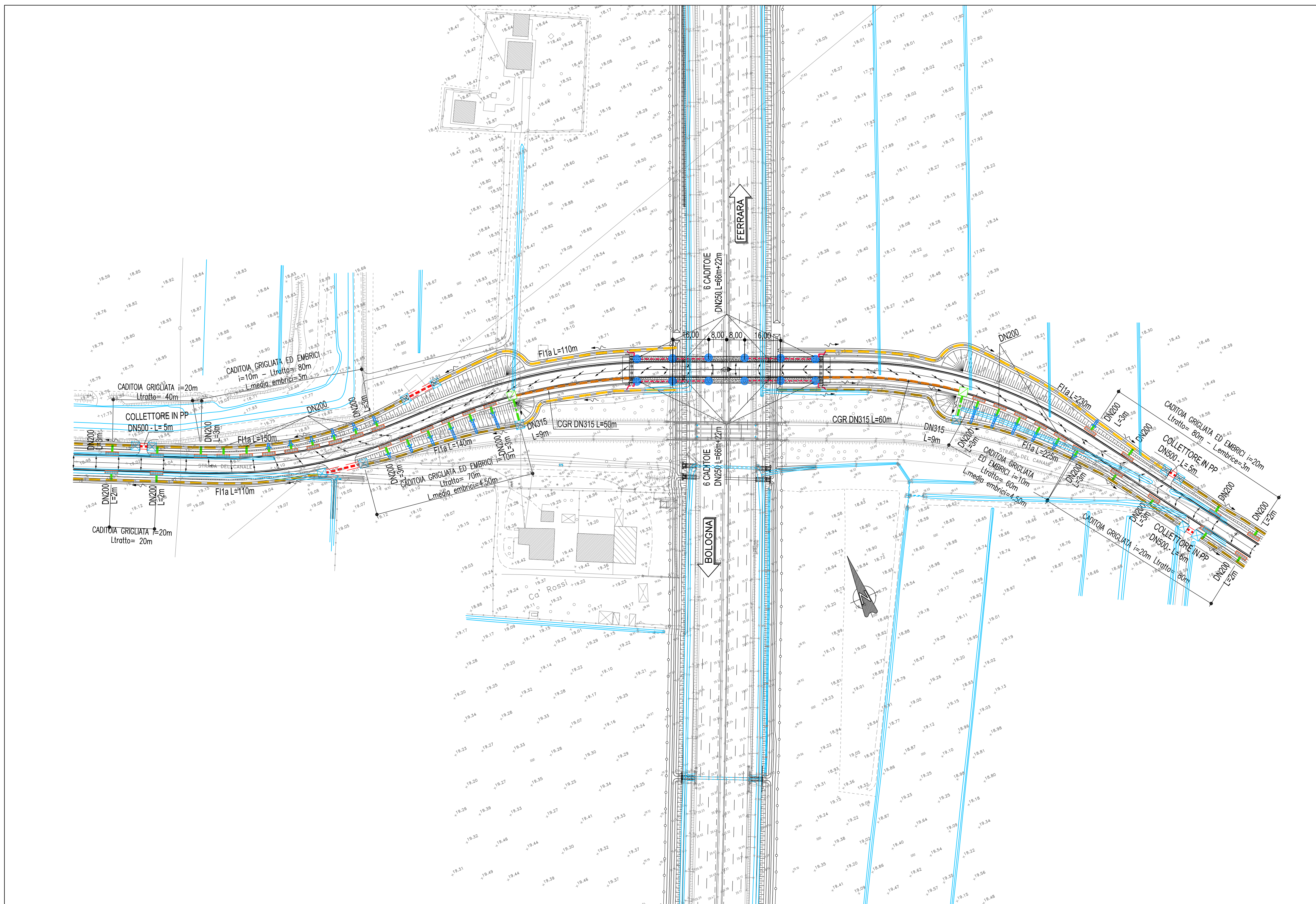
PLANIMETRIA IDRAULICA - scala 1:1000
