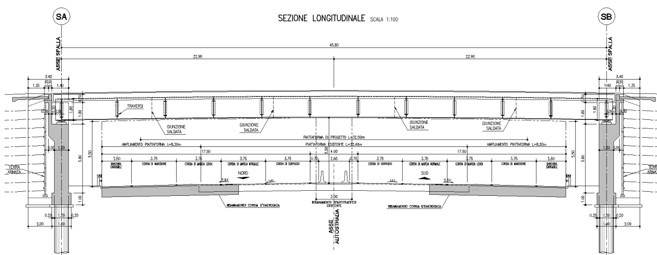
Profilo longitudinale.
