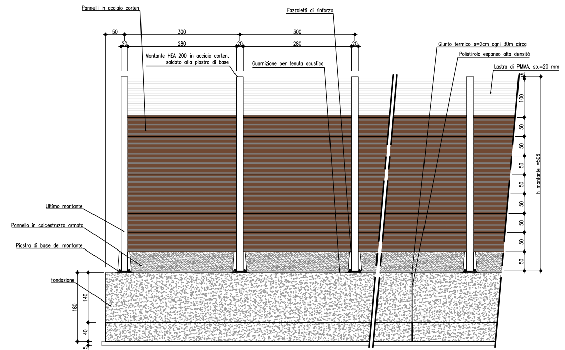
BARRIERA H=5.00m LATO RICETTORE
