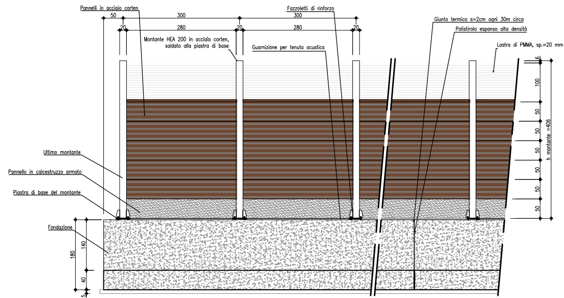
BARRIERA H=4.00m LATO RICETTORE
