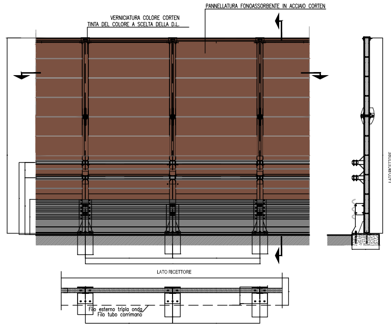
BARRIERA INTEGRATA H=5.00m LATO STRADA
