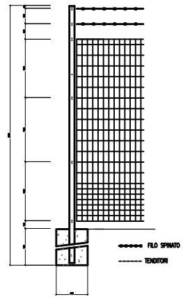
PARTICOLARE RECINZIONE METALLICA - SCALA 1:20 misure in mm.
