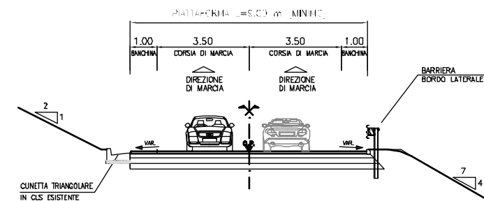
SEZIONE TIPO RAMPA DI SVINCOLO ESISTENTE MONODIREZIONALE A 2 CORSIE
