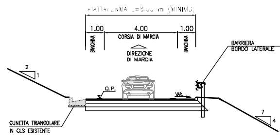
SEZIONE TIPO RAMPA DI SVINCOLO ESISTENTE MONODIREZIONALE
