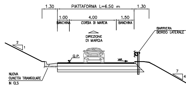
SEZIONE TIPO NUOVA RAMPA DI SVINCOLO MONODIREZIONALE *
