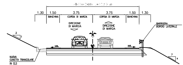
SEZIONE TIPO NUOVA RAMPA DI SVINCOLO BIDIREZIONALE *
