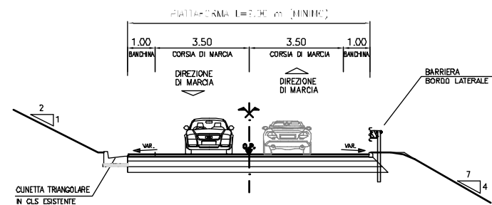
SEZIONE TIPO RAMPA DI SVINCOLO ESISTENTE BIDIREZIONALE
