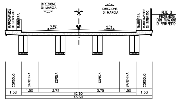
SEZIONE TIPO NUOVA RAMPA BIDIREZIONALE SU OPERA (Cavalcavia)
