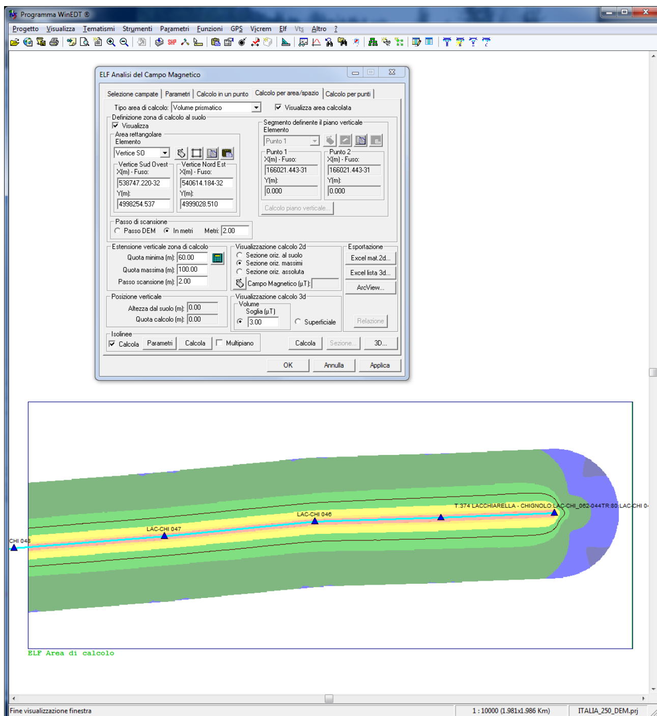
Figura 3 - Impostazione e risultati del calcolo tridimensionale
