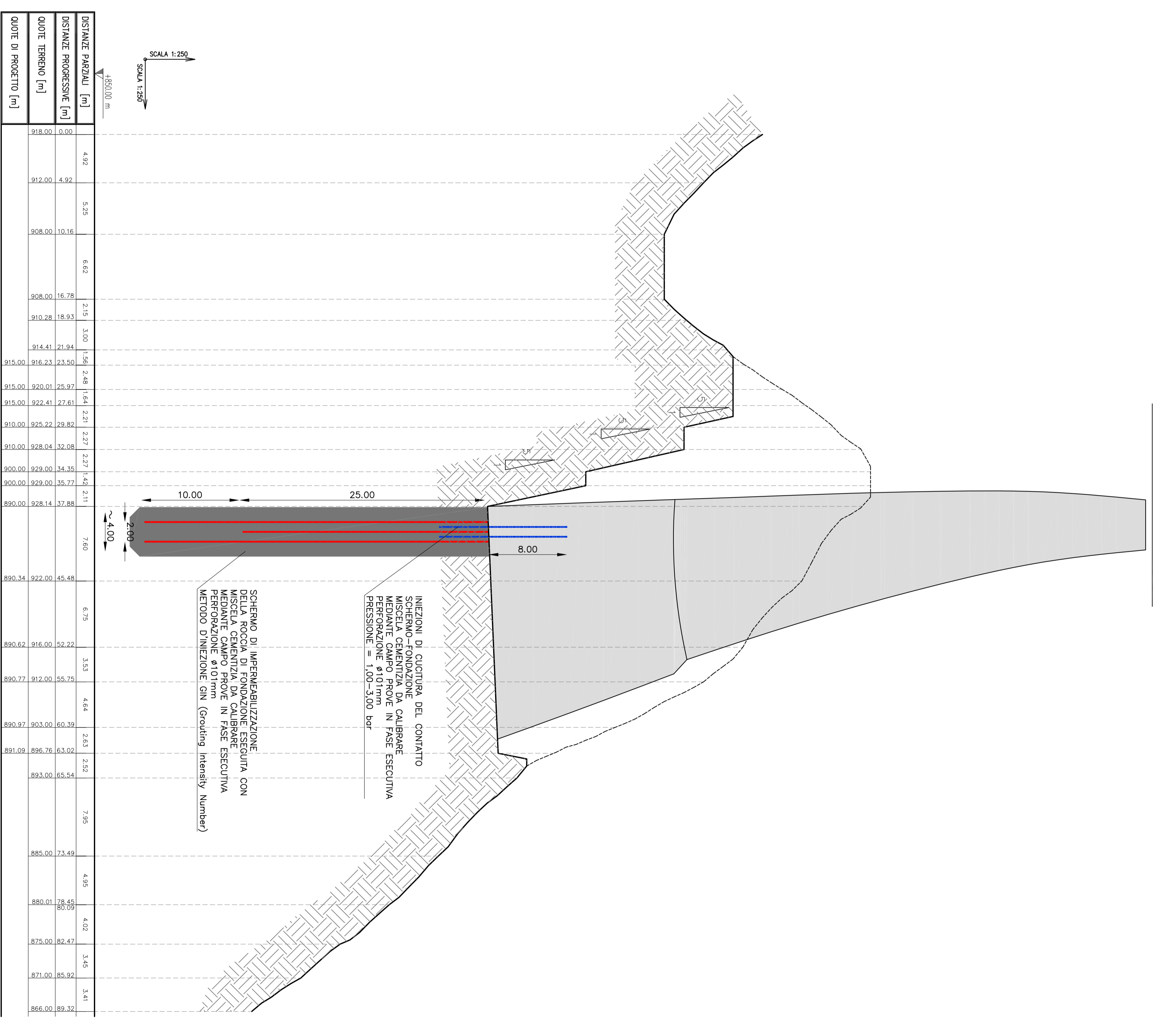
SEZIONE VERTICALE TIPOLOGICA INIEZIONI scala 1:250
