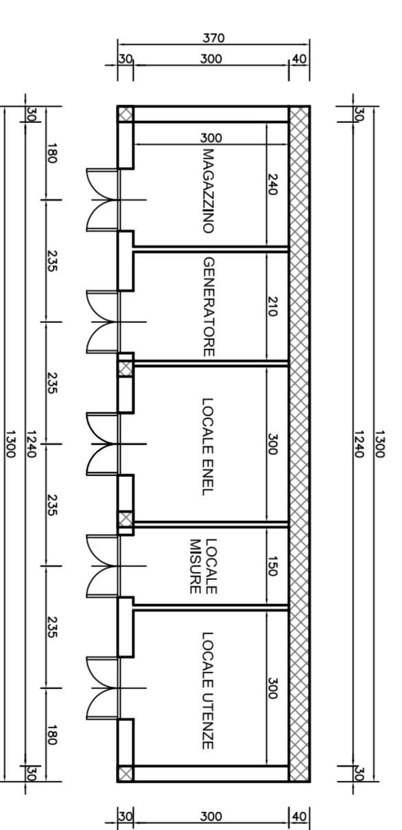
EDIFICIO SECONDARIO PIANTA PIANO TERRA Scala 1:100
