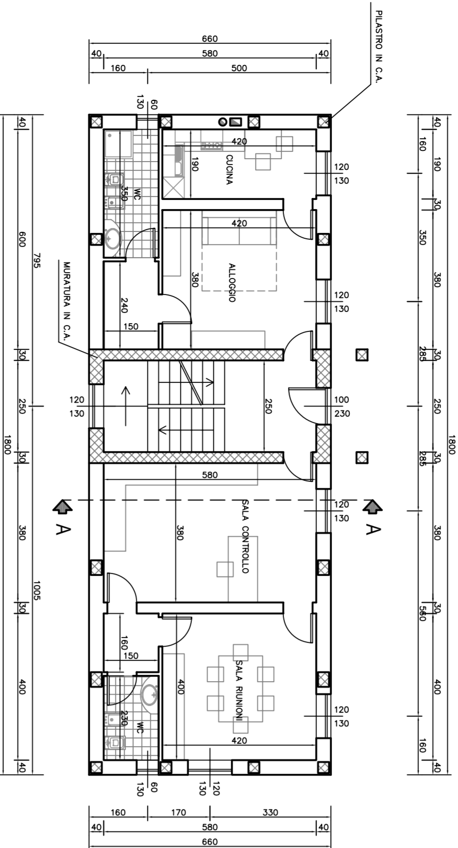
EDIFICIO PRINCIPALE PIANTA PIANO TERRA Scala 1:100
