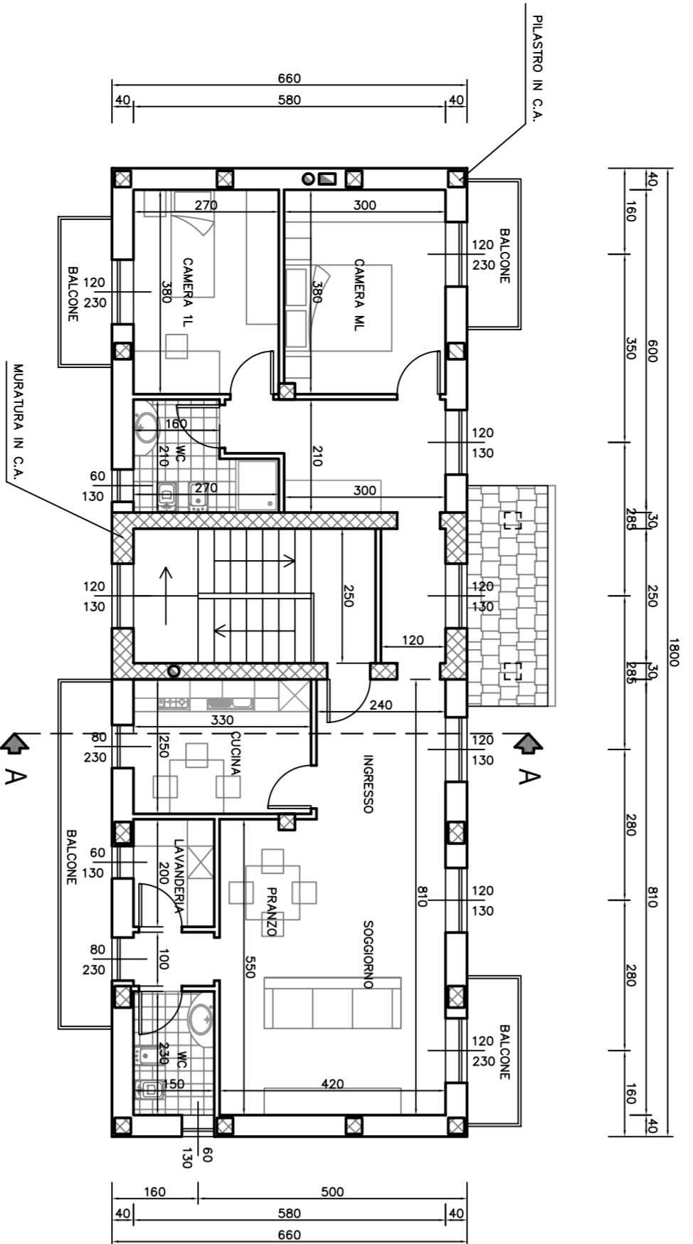
EDIFICIO PRINCIPALE PIANTA PIANO PRIMO Scala 1:100
