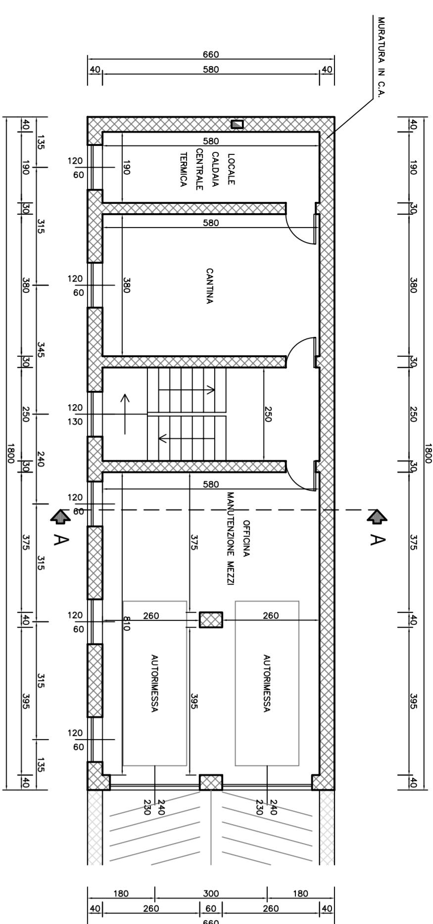
EDIFICIO PRINCIPALE PIANTA PIANO INTERRATO Scala 1:100
