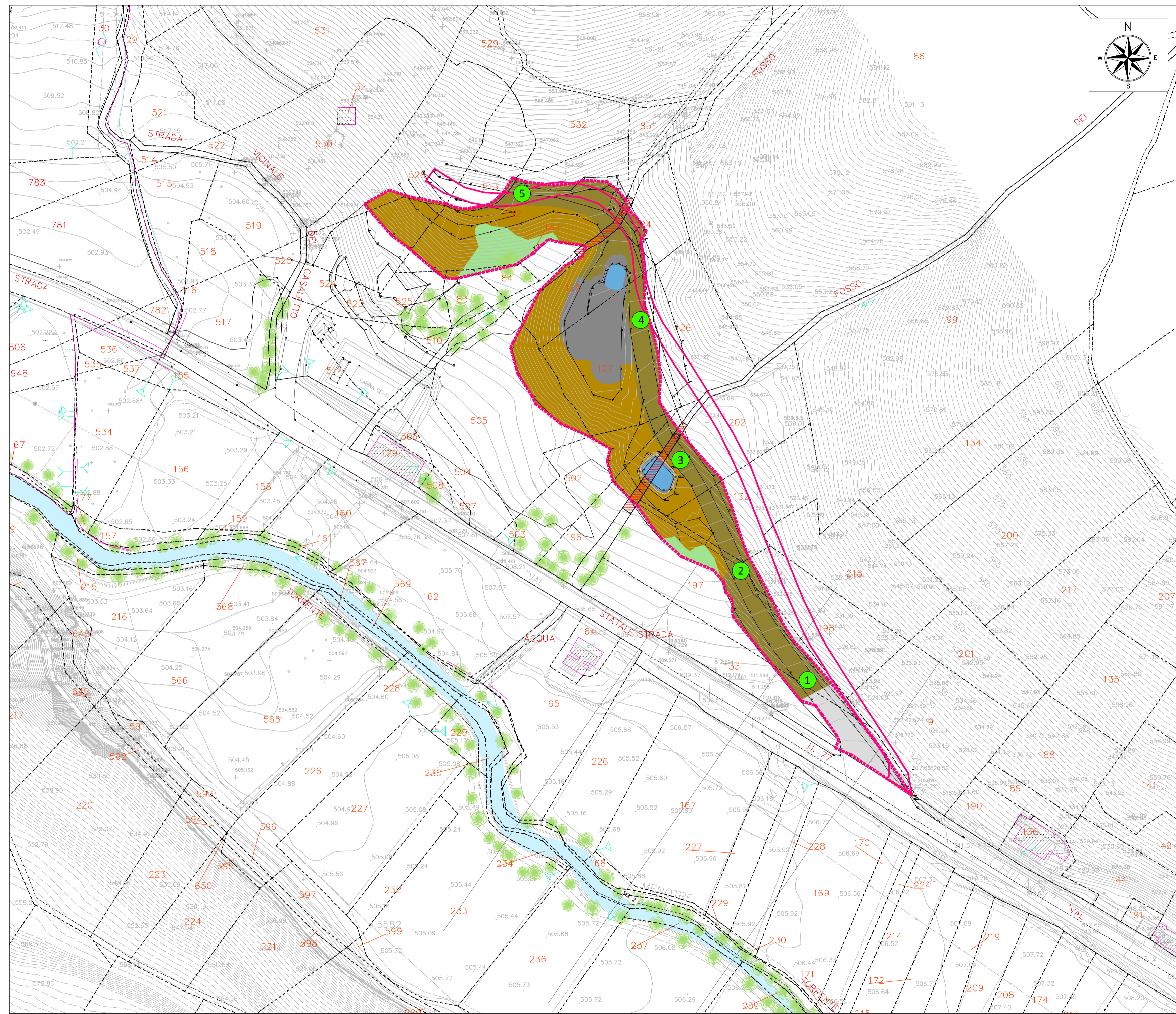
PLANIMETRIA DELLO STATO DI FATTO - SCALA 1:1000
