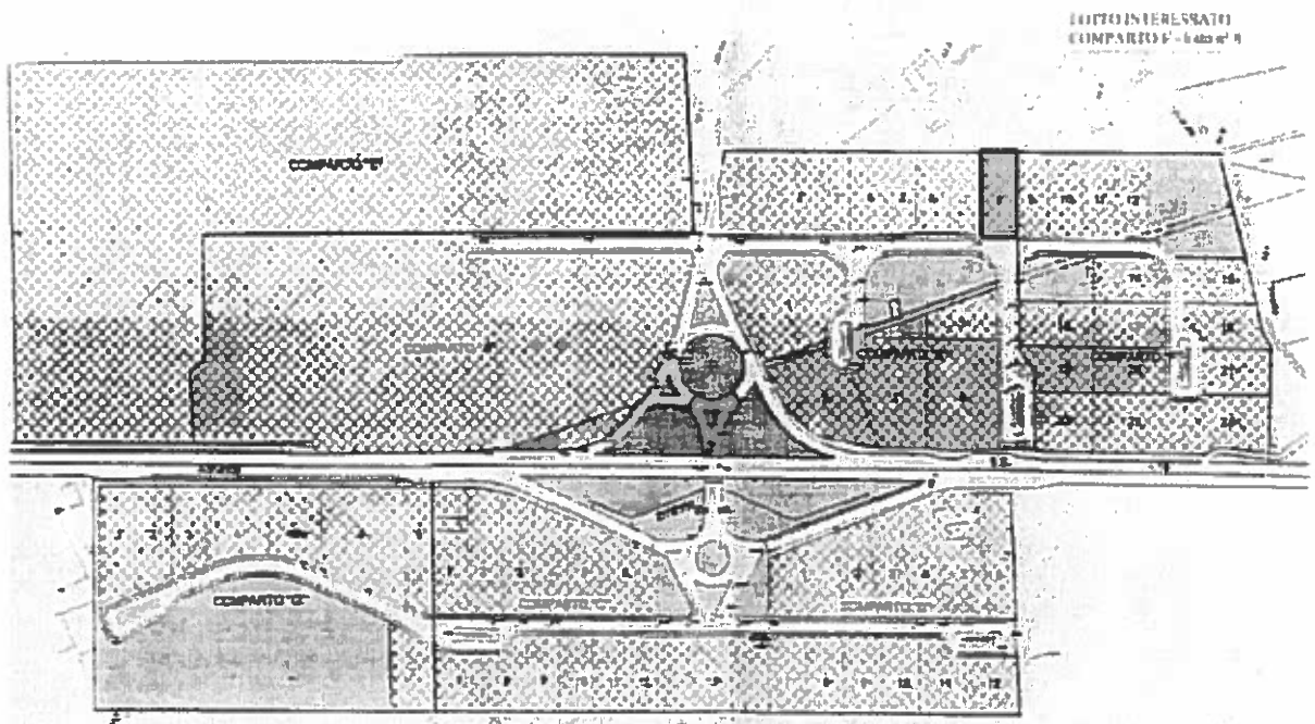
Fig. 4/5 – Zona P.I.P Stralcio comparto F – planimetria di insieme e zoom del comparto F – lotto n. 8
