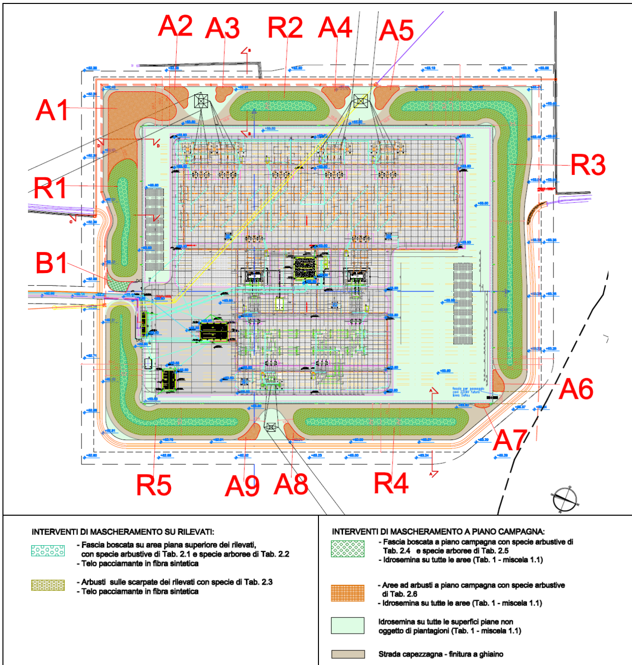
Fig. 3 – Schema planimetrico interventi (agg. Novembre 2016)
