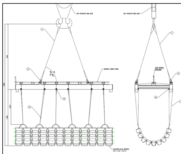
Figura 17 - Materasso in cemento armato e frame d'installazione
