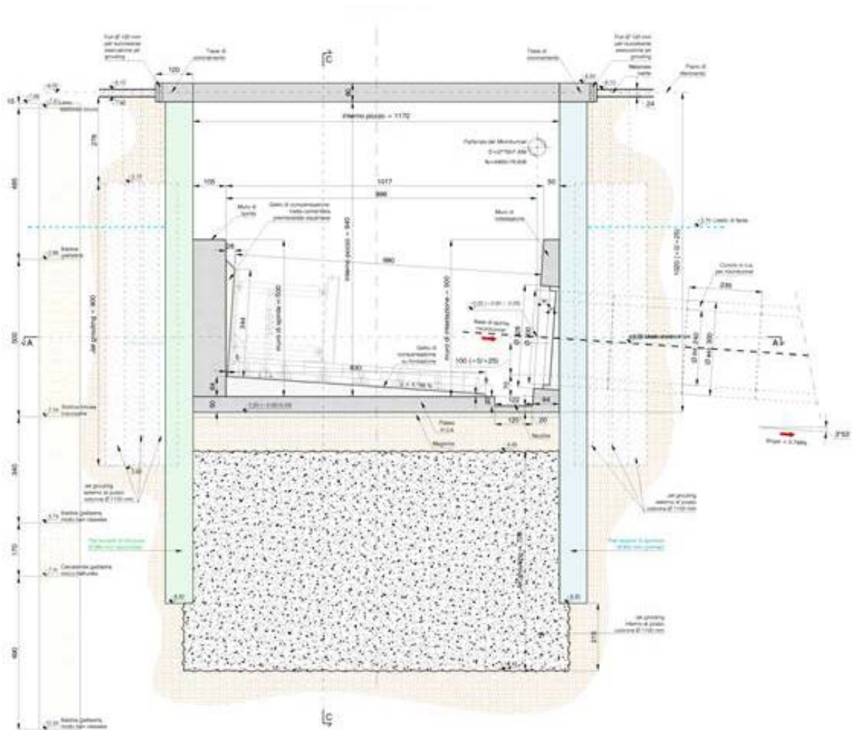
Figura 23 – Configurazione del pozzo di spinta durante la costruzione del microtunnel
