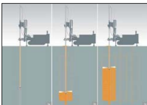
Figura 24 – Schema di costruzione jet-grouting
