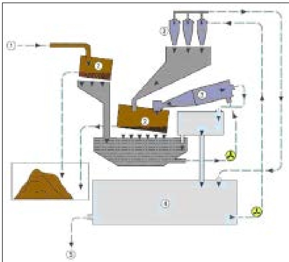
Figura 37 – Principio di funzionamento di un impianto di separazione.
