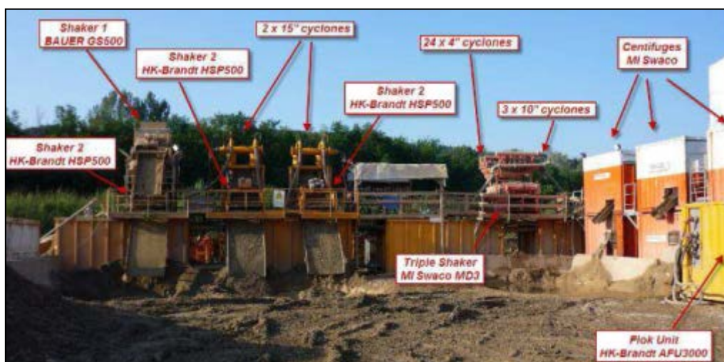
Figura 38 – Tipico impianto automatico di separazione.
