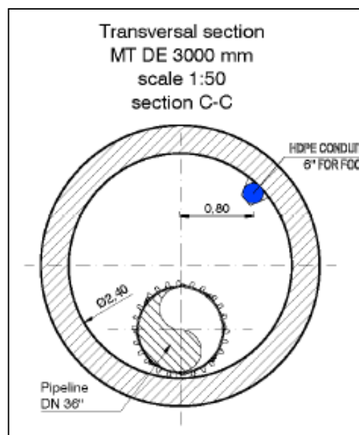
Figura 53 - Sezione trasversale Microtunnel
