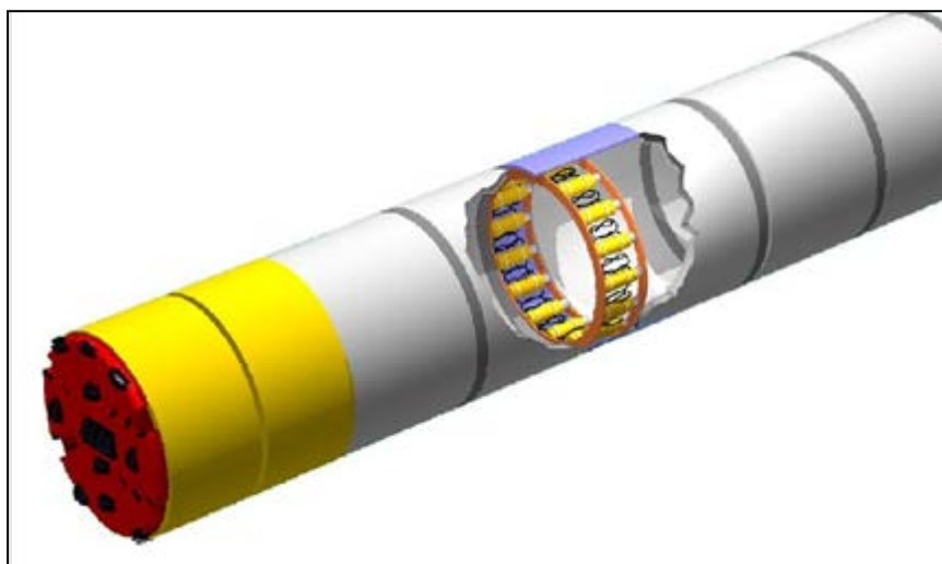
Figura 35 – Installazione degli spingitori intermedi lungo il microtunnel.
