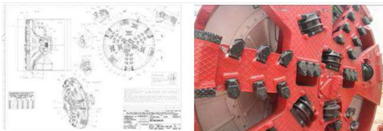
Figura 29 – Tipico testa fresante Mixed Ground per AVN2000D
