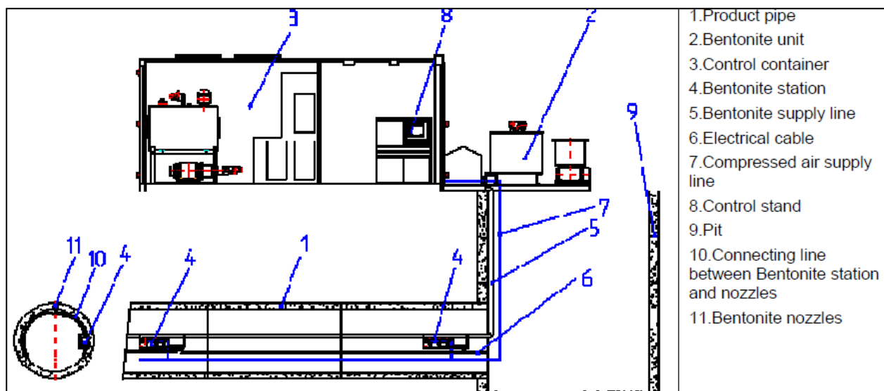
Figura 31 – Tipico schema automatico per l'impianto di lubrificazione
