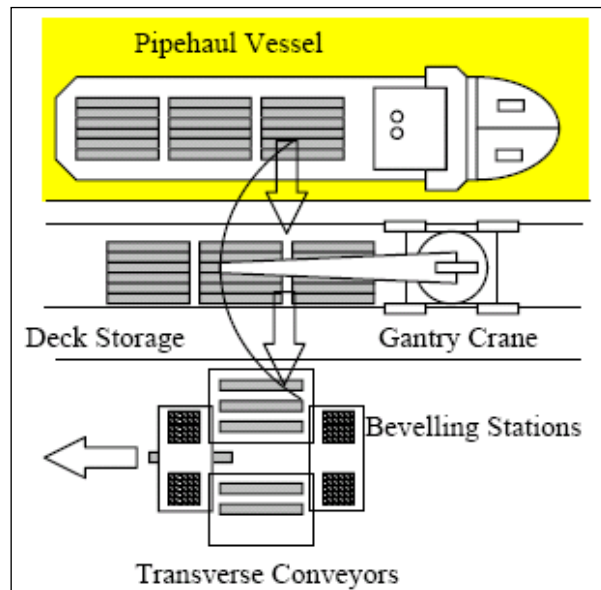
Figura 1 – Movimentazione Tubi sulla Castoro Sei
