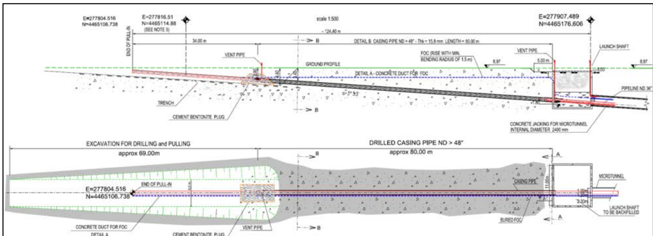
Figura 41 – Installazione del tubo di protezione da 48” a terra
