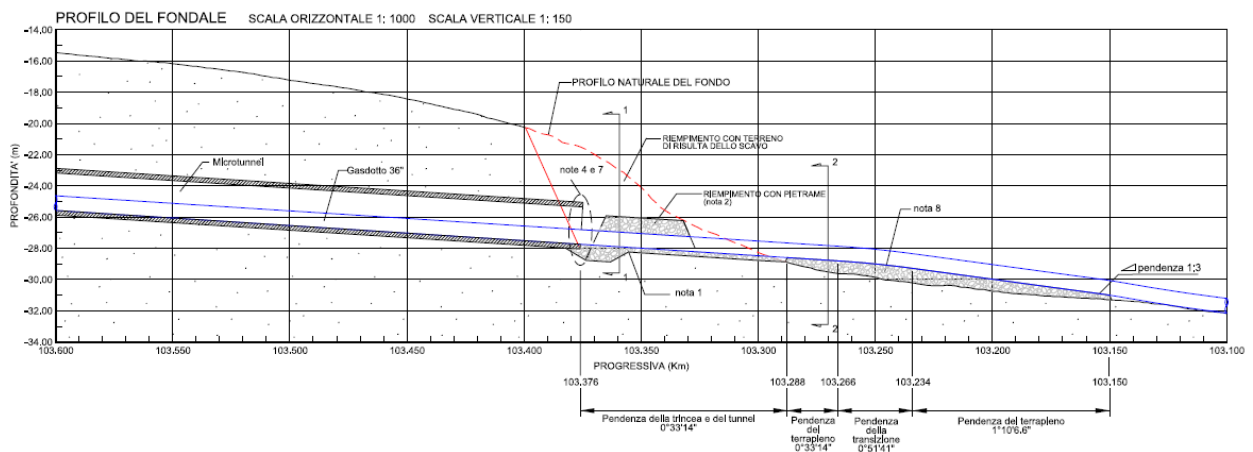
Figura 46 - Lavori all'uscita offshore del microtunnel
