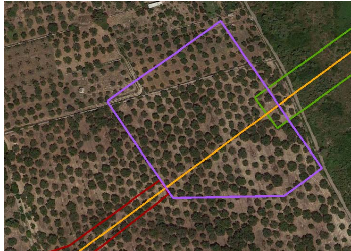
Figura 22– Area di lavoro complessiva del microtunnel e strada di accesso lungo la RoW
