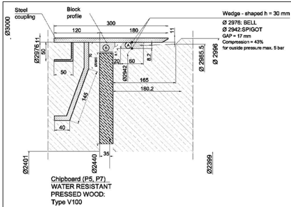
Figura 39 – Tipico giunto di un concio
