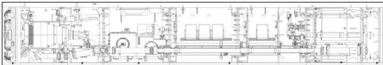
Figura 28 – Tipico schema di dettaglio di una Herrenknecht AVN2000 TBM
