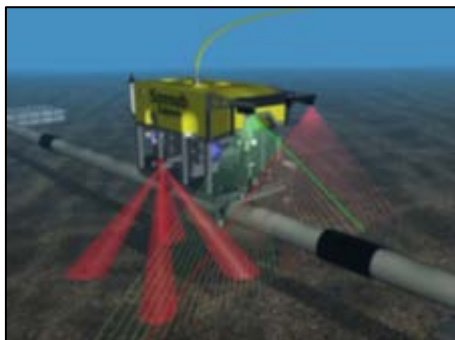
Figura 19 - Indagine As-Laid con WROV
