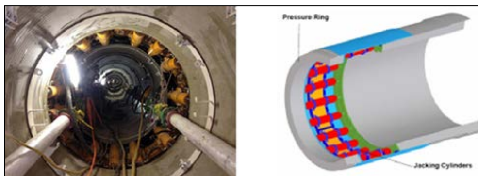
Figura 36 – Installazione di un stazione intermedia di spinta lungo il microtunnel
