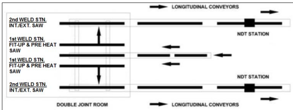
Figura 6- Area di Doppio Giunto
