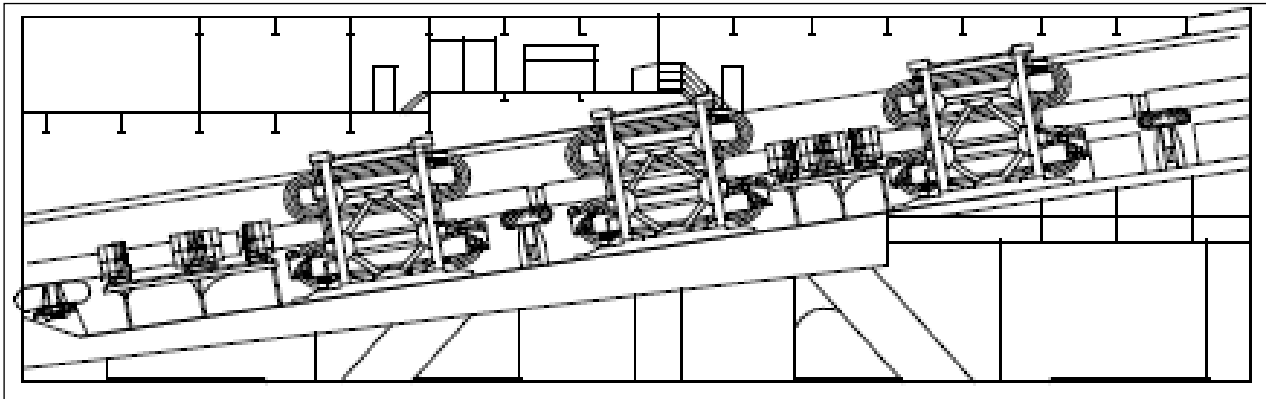
Figura 9 – Tensionatori nella linea di varo da 130 Te ognuno
