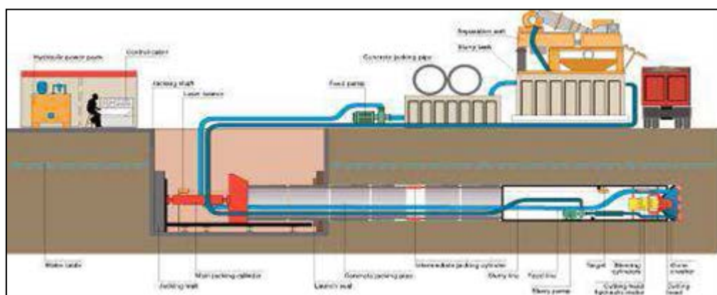
Figura 27 – Schema tipico di lavoro del microtunnel
