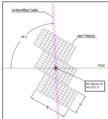
Figura 18 - Posizionamento dei materassi
