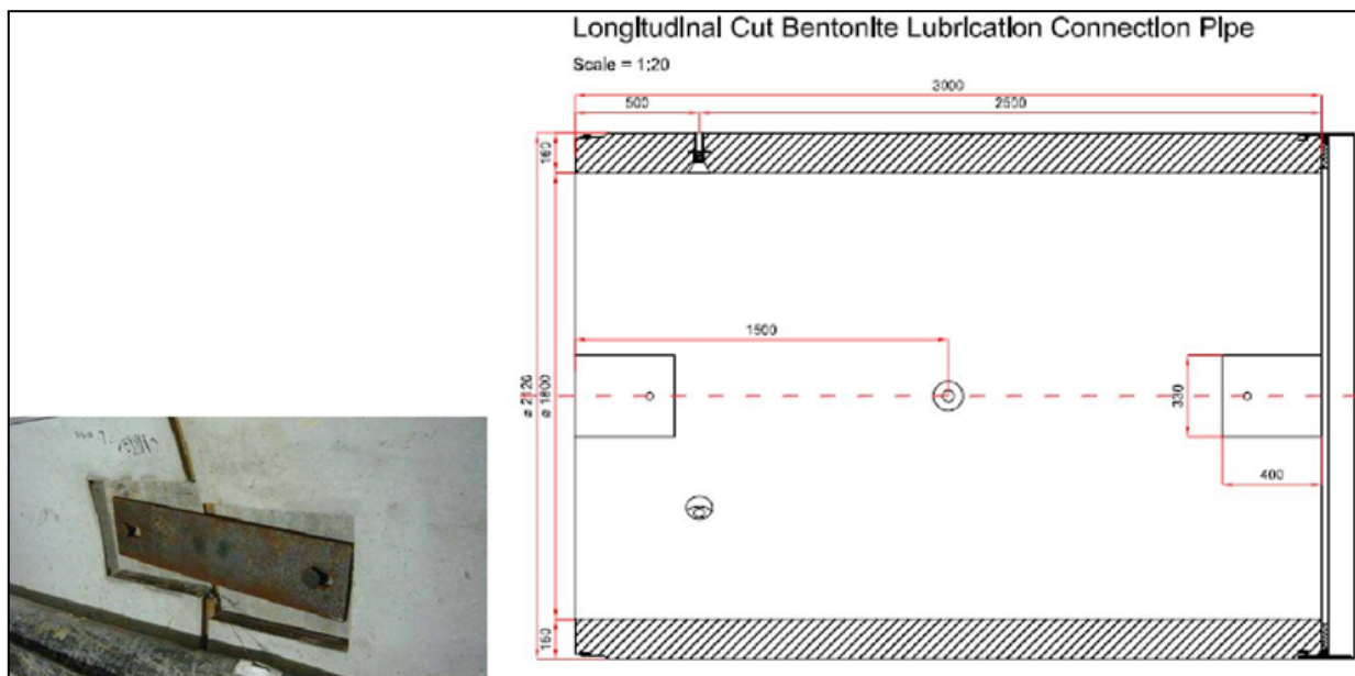
Figura 40 – Esempio di giunto di connessione e di concio di lubrificazione
