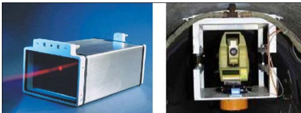
Figura 32 – Laser target ELS (sinistra) e strumento di monitoraggio, TCA montato nel tunnel (destra)
