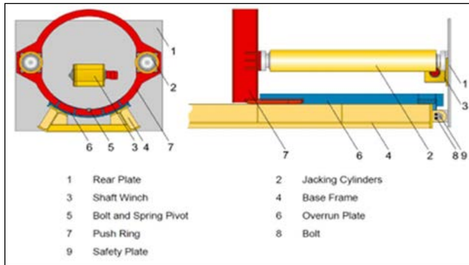
Figura 34 – Spingitore Principale e Cilindri telescopici Idraulici
