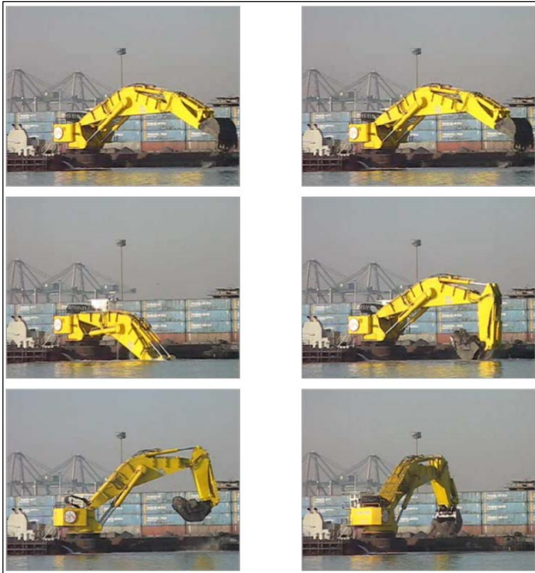
Figura 45 – Draga escavatrice al lavoro
