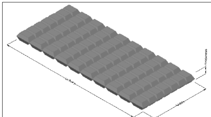
Figura 4 - Tipico materasso per l'attraversamento
