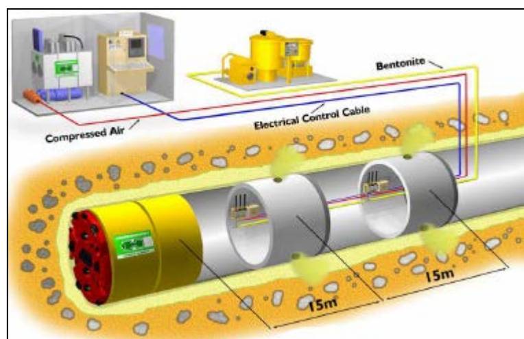
Figura 30 – Tipico Sistema Automatico di Lubrificazione
