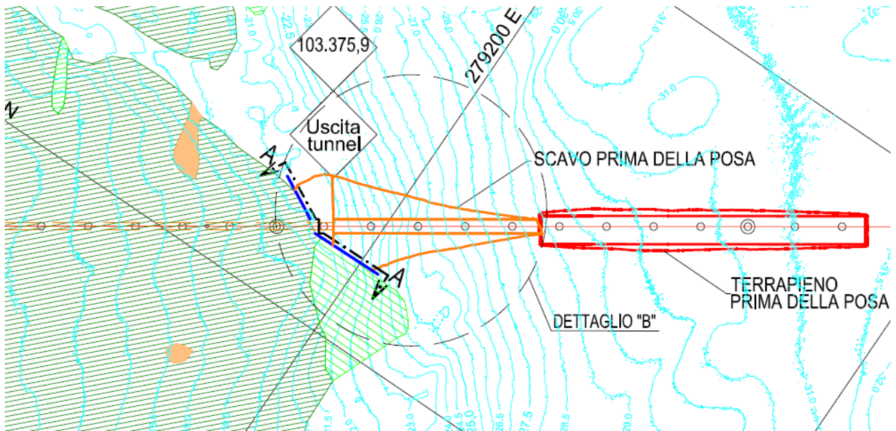
Figura 25 – Configurazione della trincea di uscita
