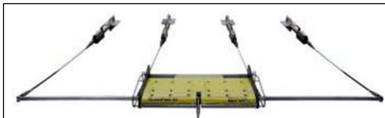
Figura 16 - EIVA ROTV "Scanfish Katria" con 4 magnetometri
