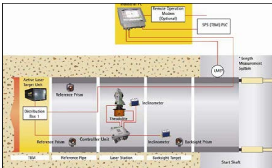
Figura 33 – Sistema di guida SLS-LT visione generale
