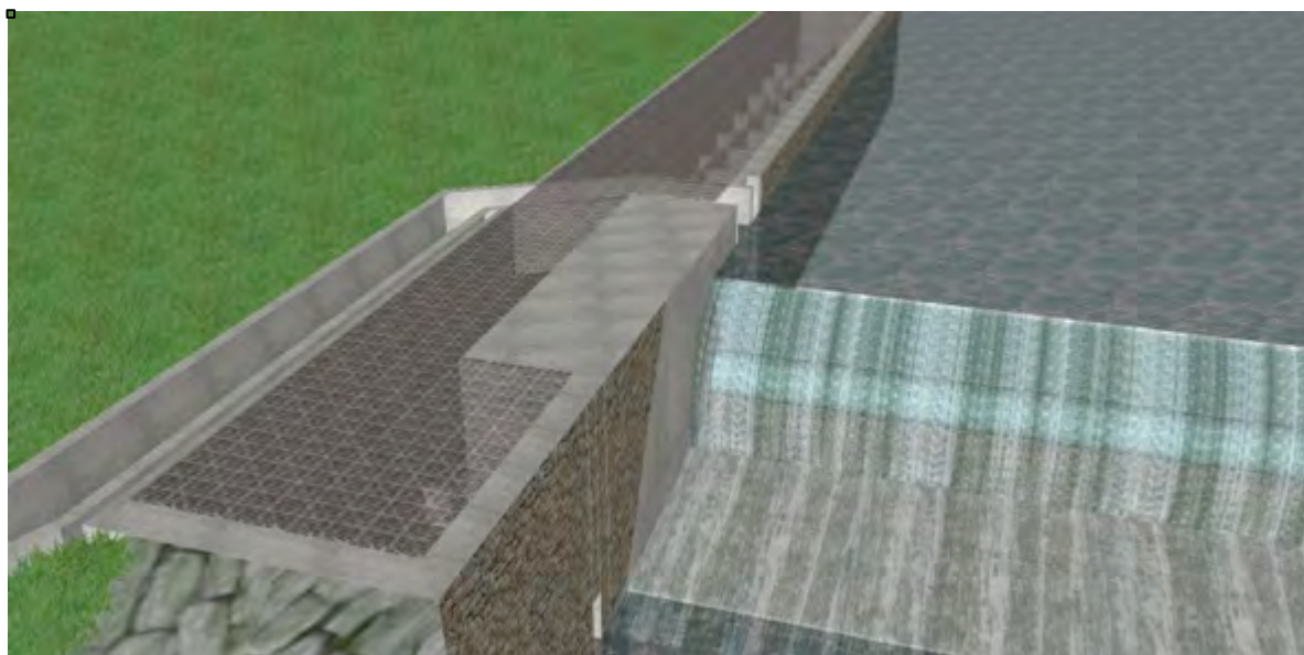
La scala di risalita posta in destra orografica
