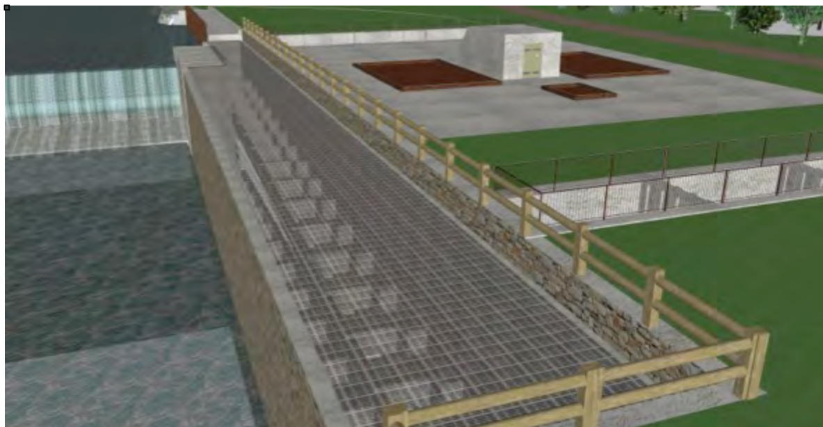
La scala di risalita posta in sinistra orografica
