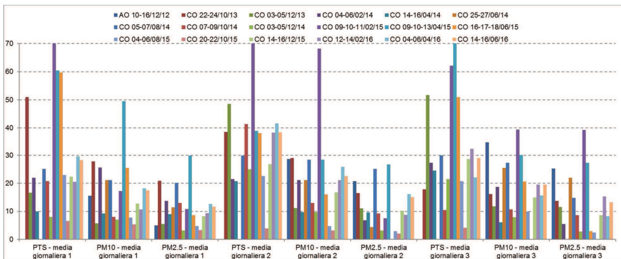
Figura 9 - Monitoraggio Atmosfera Cantieri fissi ATC 01 / Svincolo Lanzo. Dettaglio misurazioni PM 10, PM 2,5, PTS.
