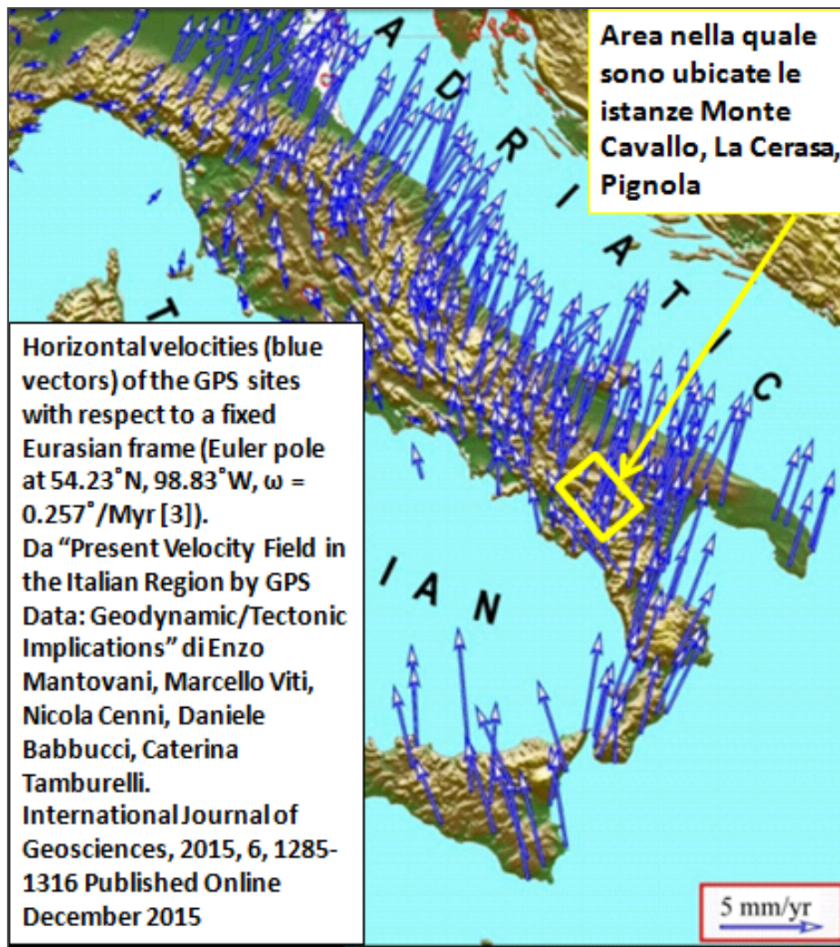
Figura 7: evidenze della tettonica crostale che determina lo spostamento lento e continuo dell'Appennino verso il Mare Adriatico interessando in maniera differenziata, in relazione alle caratteristiche litologiche, anche il sottosuolo nel quale sono state realizzate le perforazioni petrolifere provocando numerosi breakouts nelle perforazioni. E' evidente che la tettonica crostale citata interessa anche il sottosuolo che ricade nelle istanze Monte Cavallo, La Cerasa e Pignola.
