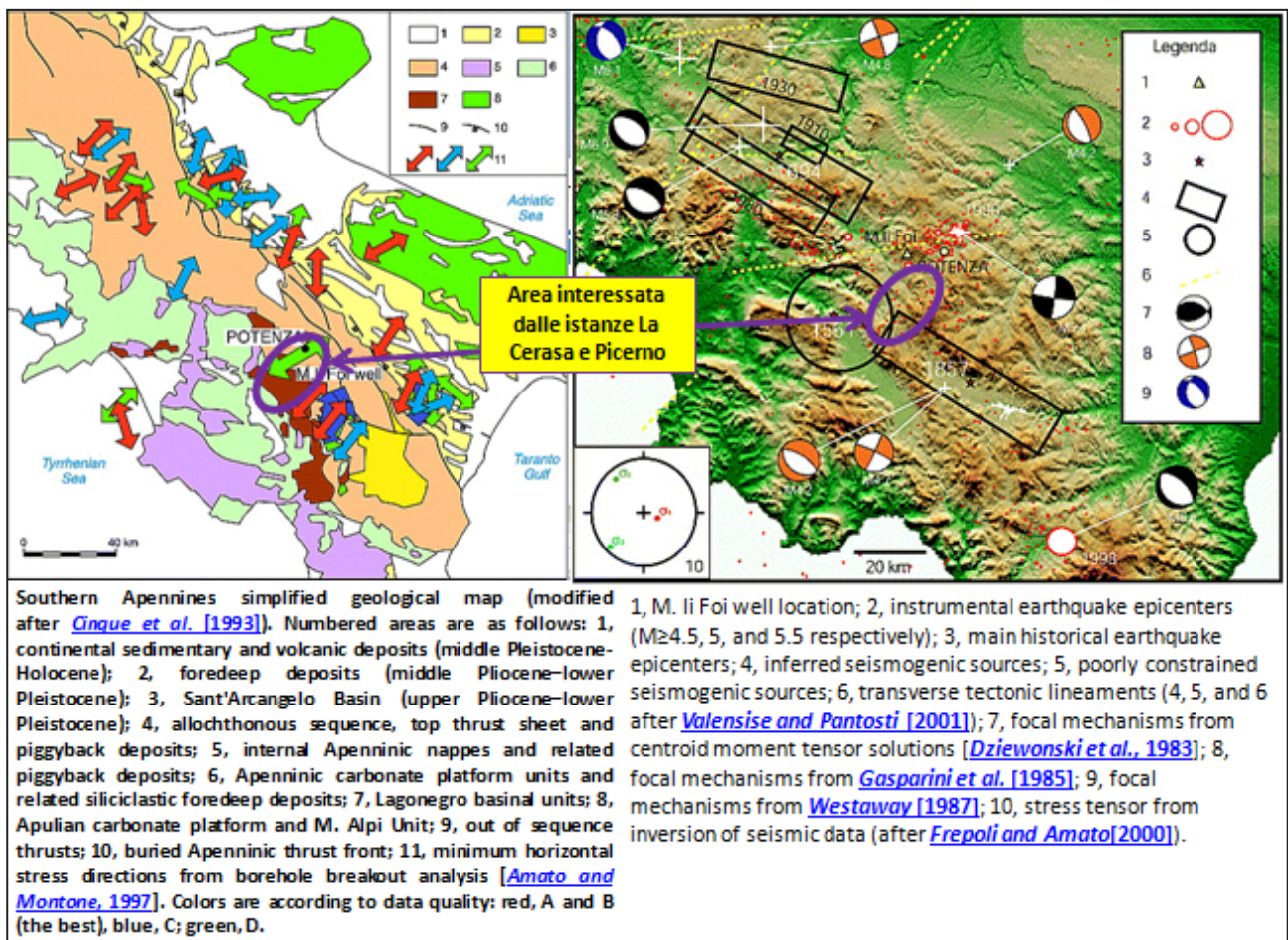
Figura 5 : Figure tratte da: Along-depth stress rotations and active faults: An example in a 5-km deep well of southern Italy; di Maria Teresa Mariucci, Alessandro Amato, Roberto Gambini, Maurizio Giorgioni, Paola Montone, pubblicata su Tectonics, vol. 21, Issue 4, august 2002, pages 3-1 - 3-9. Come si vede le aree interessate dalle istanze Lça Cerasa e
