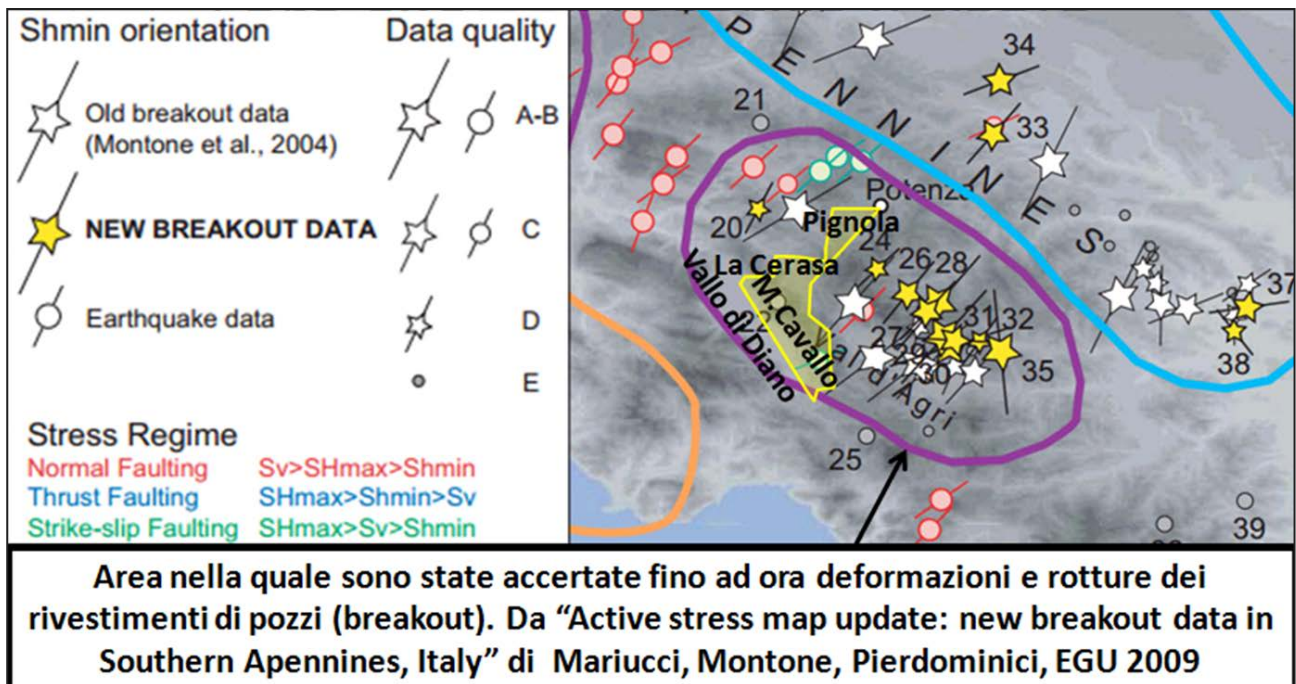
Figura 6: l'immagine evidenzia le deformazioni (breakouts) registrate nelle perforazioni in Basilicata già note (stelle bianche) e pubblicate da Montone et al. 2004 e nuove (stelle gialle). Come si vede l'istanza La Cerasa si trova nella fascia appenninica tipicamente caratterizzata dai fenomeni di breakouts.
