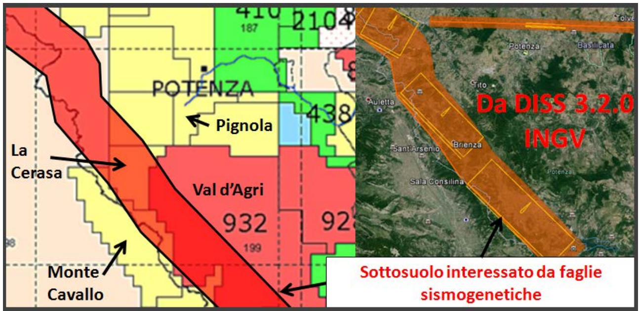
Figura 4: le faglie sismogenetiche che interessano il sottosuolo delle istanze Monte Cavallo e La Cerasa secondo DISS 3.2.0 di INGV. I riquadri con linea gialla nella immagine a destra individuano faglie sismogenetiche individuali che hanno originato i terremoti del 1561 (riquadro in alto nell'immagine a destra) e 1857 ( riquadri al centro e a sinistra, nell'immagine a destra, che interessano l'istanza La Cerasa ).
