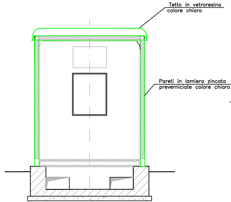
SEZIONE W-W
