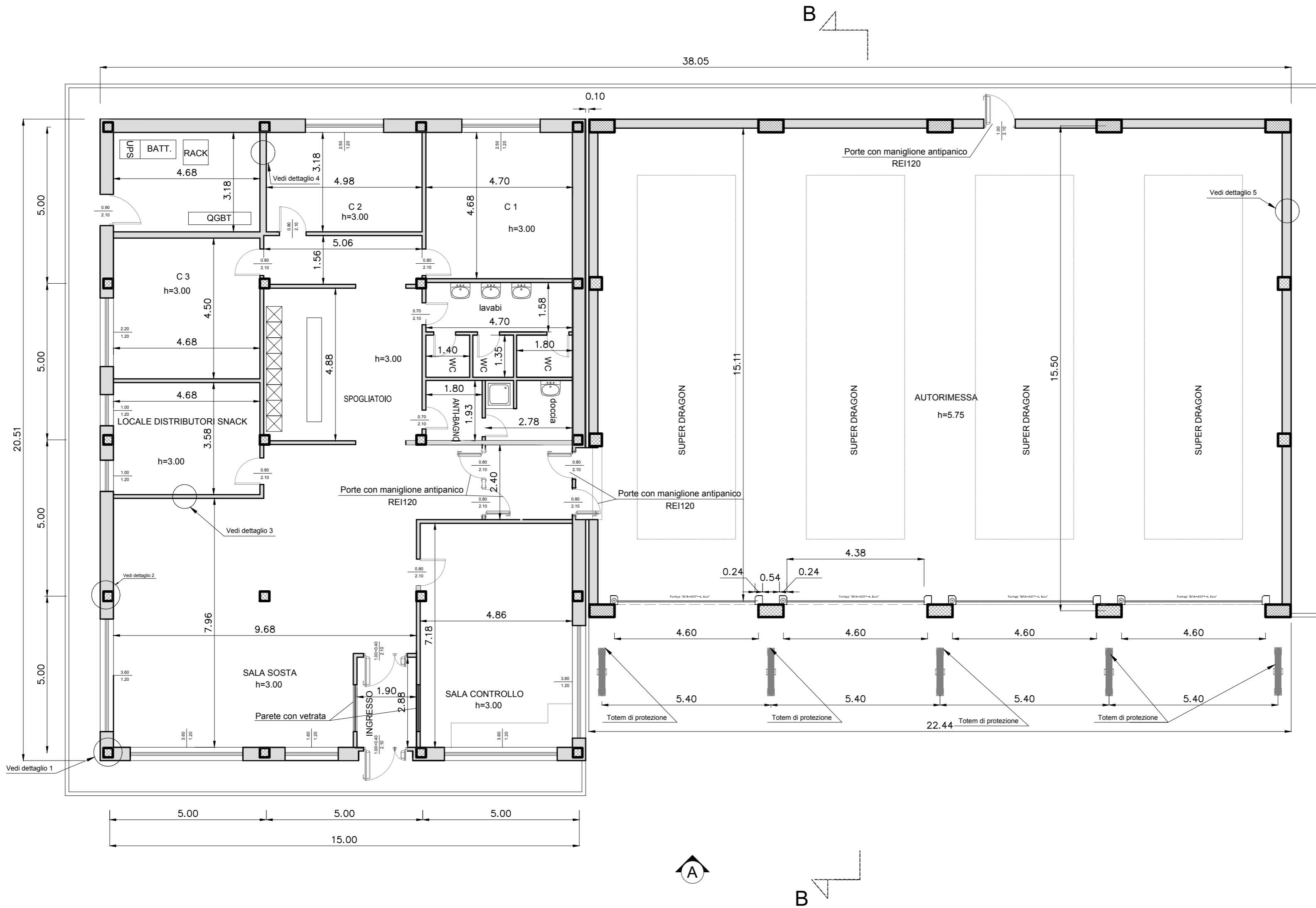
PIANTA Scala 1:100
