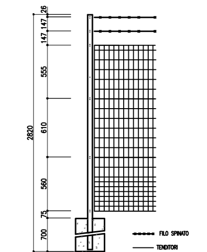
PARTICOLARE RECINZIONE METALLICA Scala 1:40 misure in mm
