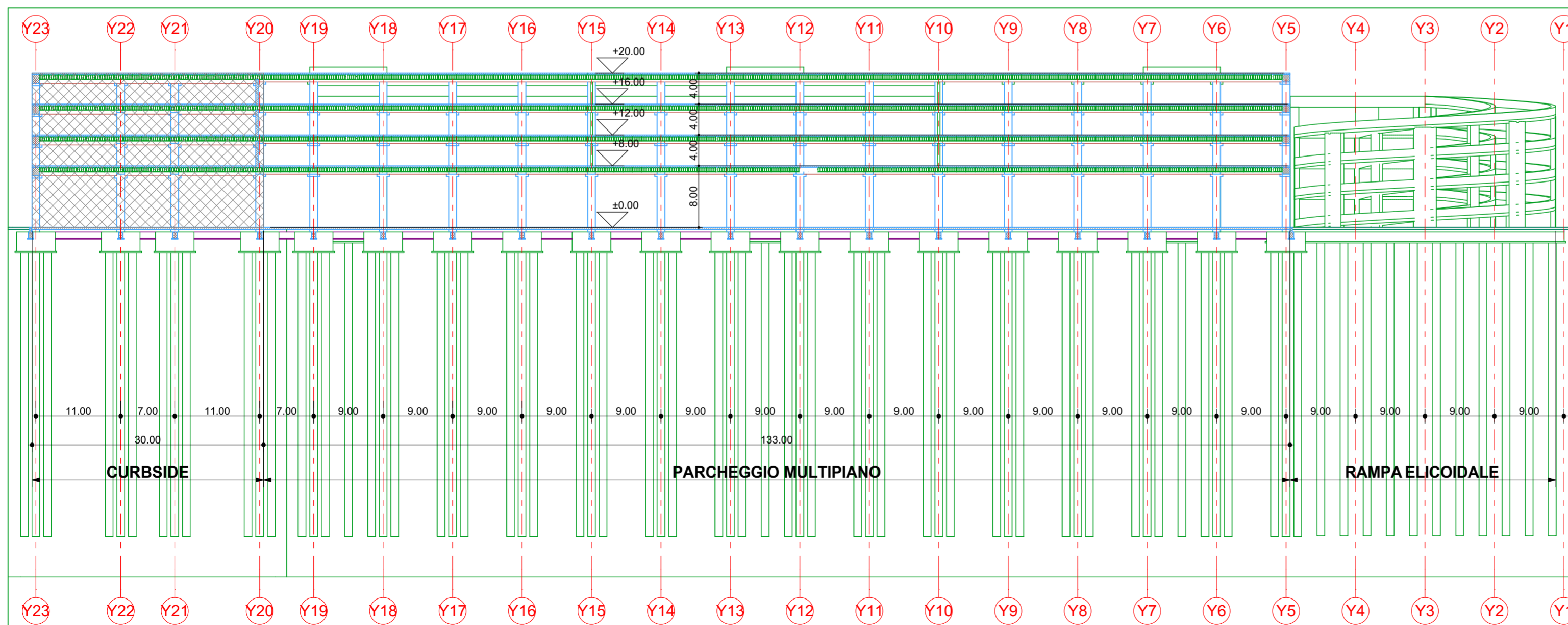
Sezione Edificio S2
