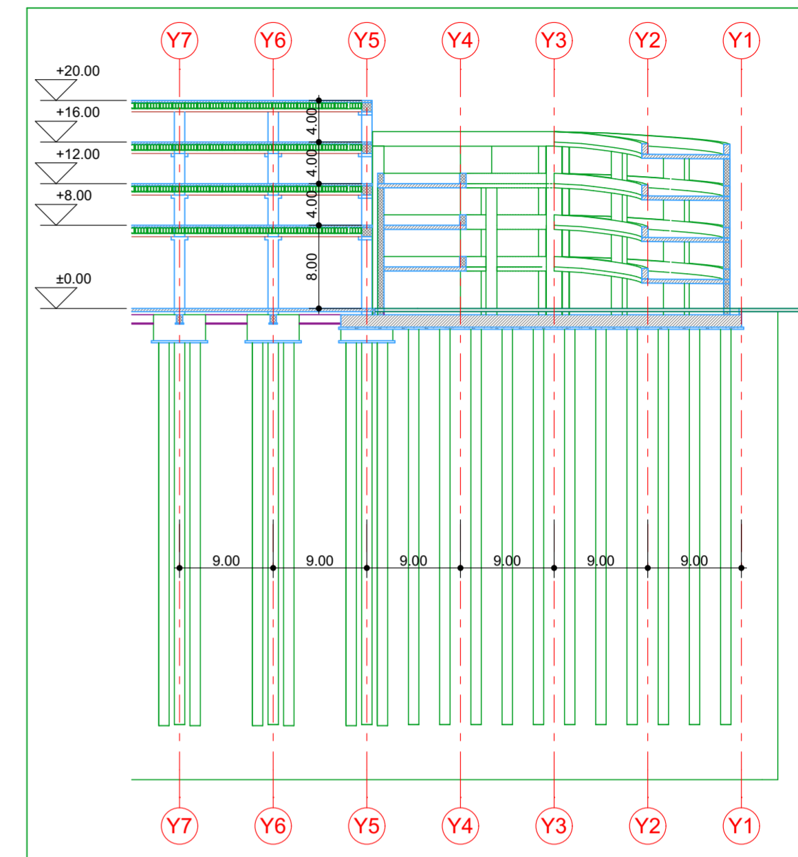
Sezione Edificio S3
