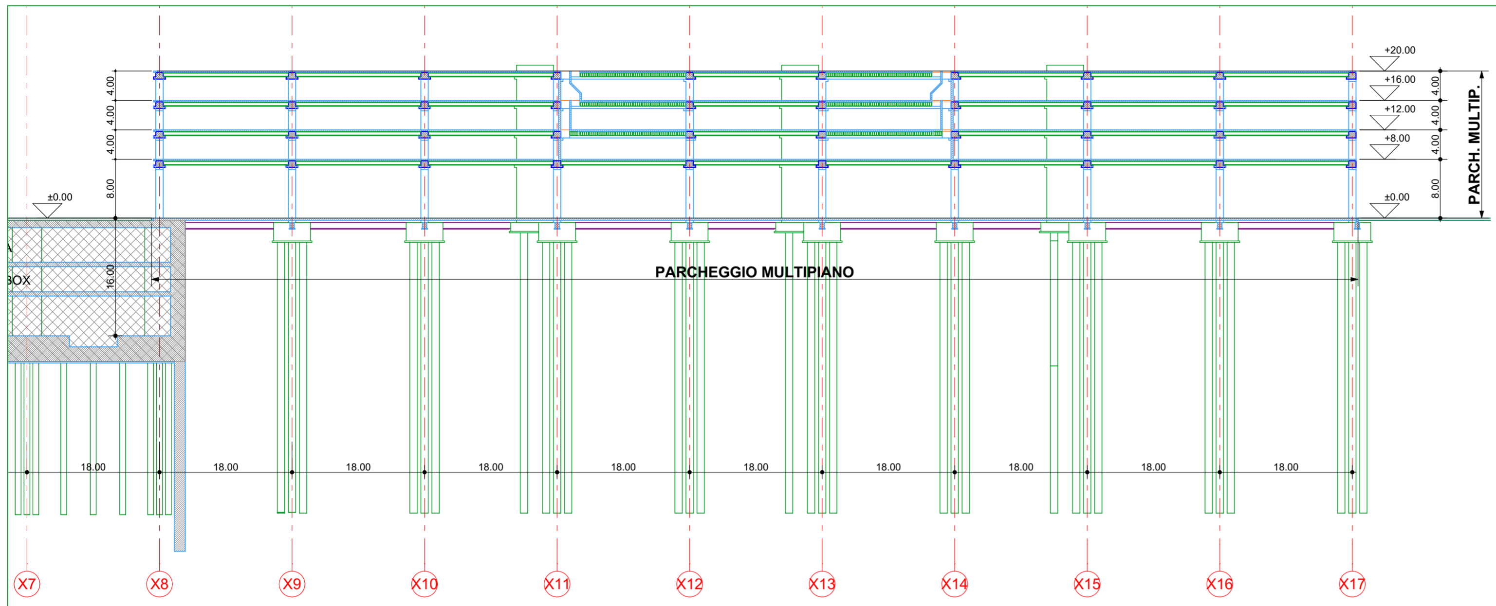
Sezione Edificio S1
