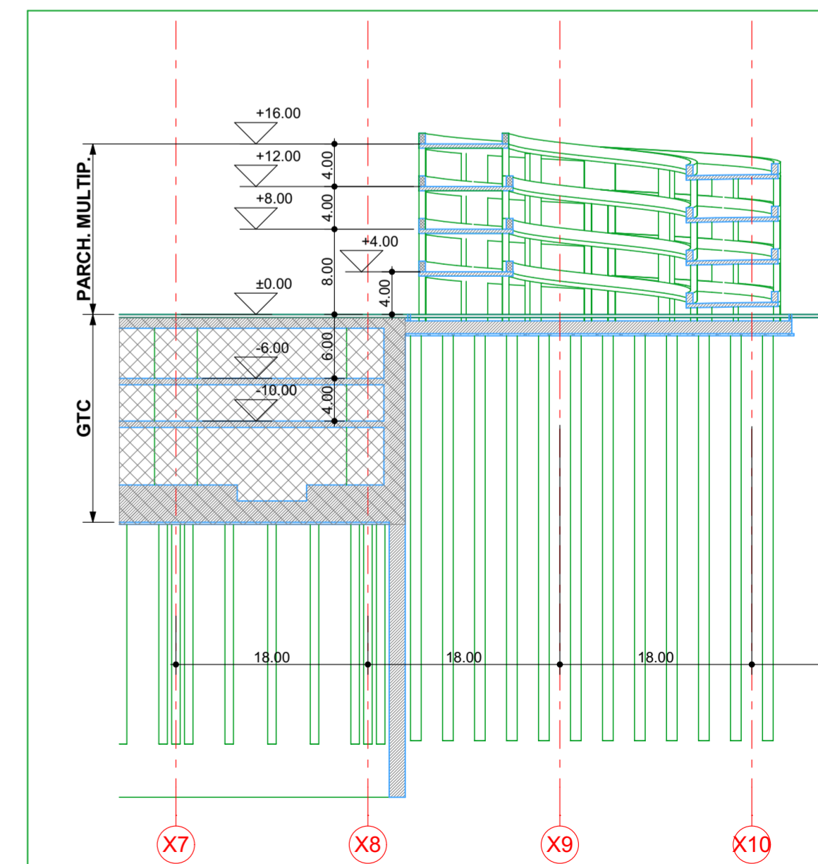
Sezione Edificio S4
