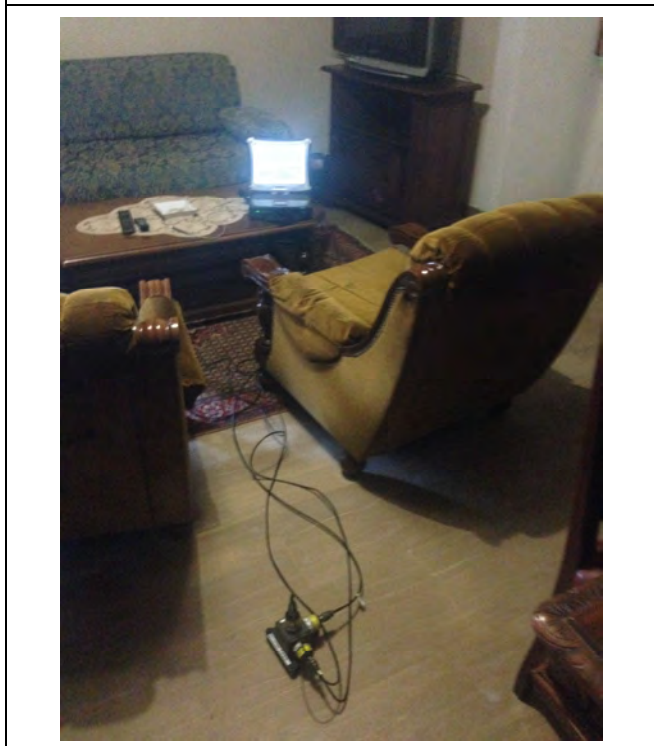
Posizionamento accelerometro triassiale, 1° piano f.t.
