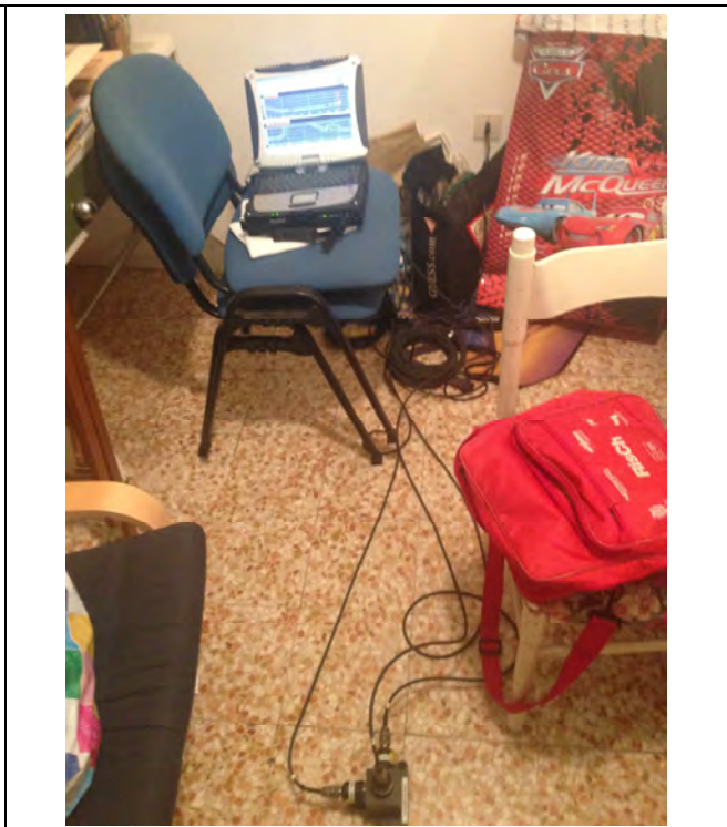
Posizionamento accelerometri monoassiali, 2° piano f.t.
