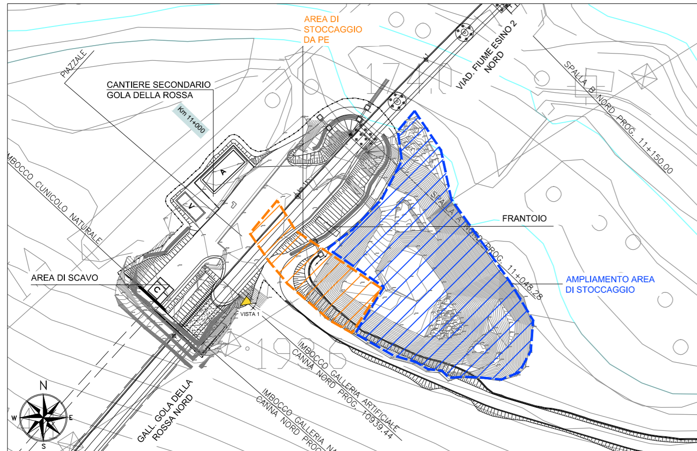
Planimetria
