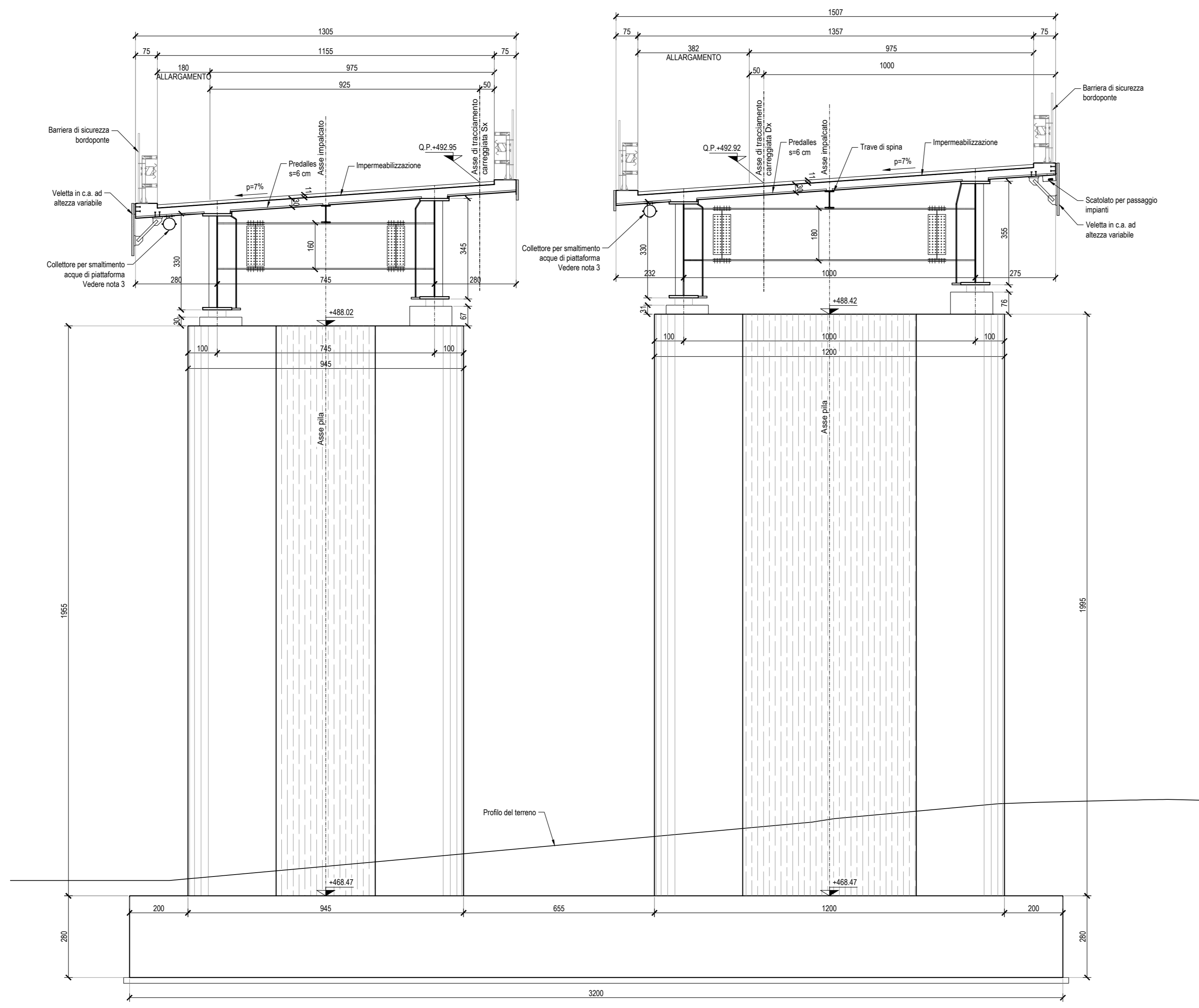
Sezione trasversale su P4SX Scala 1:100
