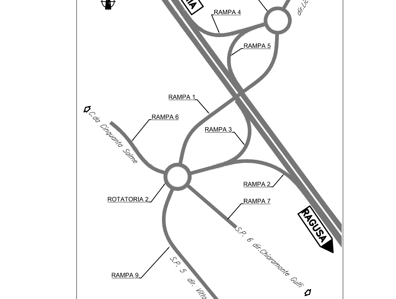
SCHEMA SVINCOLO 3
