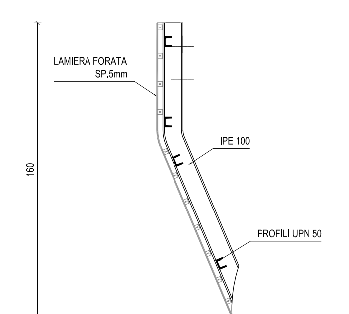
PARTICOLARE VELETTA METALLICA SCALA 1:20 (quote in cm)
