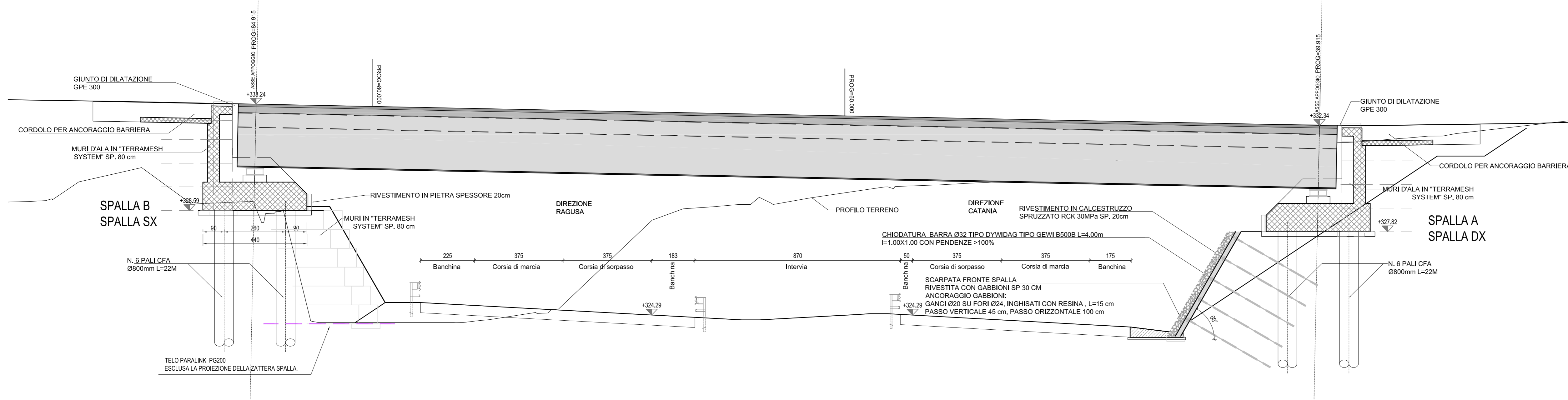
PROSPETTO SCALA 1:100
