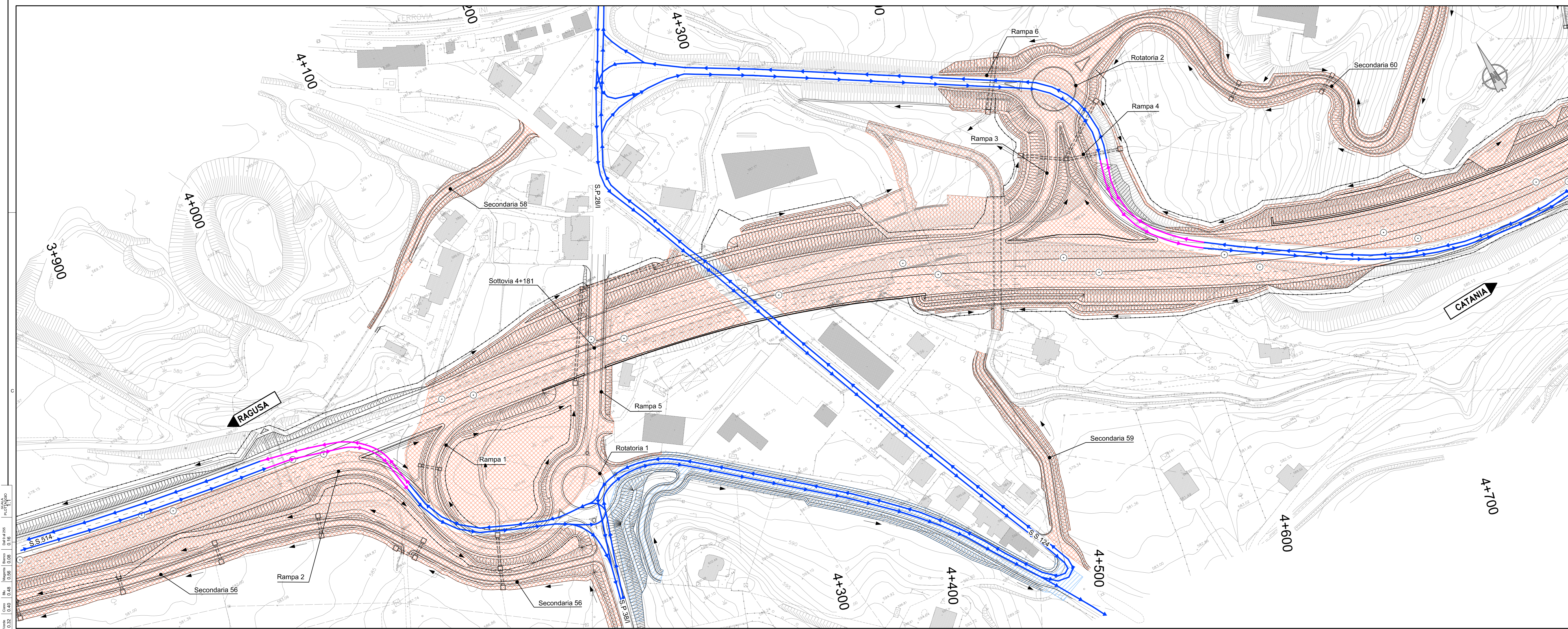
FASE 1 - DEVIAZIONE DEL TRAFFICO DELLA S.S.514 SULLA VIABILITA' DI SVINCOLO ESISTENTE CON COLLEGAMENTO NORD-SUD GARANTITO DAL SOTTOVIA DELLA S.S. 124 - REALIZZAZIONE CARREGGIATA DX E CARREGGIATA SX ASSE PRINCIPALE NELLE PORZIONI ESTERNE ALLA VIABILITA' TRA PROGRESSIVA 4+030-4+550, REALIZZAZIONE CARREGGIATA SX DA PROGRESSIVA 4+650
