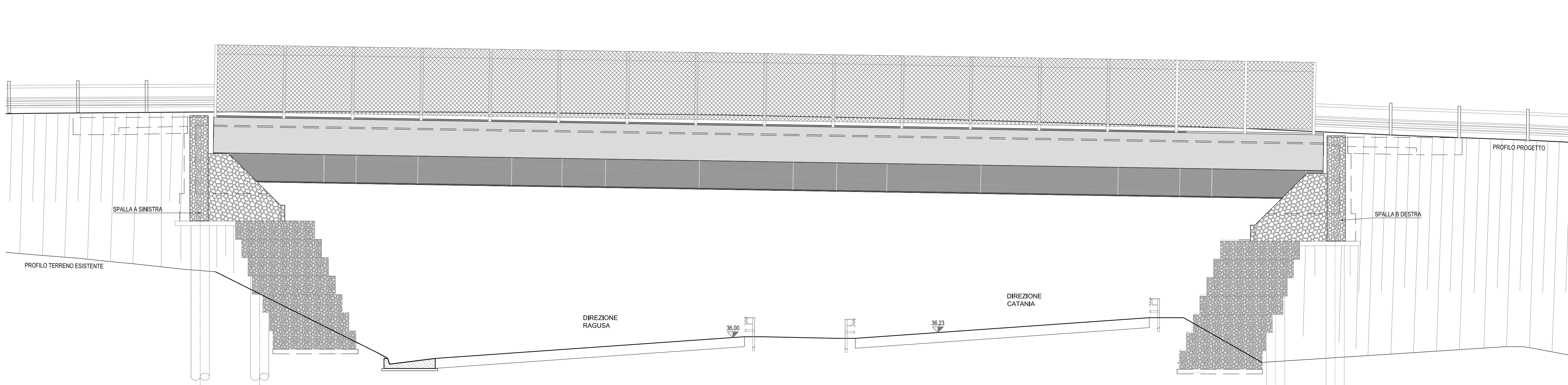
PROSPETTO SCALA 1:100
