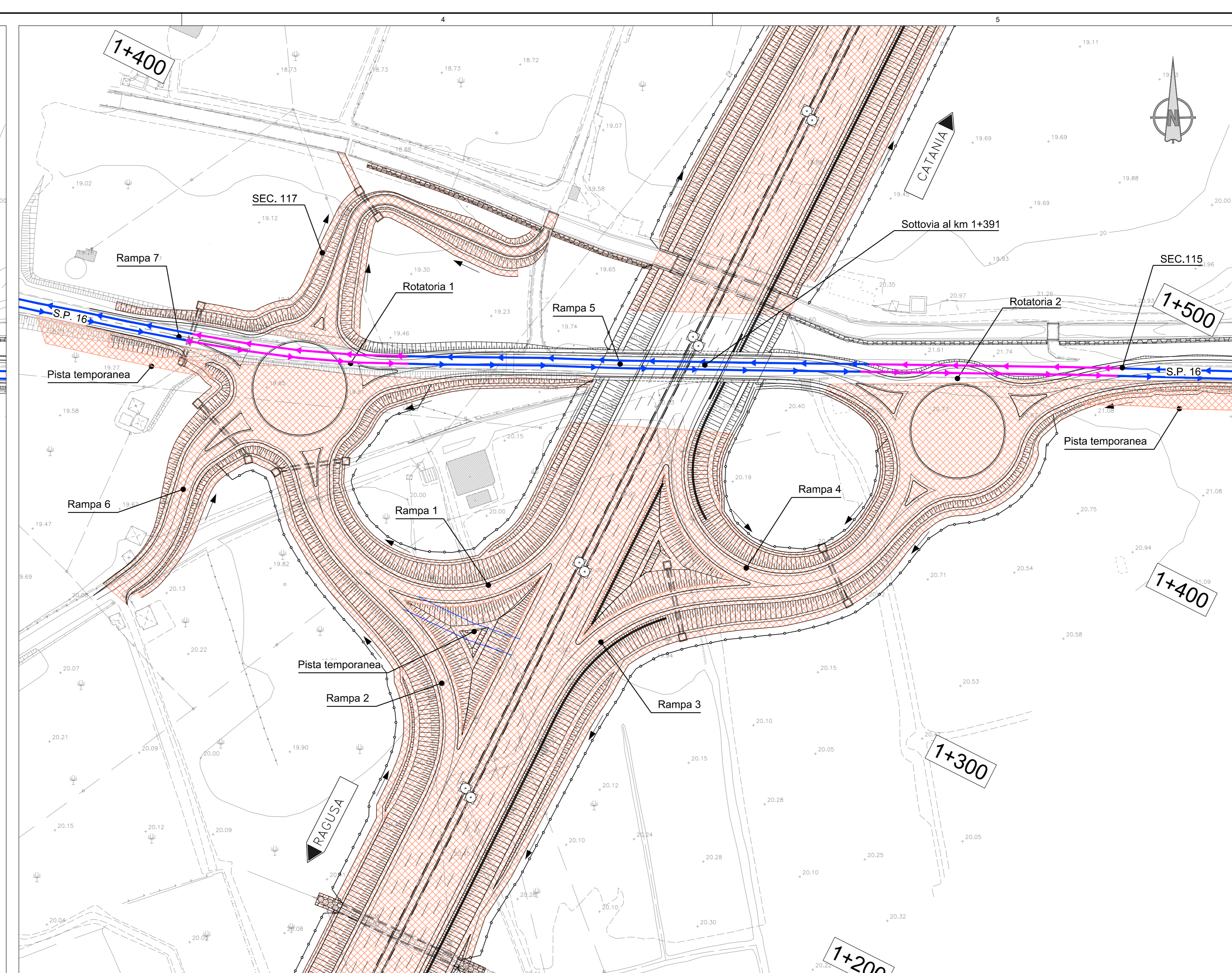
FASE 1 - TRAFFICO SU SEDE ESISTENTE S.P. 16 CON LOCALI RESTRINGIMENTI - REALIZZAZIONE PISTE TEMPORANEE PER DEVIAZIONE TRAFFICO IN FASE 2 - REALIZZAZIONE SECONDARIA 117 E RAMPE 1, 2, 3, 4, 6 E PARZIALE ROTATORIE 1 E 2 FUORI SEDE - REALIZZAZIONE ASSE PRINCIPALE A NORD E A SUD DEL SOTTOVIA
