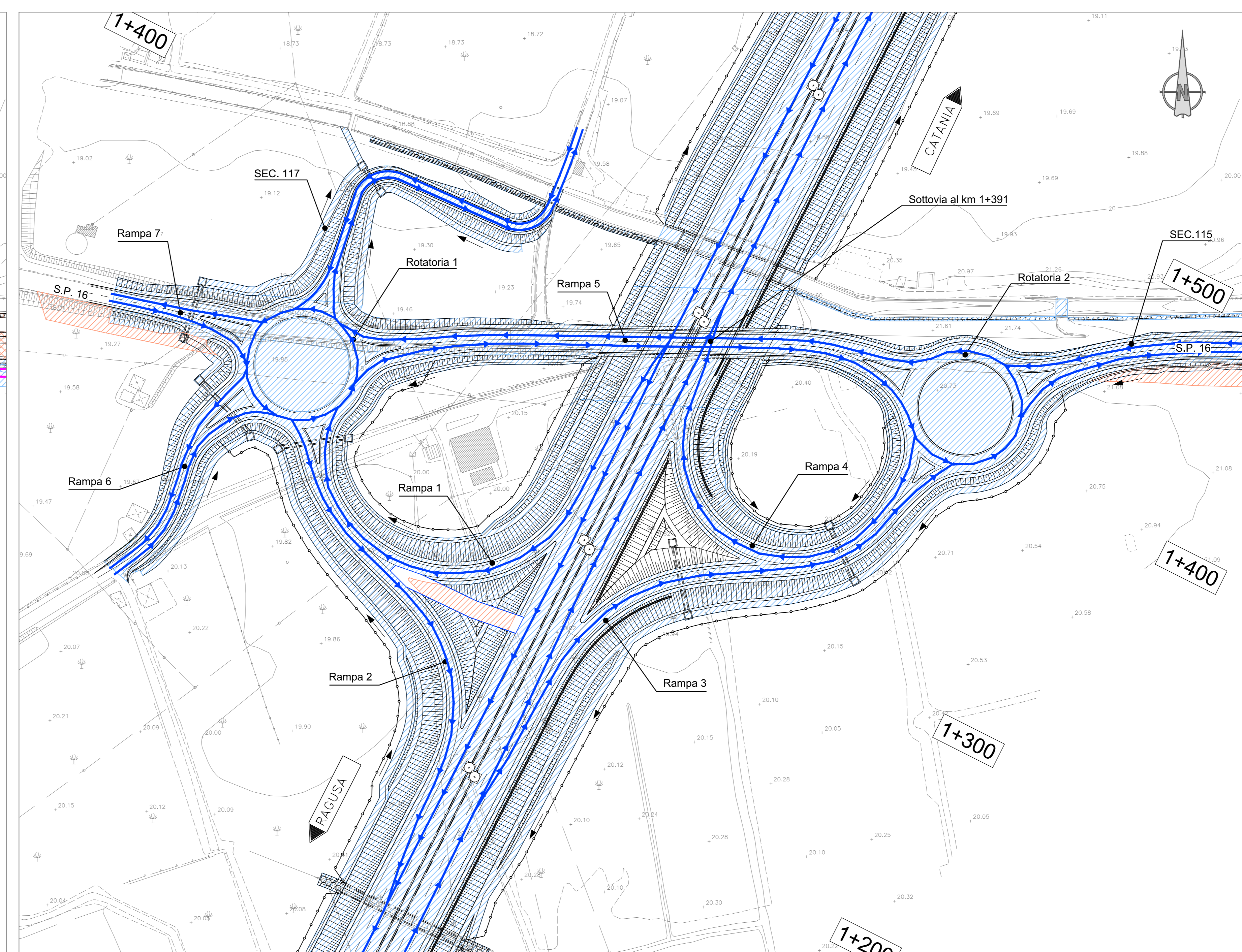
FASE 3 - DEMOLIZIONE PISTE TEMPORANEE E RINATURALIZZAZIONE DELLE AREE - COMPLETAMENTO DELL'INFRASTRUTTURA - APERTURA AL TRAFFICO
