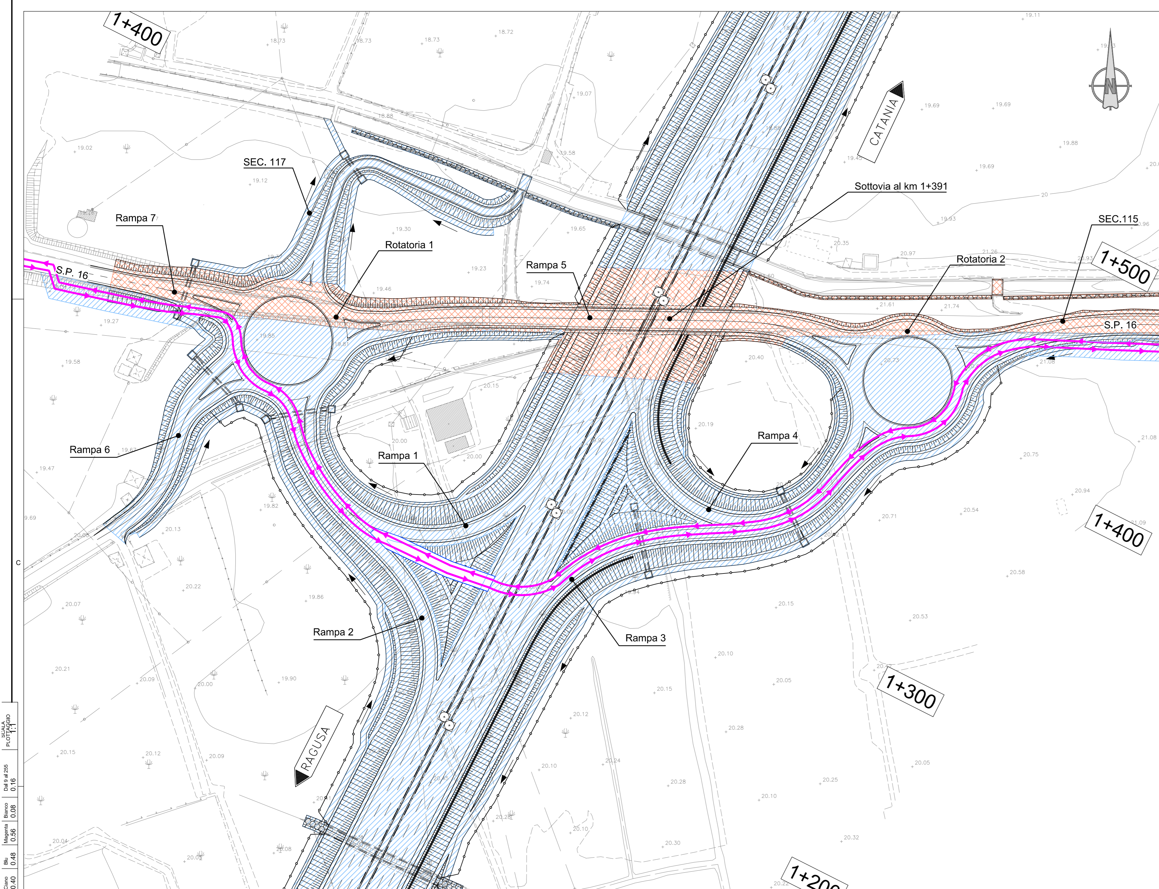
FASE 2 - DEVIAZIONE DEL TRAFFICO SU PISTE TEMPORANEE, ROTATORIA 1-2, RAMPE 1-2-3 E ASSE PRINCIPALE - REALIZZAZIONE DEL SOTTOVIA - COMPLETAMENTO RAMPE DI SVINCOLO E ROTATORIE
