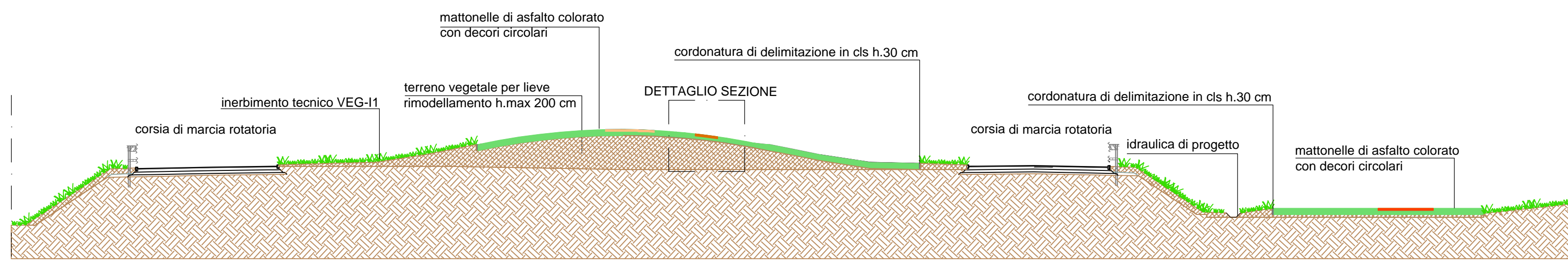
SCHEMA SEZIONE A-A scala 1:200
