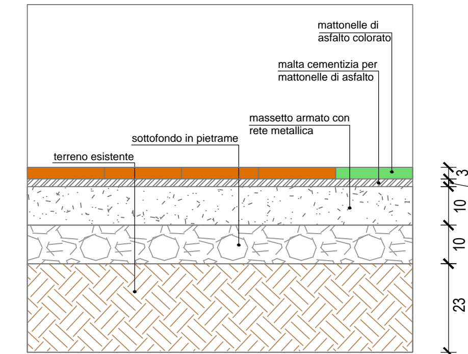
DETTAGLIO SEZIONE A-A scala 1:10
