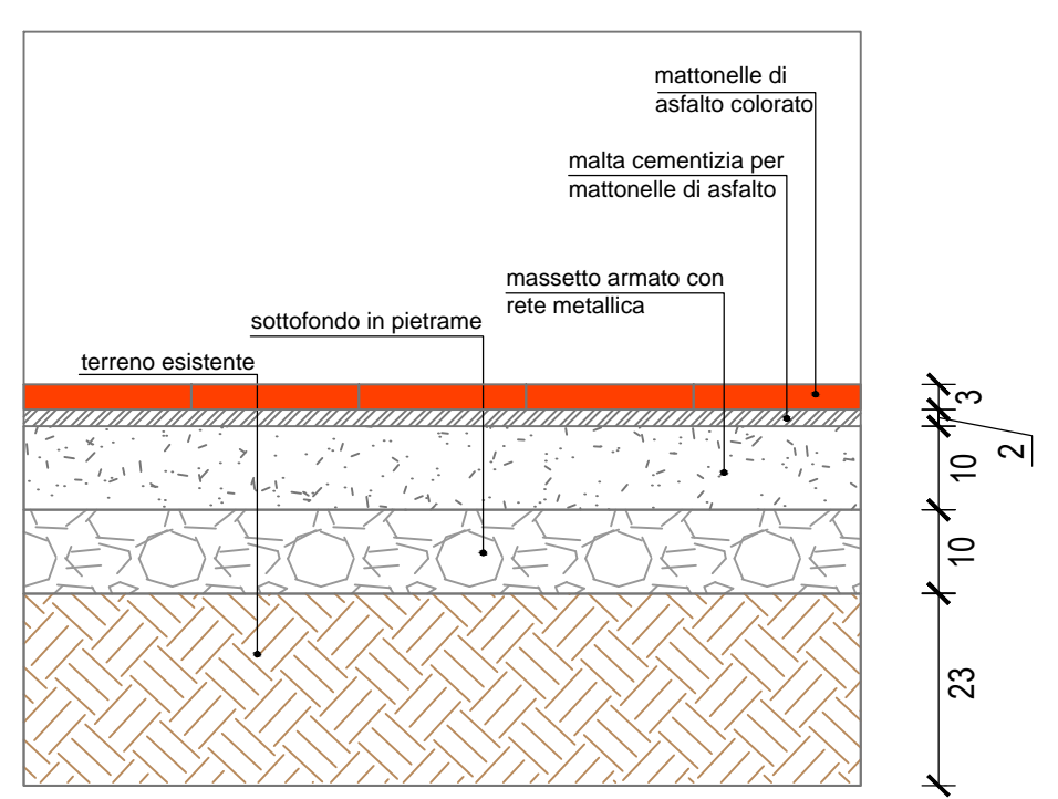
DETTAGLIO SEZIONE A-A scala 1:10
