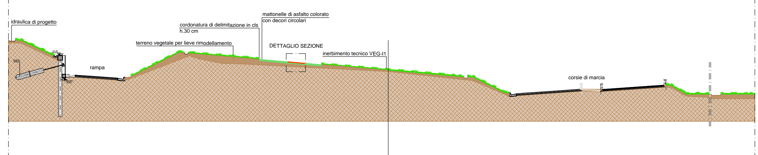
SCHEMA SEZIONE A-A scala 1:500
