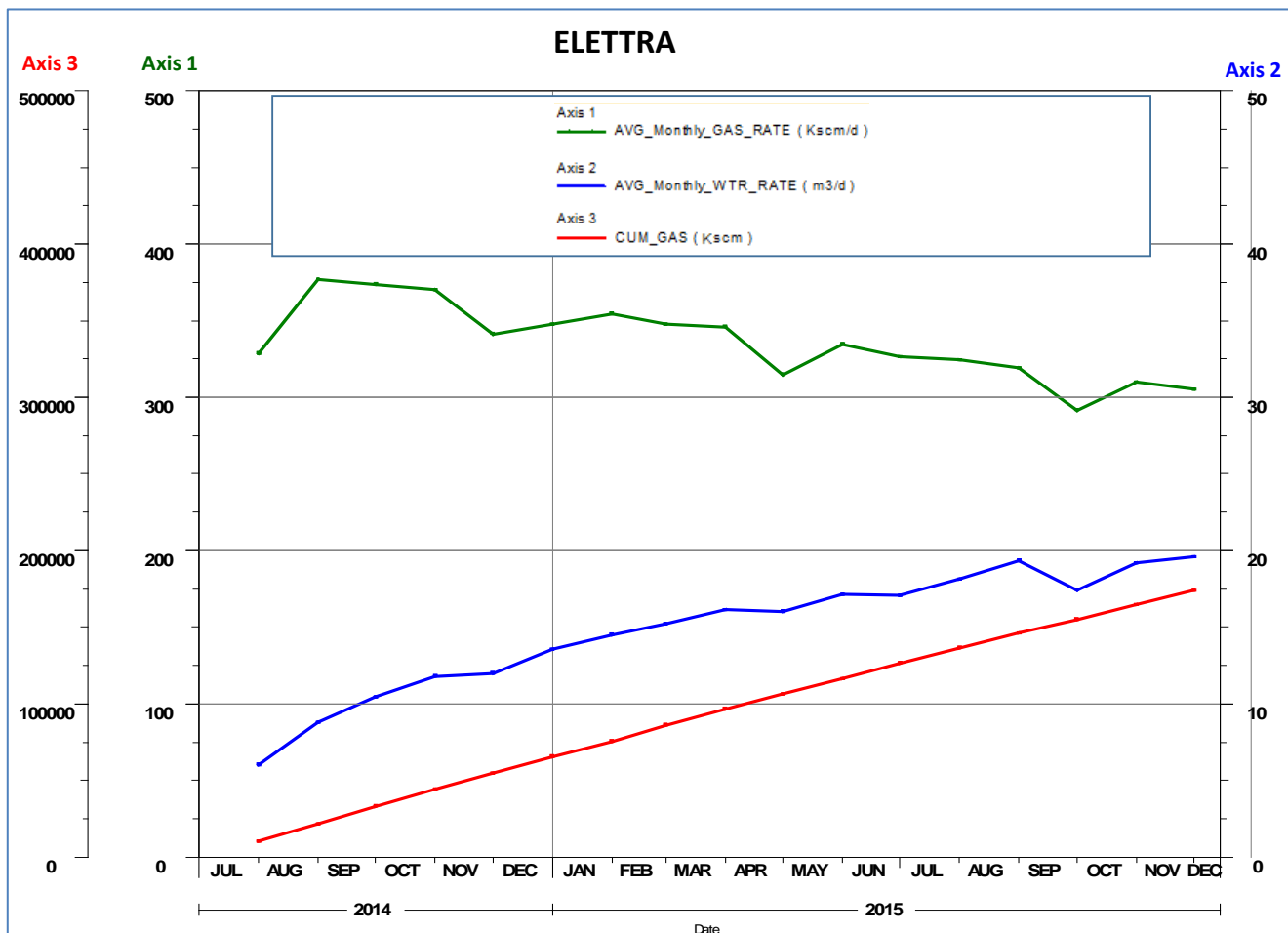
Figura 4 - Campo di Elettra: grafico di produzione storica
