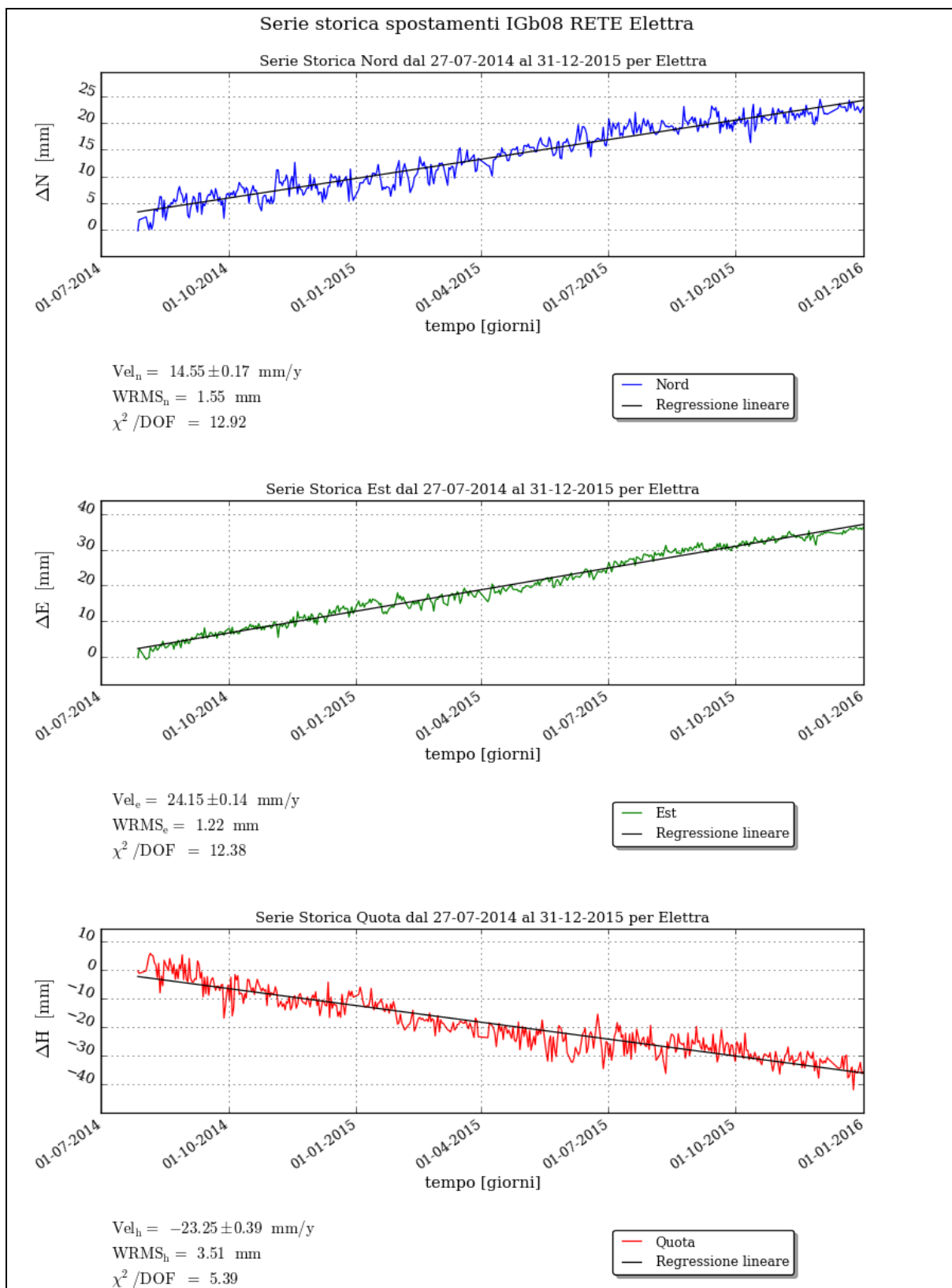
Figura 9 - Campo di Elettra: serie storiche plano-altimetriche CGPS
