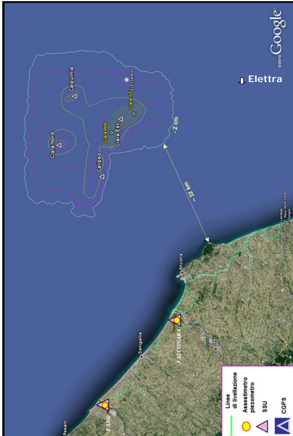
Figura 5 - Curve d'isosubsidenza per lo scenario di riferimento "C m _Med" al 2065. Max subs. su Elettra: 18 cm @ 2065 (modello geomeccanico del sett. 2013)
