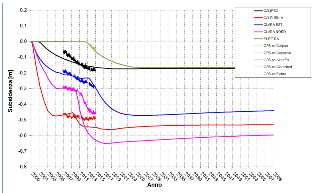
Figura 11 - Andamento temporale della subsidenza prevista da modello geomeccanico (sett. 2013), scenario Cm_Med, in corrispondenza delle p.me di produzione vs. le misure altimetriche da CGPS aggiornato al dic. 2015
