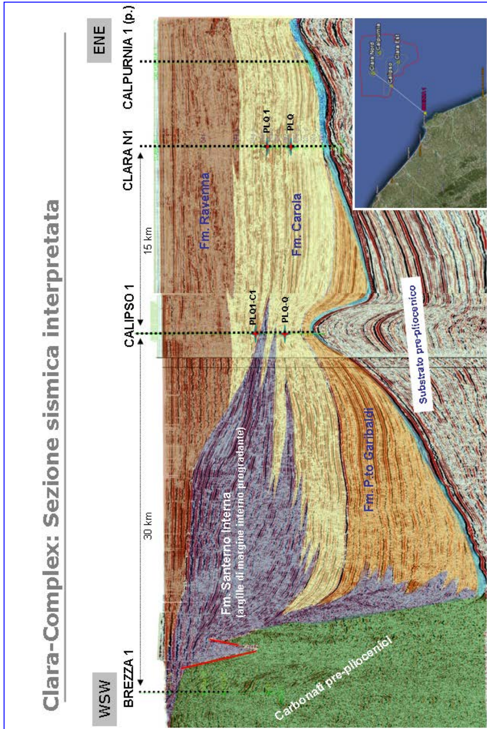
Figura 6 - Sezione sismica interpretata
