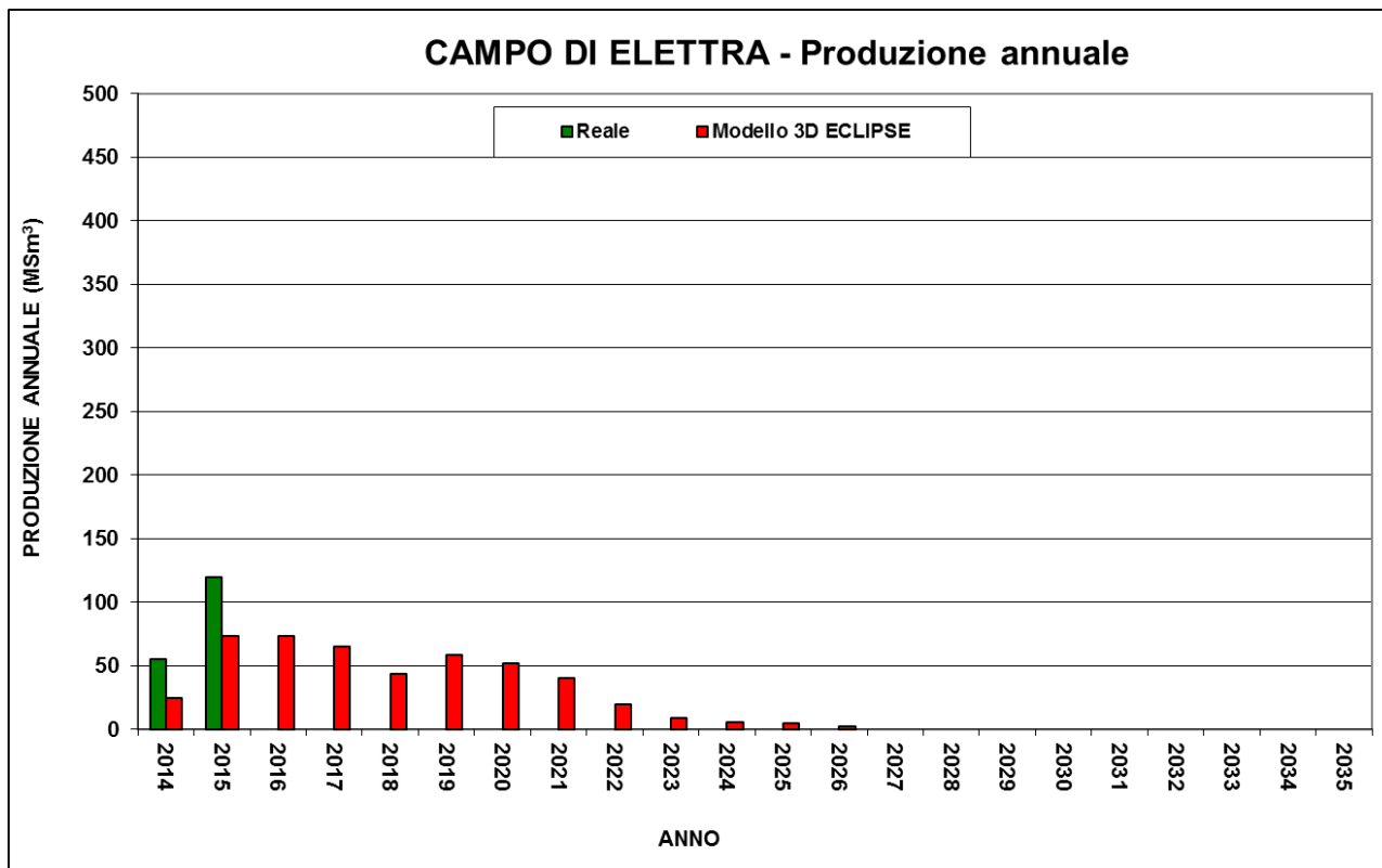
Figura 3 - Campo di Elettra: tabella e grafico di produzione vs. modello Eclipse (agosto 2010)
