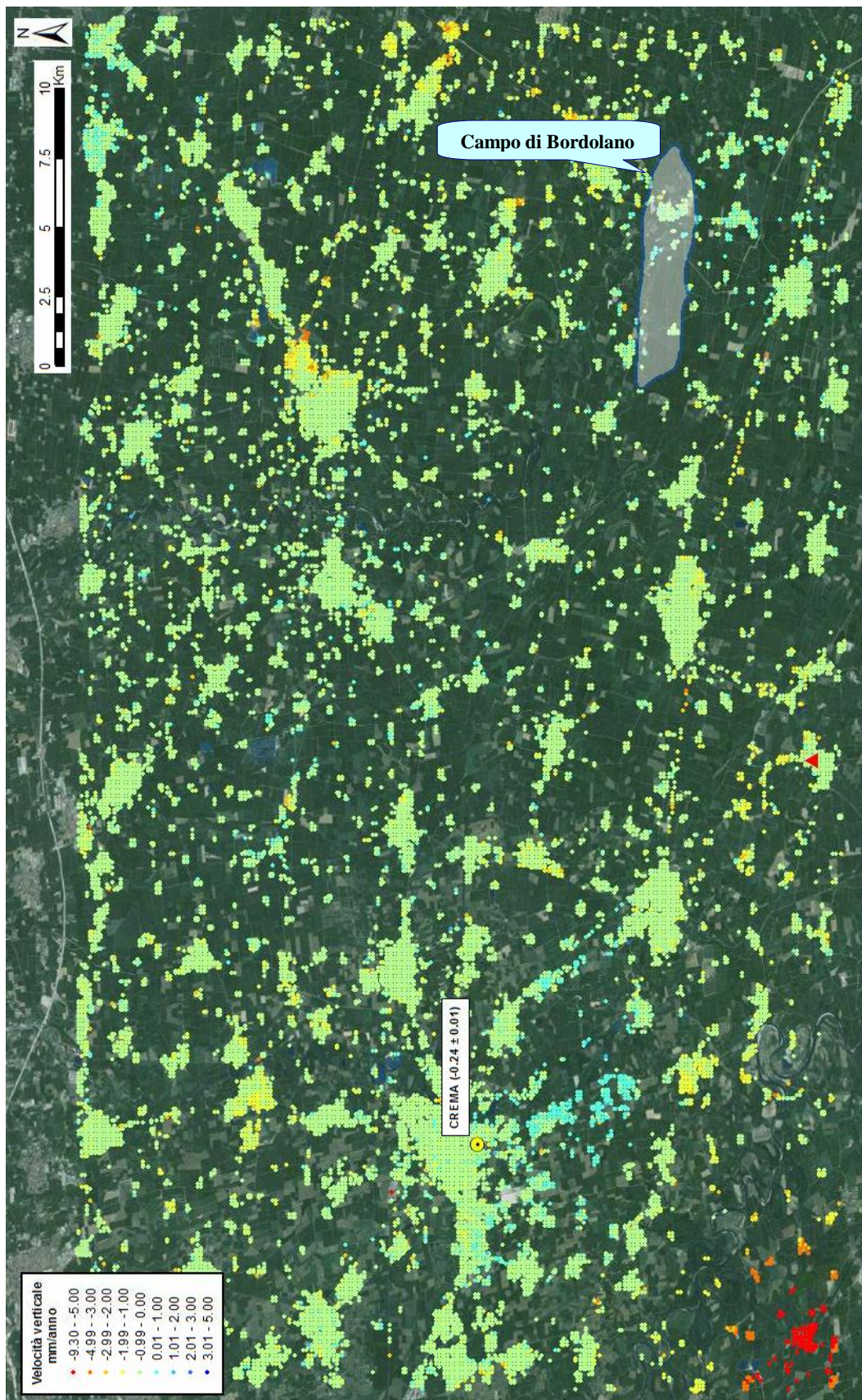
Fig. 10 – Dati Regional scomposti secondo il vettore verticale e calibrati. In evidenza l'ubicazione del CGPS di Crema utilizzato per la calibrazione, il punto di riferimento (triangolo rosso) ed i limiti del giacimento.
