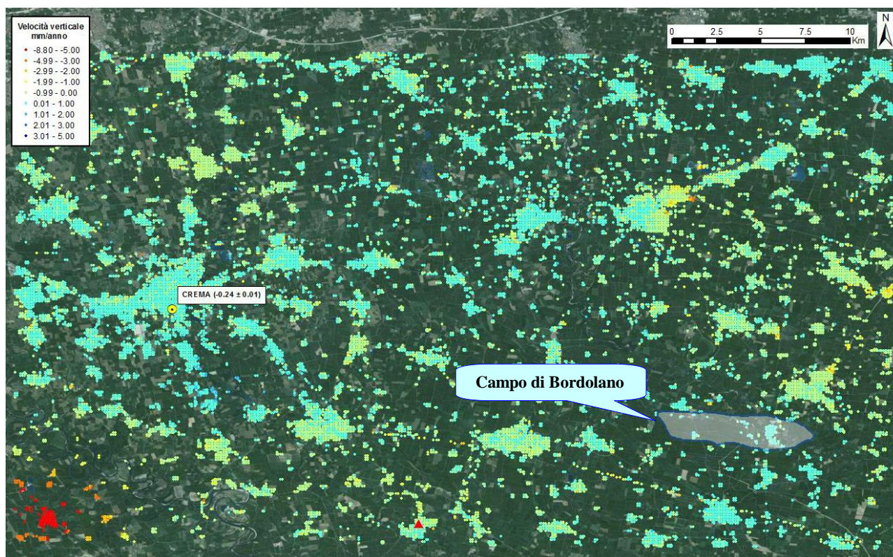
Fig. 7 – Dati dell’analisi Regional in scala di colori. I valori si riferiscono al solo vettore verticale risultato dalla scomposizione dei dati originali. Il triangolo rosso indica la posizione del punto di riferimento utilizzato per la scomposizione ed in giallo il GPS di Crema utilizzato per la calibrazione del dataset.
