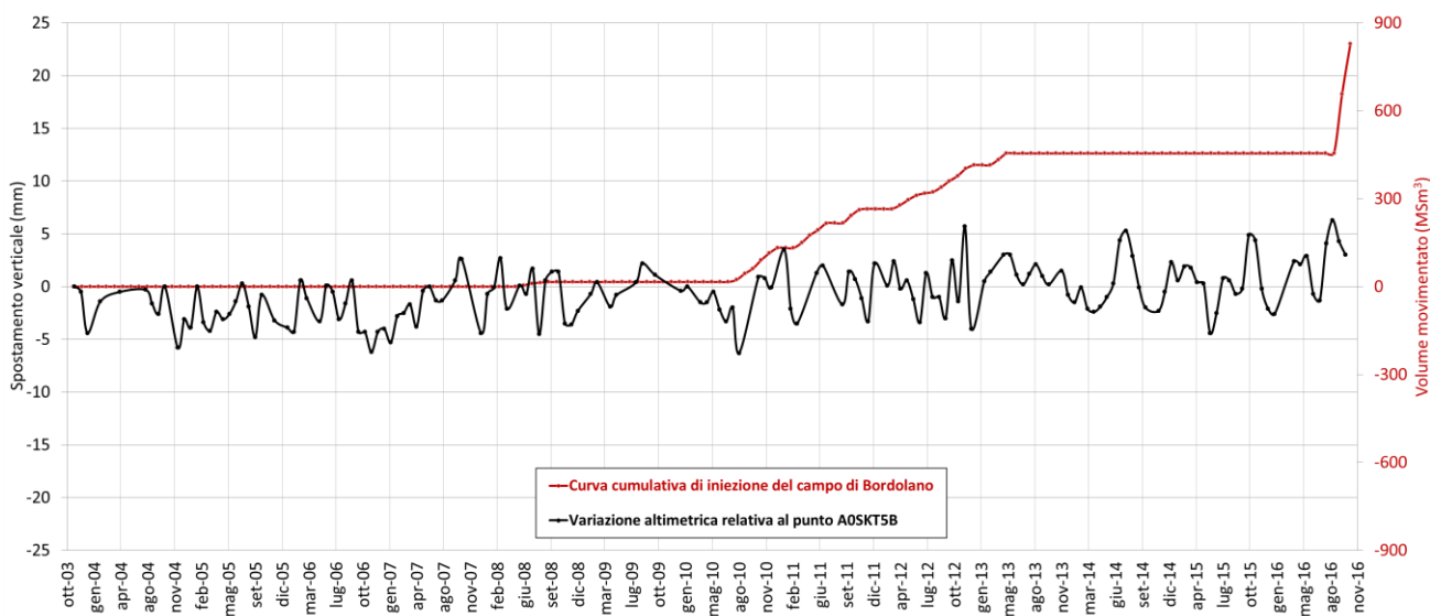
Fig. 24 – In alto, ubicazione del punto scomposto A0SKT5B con evidenza dei PS ascendenti e discendenti presenti nelle vicinanze e loro coerenza. In basso, confronto tra l'andamento temporale delle variazioni altimetriche del punto scomposto A0SKT5B e la curva di iniezione del giacimento di Bordolano.
