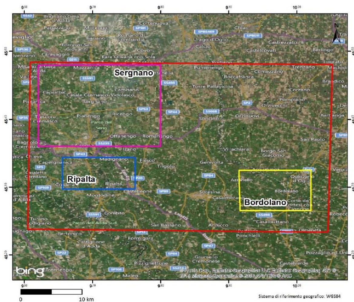
Fig. 4 – Estensione dell'area Regional di Crema rispetto alle tre aree Local di Ripalta, Sergnano e Bordolano.
