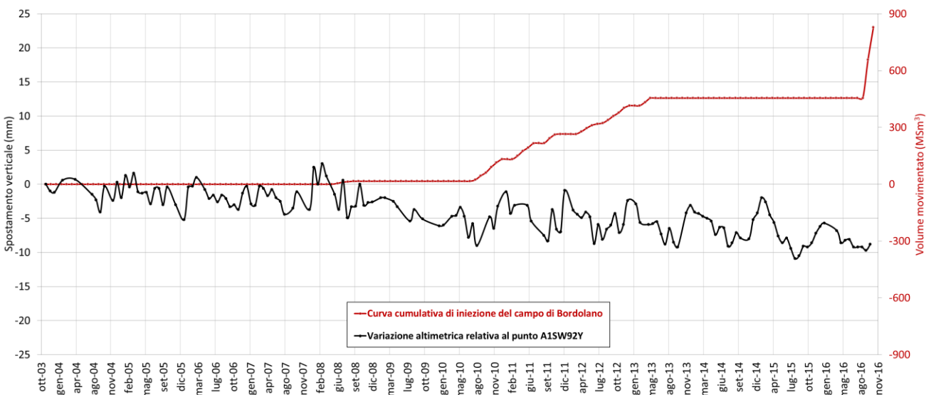
Fig. 28 – In alto, ubicazione del punto scomposto A1SW92Y con evidenza dei PS ascendenti e discendenti presenti nelle vicinanze e loro coerenza. In basso, confronto tra l'andamento temporale delle variazioni altimetriche del punto scomposto A1SW92Ye la curva di iniezione del giacimento di Bordolano.
