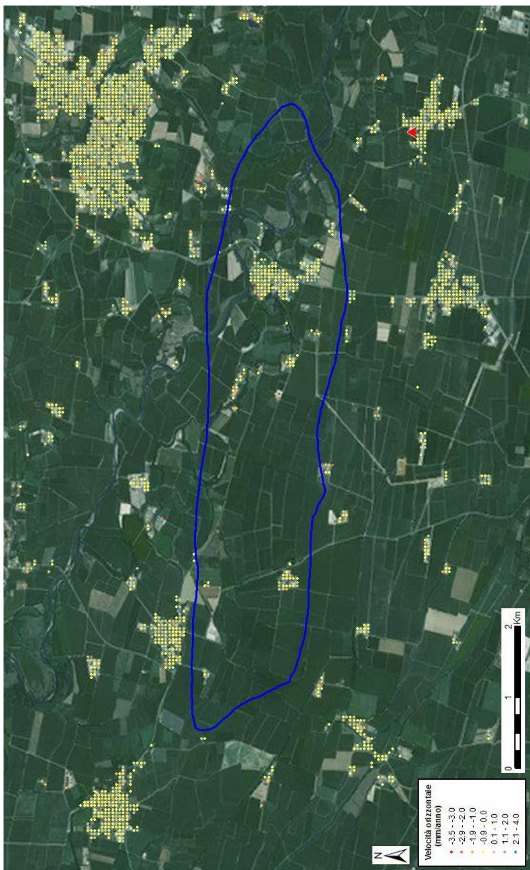
Fig. 16 – Visualizzazione in scala di colori delle velocità orizzontali dei punti scomposti dell’analisi Local.
