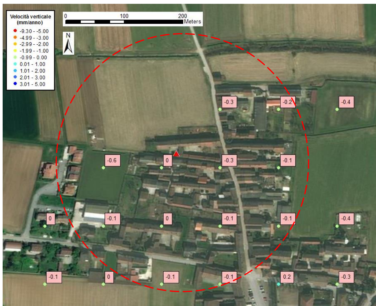
Fig. 17 – Visualizzazione del punto di riferimento utilizzato per la scomposizione Local (triangolo rosso) ed indicazione dei punti Regional più vicini con i rispettivi valori di velocità calibrati ed arrotondati ad una cifra decimale. L'area per la quale è stata calcolata la media delle velocità verticali è delimitata da un cerchio avente un raggio di circa 200 metri.
