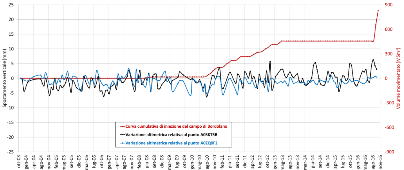
Fig. 30 – Confronto tra la curva di iniezione del giacimento di Bordolano e le serie storiche dei punti scelti all'interno dei limiti del campo.
