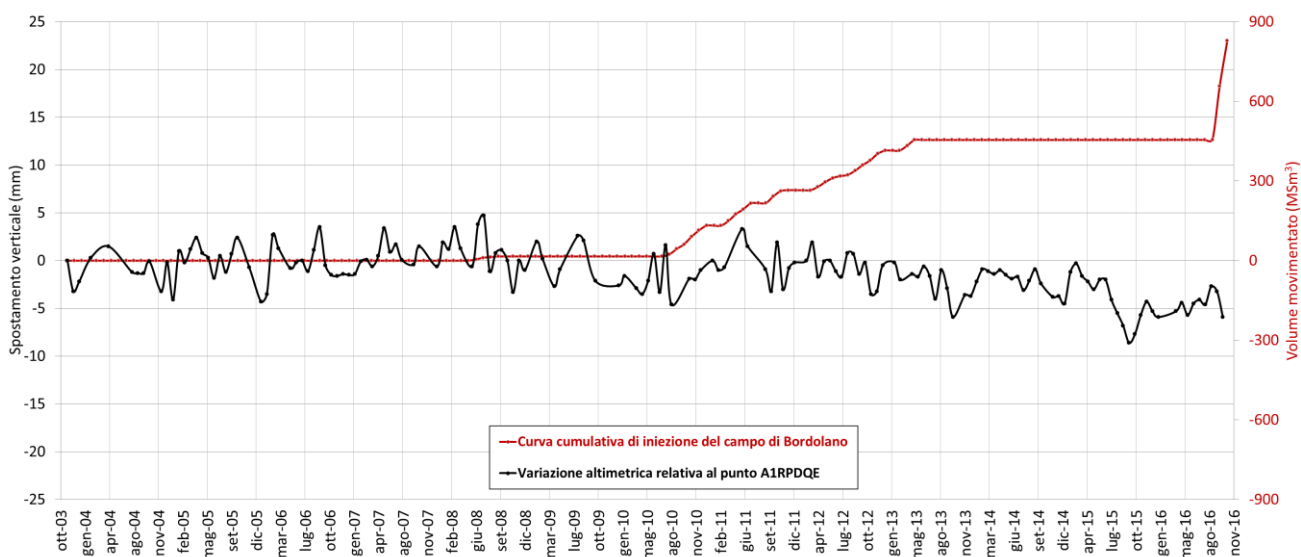
Fig. 26 – In alto, ubicazione del punto scomposto A1RPDQE con evidenza dei PS ascendenti e discendenti presenti nelle vicinanze e loro coerenza. In basso, confronto tra l'andamento temporale delle variazioni altimetriche del punto scomposto A1RPDQE e la curva di iniezione del giacimento di Bordolano.
