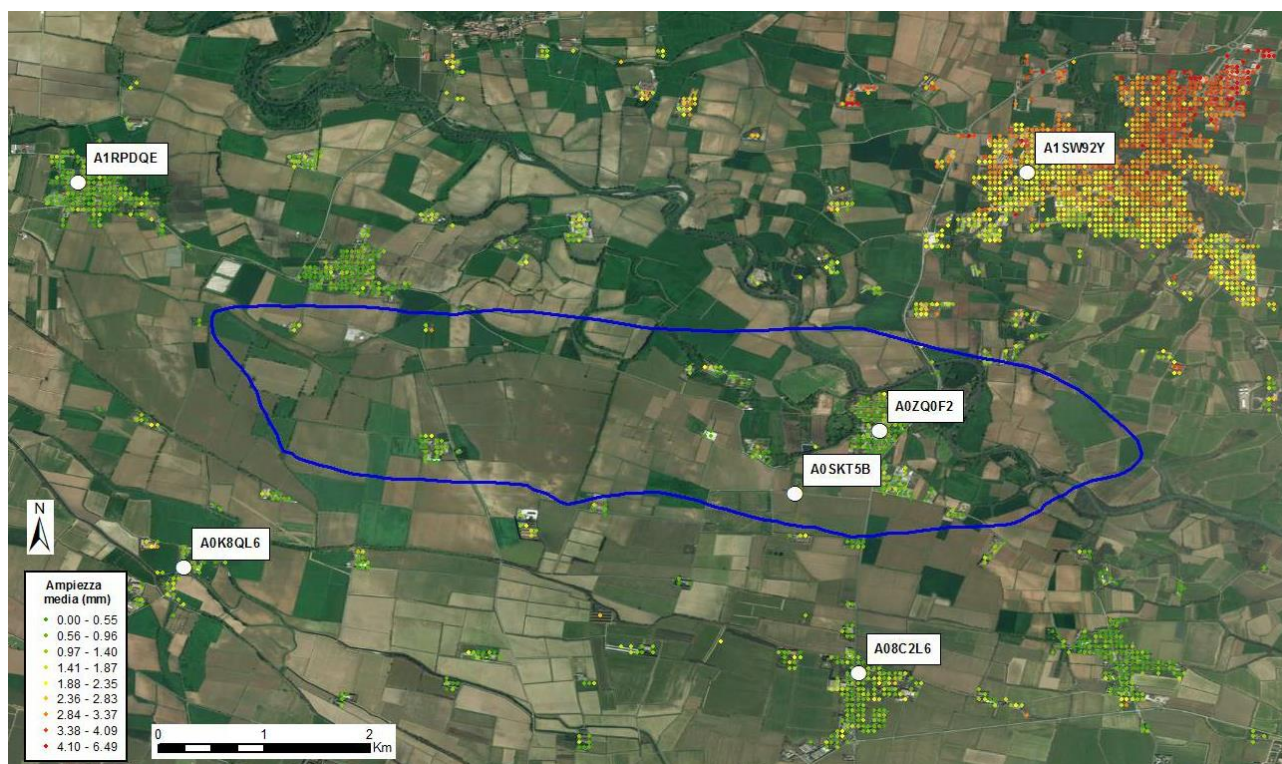
Fig. 22 – Valori medi di ampiezza della stagionalità calcolati per la componente verticale dei PS Local ed ubicazione dei 2 punti interni e dei 4 punti esterni alla proiezione in superficie del limite del giacimento.
