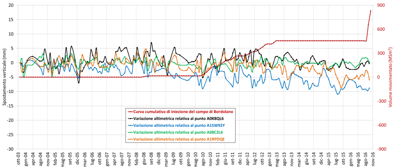
Fig. 31 – Confronto tra la curva di iniezione del giacimento di Bordolano e le serie storiche dei punti scelti all'esterno dei limiti del campo.
