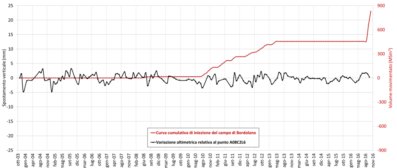
Fig. 29 – In alto, ubicazione del punto scomposto A08C2L6 con evidenza dei PS ascendenti e discendenti presenti nelle vicinanze e loro coerenza. In basso, confronto tra l'andamento temporale delle variazioni altimetriche del punto scomposto A08C2L6 e la curva di iniezione del giacimento di Bordolano.
