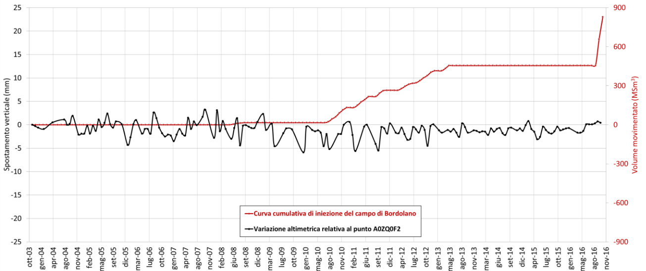
Fig. 25 – In alto, ubicazione del punto scomposto A0ZQ0F2 con evidenza dei PS ascendenti e discendenti presenti nelle vicinanze e loro coerenza. In basso, confronto tra l'andamento temporale delle variazioni altimetriche del punto scomposto A0ZQ0F2 e la curva di iniezione del giacimento di Bordolano.
