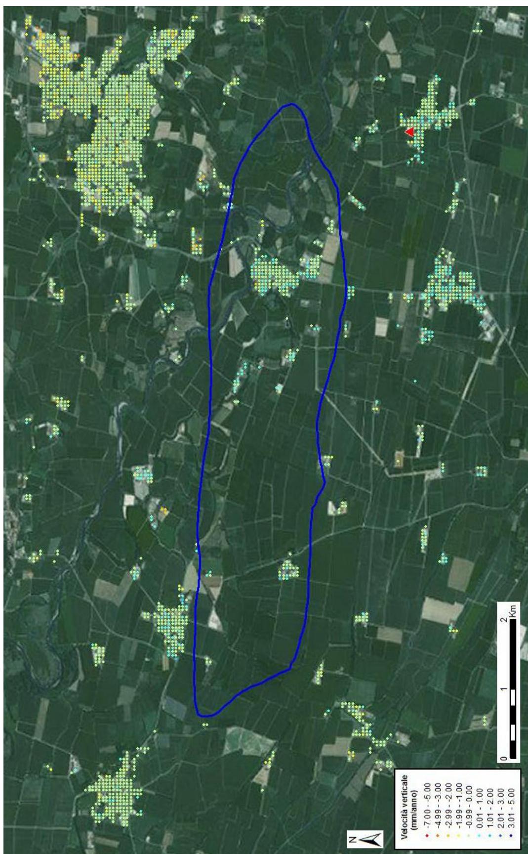
Fig. 15 – Visualizzazione in scala di colori delle velocità verticali dei punti scomposti dell’analisi Local, così come registrati dal satellite prima della calibrazione.
