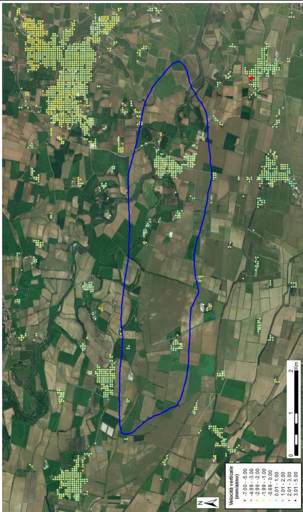
Fig. 19 – Visualizzazione in scala di colori delle velocità verticali dei punti scomposti dell'analisi Local dopo la variazione di -0.16 mm/anno effettuata sull'intero dataset. Il triangolo rosso indica la posizione del punto di riferimento utilizzato per la scomposizione del vettore velocità.
