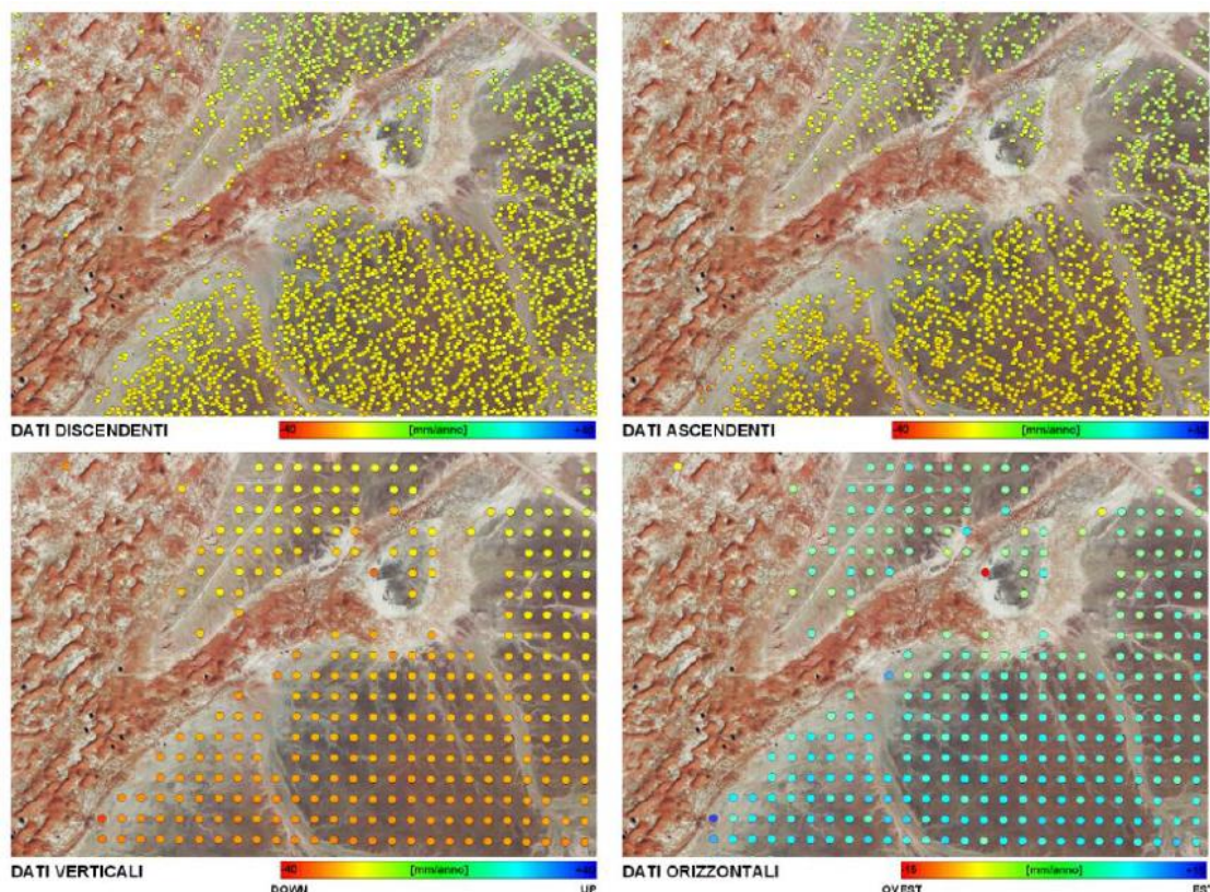
Fig. 3 – Trasformazione dei dati di spostamento dei PS/DS su griglia regolare. In alto i risultati ottenuti dai PS/DS, in basso gli stessi ricampionati su griglia regolare per la scomposizione del moto.
