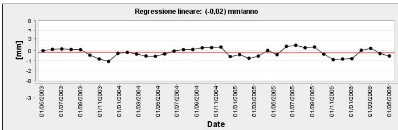
Fig. 21 – Esempio di serie storica con valori di regressione lineare nulla.
