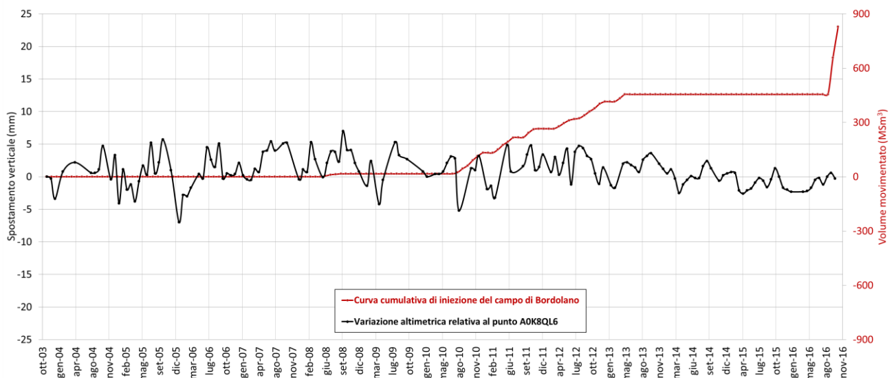
Fig. 27 – In alto, ubicazione del punto scomposto A0K8QL6 con evidenza dei PS ascendenti e discendenti presenti nelle vicinanze e loro coerenza. In basso, confronto tra l'andamento temporale delle variazioni altimetriche del punto scomposto A0K8QL6 e la curva di iniezione del giacimento di Bordolano.
