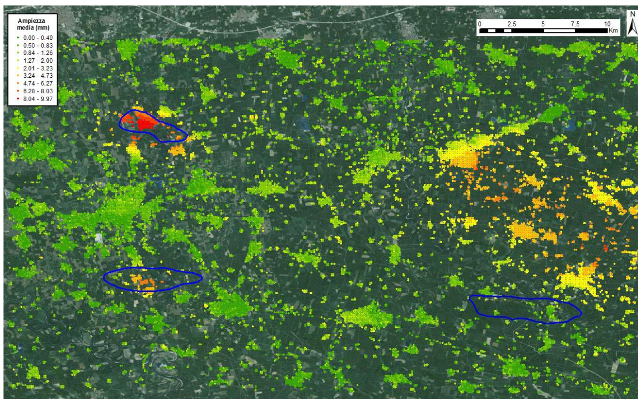
Fig. 12 – Dettaglio dei valori di ampiezza media della stagionalità per la componente verticale del rilievo Regional ed in blu le proiezioni in superficie dei giacimenti di Sergnano (a NW), Ripalta (a SW) e Bordolano (a SE).
