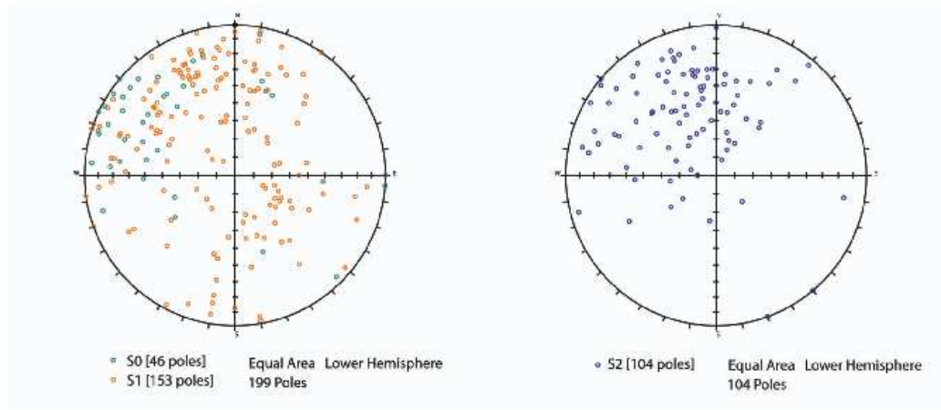
Figura 26 - Proiezione stereografica dei poli delle scissosità S1 e S2 nell'area di Cravasco-Isoverde (reticolo di Schmidt, emisfero inferiore); nel diagramma di sinistra sono state incluse anche le scissosità S0 misurate nelle Dolomie del Monte Gazzo.
