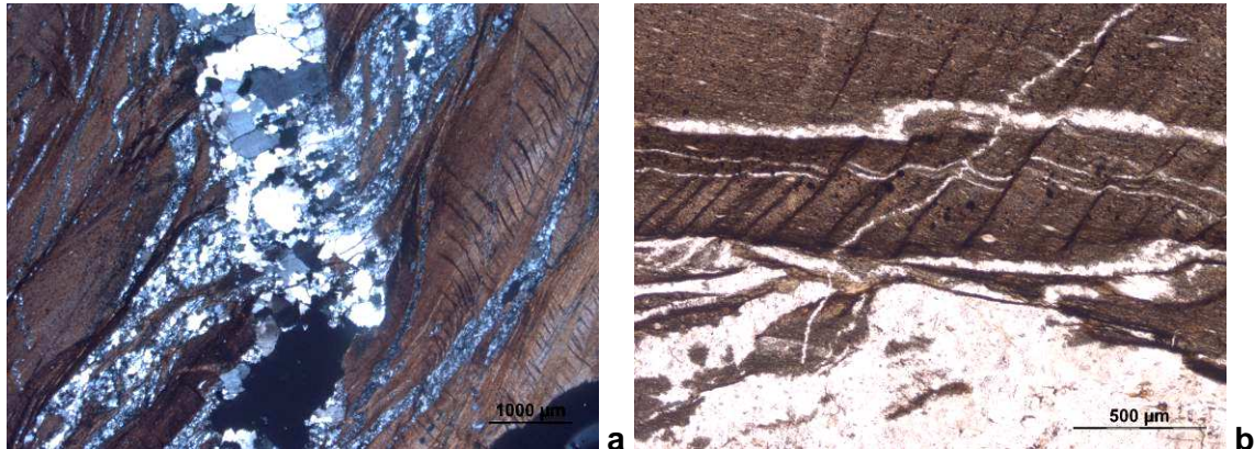
Figura 11 – (a): foliazione principale della roccia, con vene a quarzo sia parallele sia discordanti. La foliazione principale (S1+S2) è crenulata da una fase deformativa successiva (D3 probabile); (b): intersezione tra due generazioni di vene di quarzo; si noti il clivaggio di fase D3 probabile.
