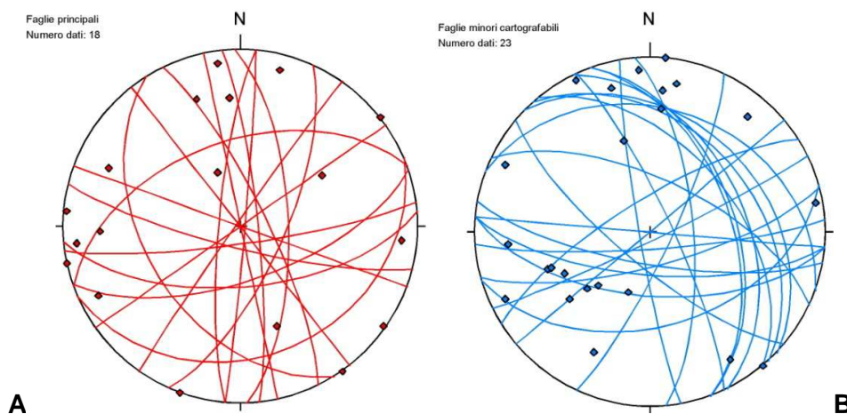
Figura 30 – Set di faglie cartografabili osservate nella zona di Cravasco-Isoverde. A: faglie principali (con potenza delle rocce di faglia superiore a 100 cm); B: faglie minori (con rocce di faglia di spessore centimetrico-decimetrico). Proiezione equiareale di Schmidt, emisfero inferiore.
