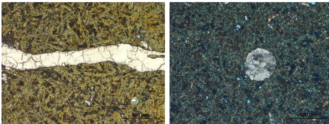
Figura 9 – (a): nonostante la totale sostituzione da parte di pumpellyite l'originaria struttura intersertale a grana fine della vulcanite è ancora perfettamente riconoscibile. La roccia è tagliata da una vena a carbonato; (b) originaria bolla nella vulcanite riempita da carbonato.
