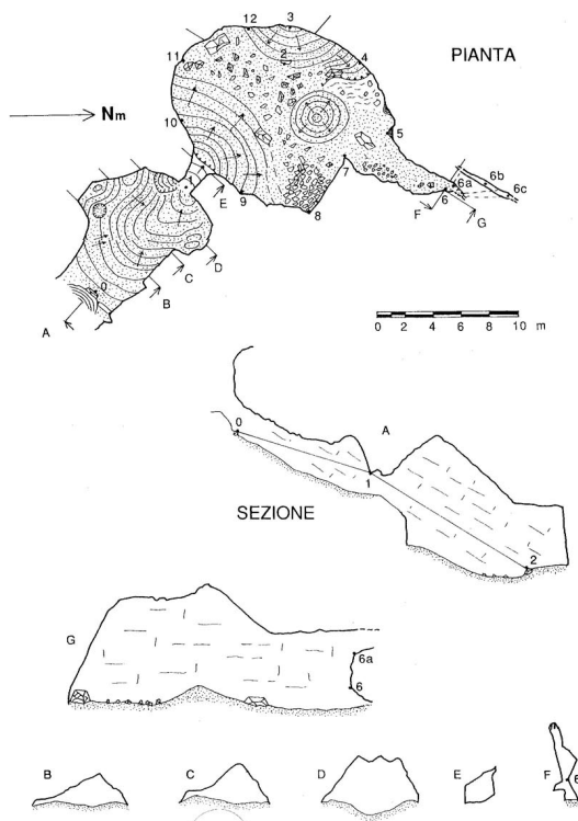
Figura 35 – Sistema carsico di Isoverde, Grotta del Drago. Planimetria e sezioni.
