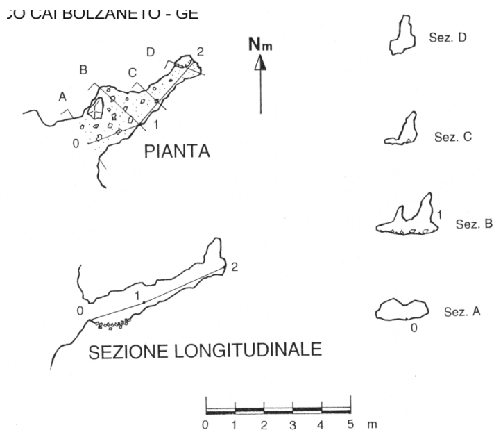
Figura 36 – Sistema carsico di Isoverde, Grotta della Strega. Planimetria e sezioni.
