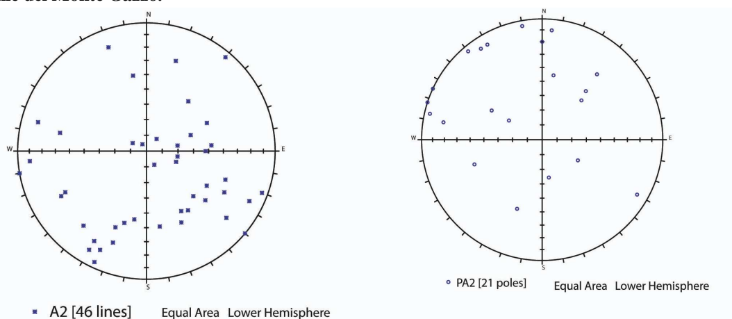
Figura 27 - Proiezione stereografica degli assi di piega (A2) e dei poli di piani assiali (PA2) relativi alla fase D2 nell'area di Cravasco-Isoverde (reticolo di Schmidt, emisfero inferiore).
