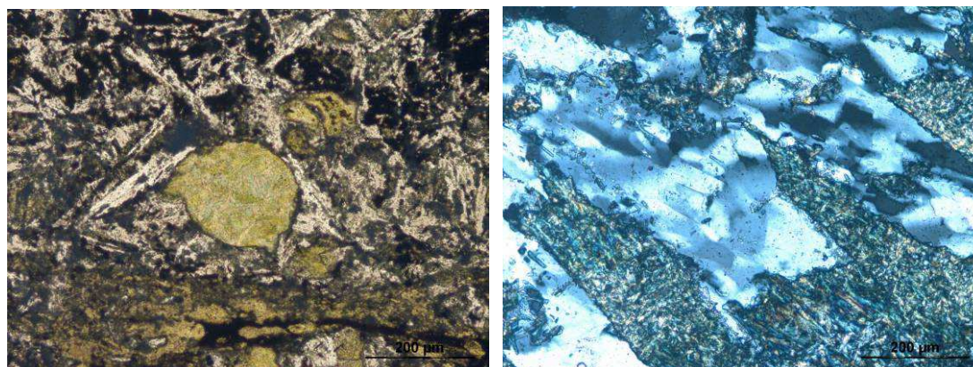
Figura 16 – (a): originaria cavità (bolla) della lava, riempita da pumpellyite a grana fine; (b): grossi cristalli di quarzo circondati da mica bianca.
