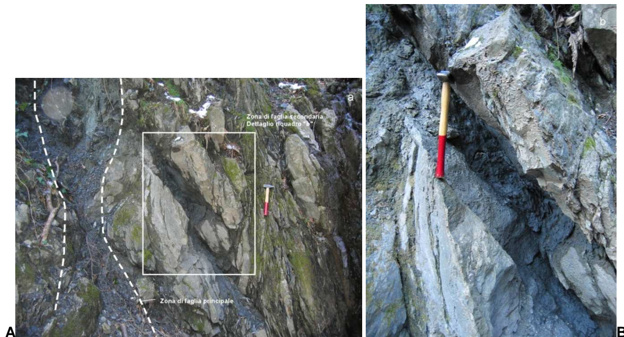
Figura 32 - Faglia all'interno degli argilloscisti nei dintorni di Case Noage (progressiva della Galleria di Valico 9+700 ca.). Si notino le superfici di movimento caratterizzate da gouge non coesivo.
