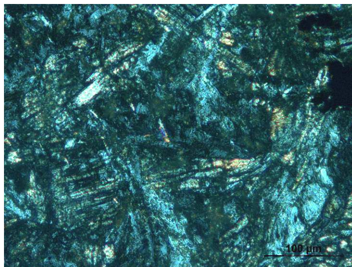
Figura 8 – Basalto riequilibrato in condizioni metamorfiche di grado molto basso, in cui sono riconoscibili relitti di plagioclasio (più chiari) e clinopirosseno (più scuri) con abito scheletrico, che indicano il rapido raffreddamento subito dalla lava.
