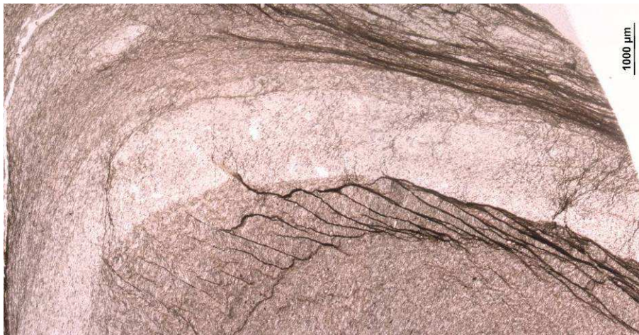
Figura 12 - Argilloscisto costituito da alternanze di livelli alternativamente più ricchi in fillosilicati o in quarzo, che definiscono una foliazione principale (S1±S2) deformata da pieghe aperte D3, con sviluppo di pressure solution cleavage di piano assiale.
