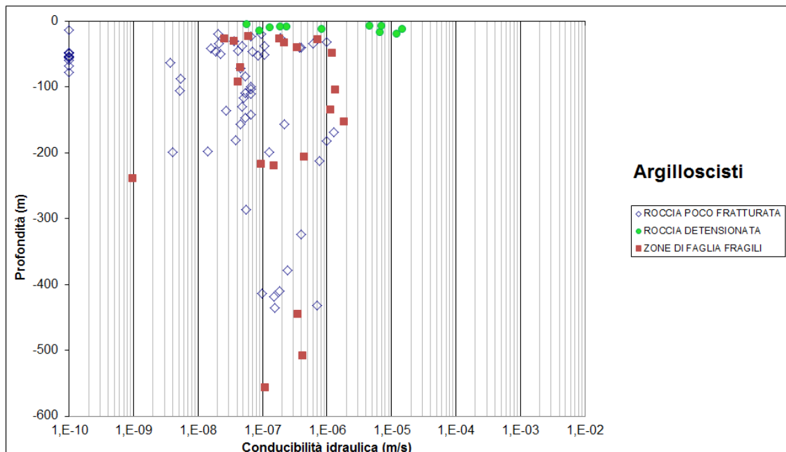
Figura 11. Grafico delle conducibilità idrauliche per gli argilloscisti (Argille a Palombini e argilliti in genere).
