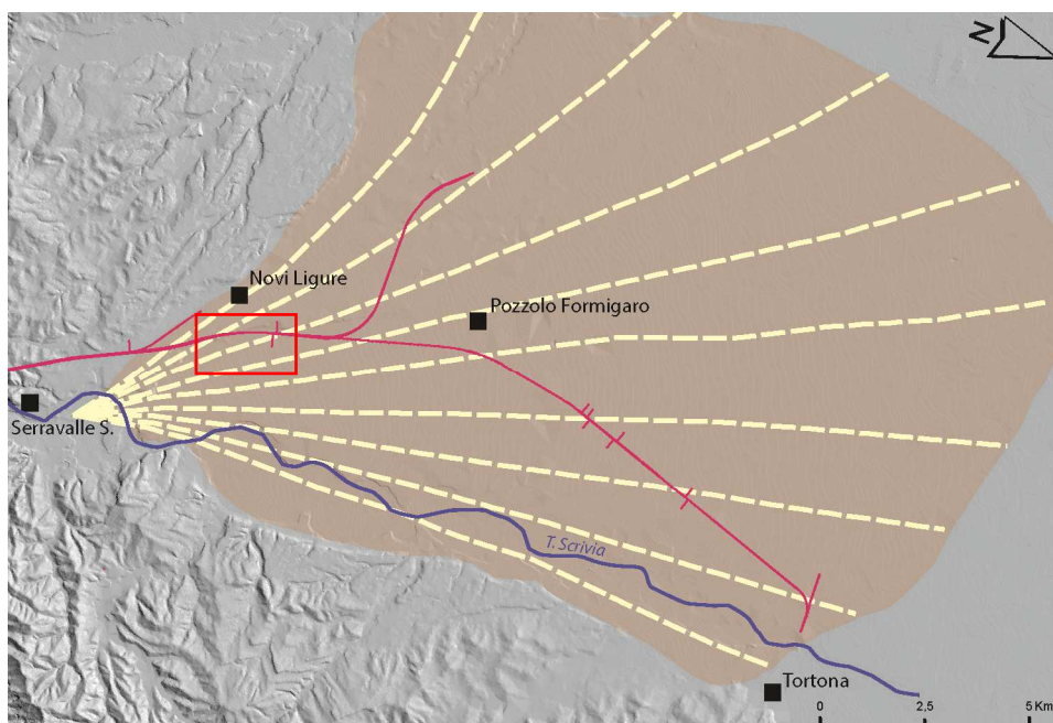
Figura 8 - Rappresentazione schematica dell'estensione areale del conoide del T. Scrivia, dei vari ordini di terrazzi da cui esso è disseccato. Il quadrato rosso indica la posizione dell'opera in progetto.
