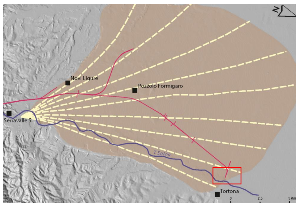
Figura 9: Rappresentazione schematica dell'estensione areale del conoide del T. Scrivia, dei vari ordini di terrazzi da cui esso è disseccato. Il quadrato rosso indica la posizione dell'opera in progetto.
