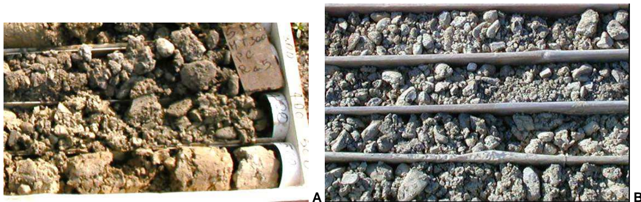
Figura 7 - Dettaglio dell'unità fl3b: (A): sondaggio XA301C070, (B): sondaggio XA301C087.
