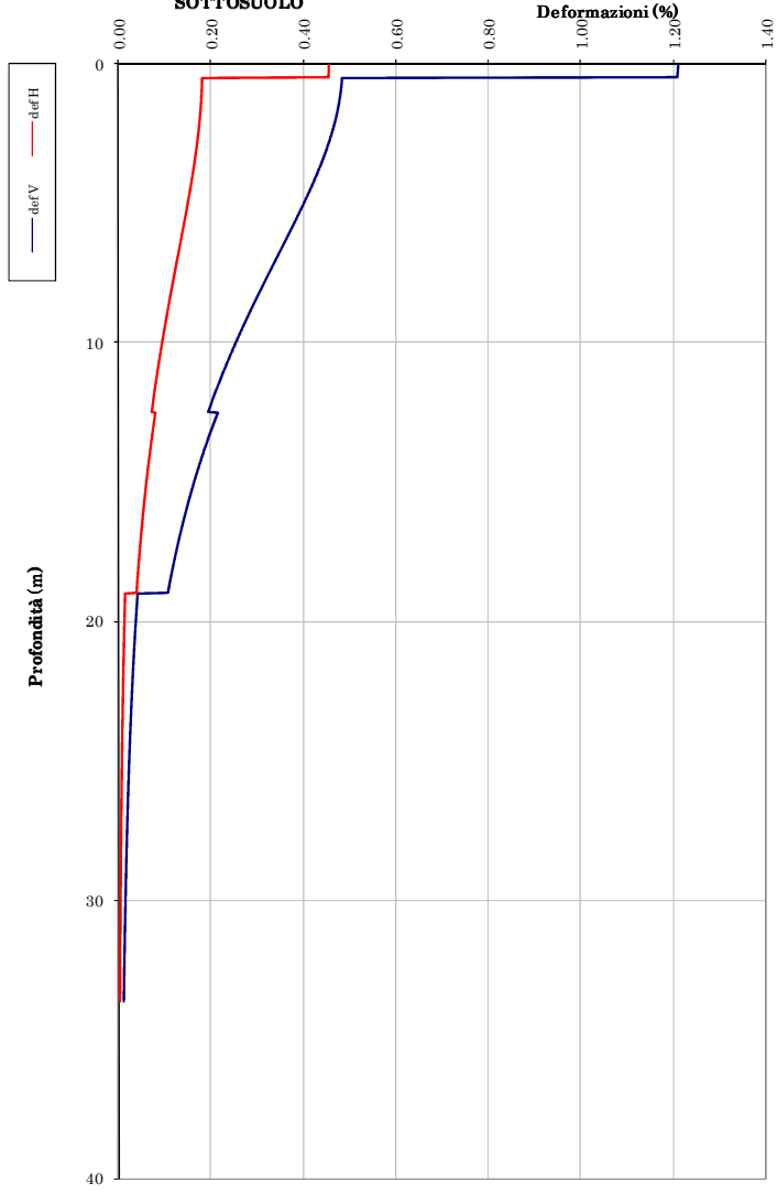
CURVE DI DEFORMAZIONE DEL SOTTOSUOLO
