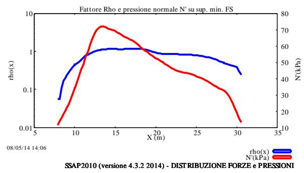
SSAP2010 (versione 4.3.2 2014) - DISTRIBUZIONE FORZE e PRESSIONI
