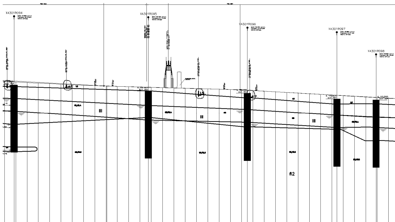
Figura 1. Caratteristiche idrogeologiche dell'area in esame
