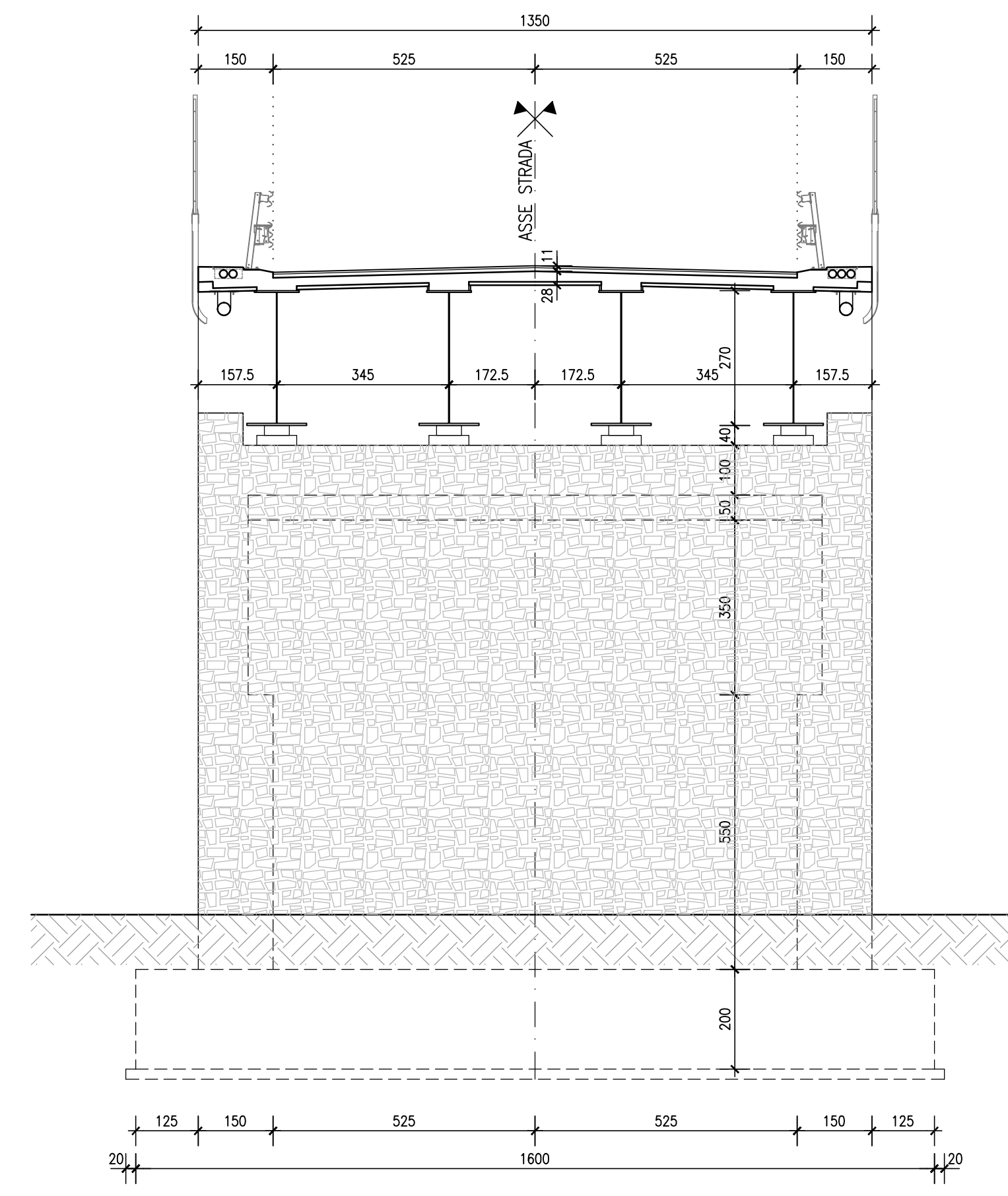
SEZIONE TRASVERSALE X-X scala 1:100
