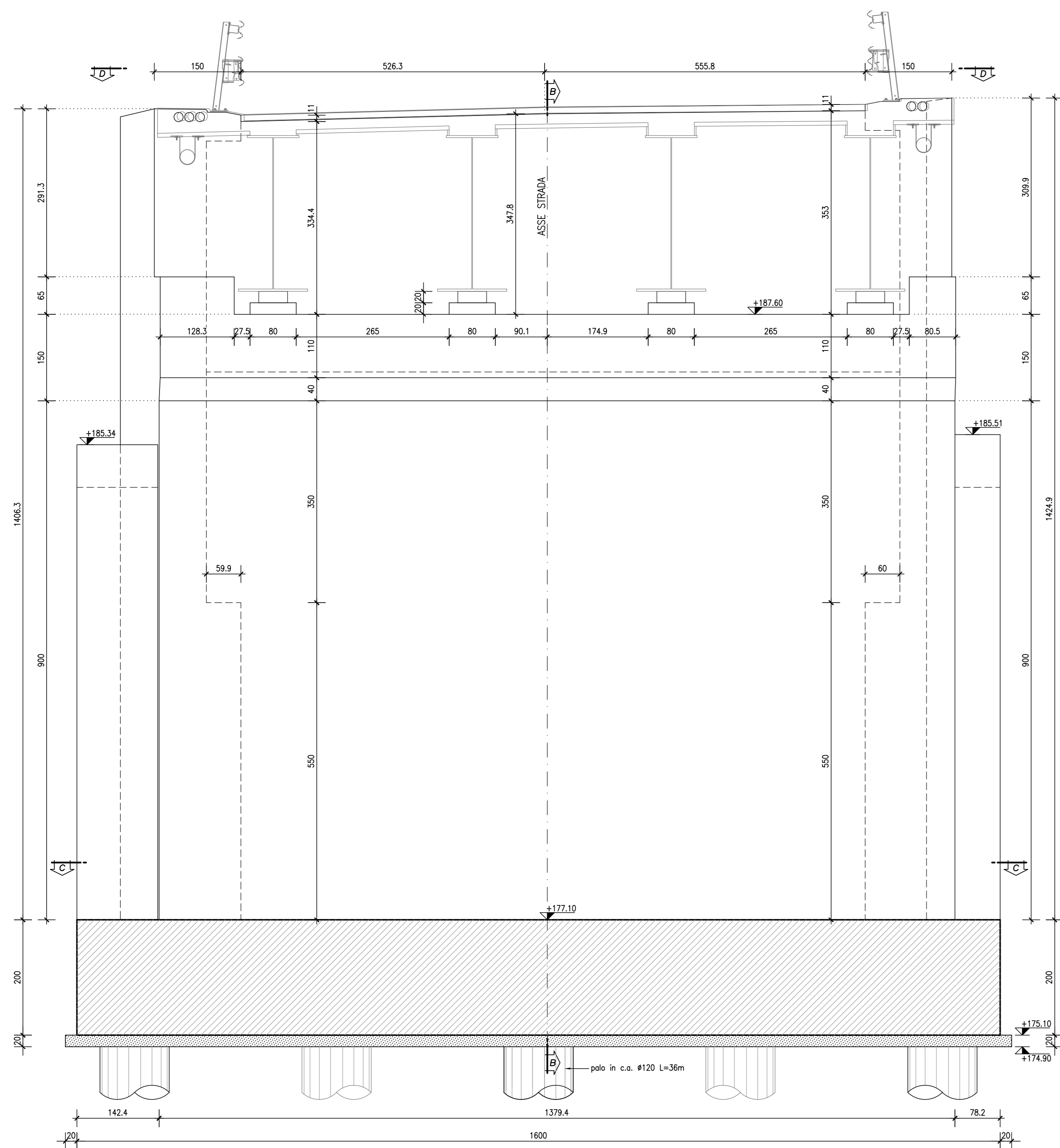
SEZIONE C-C scala 1:50
