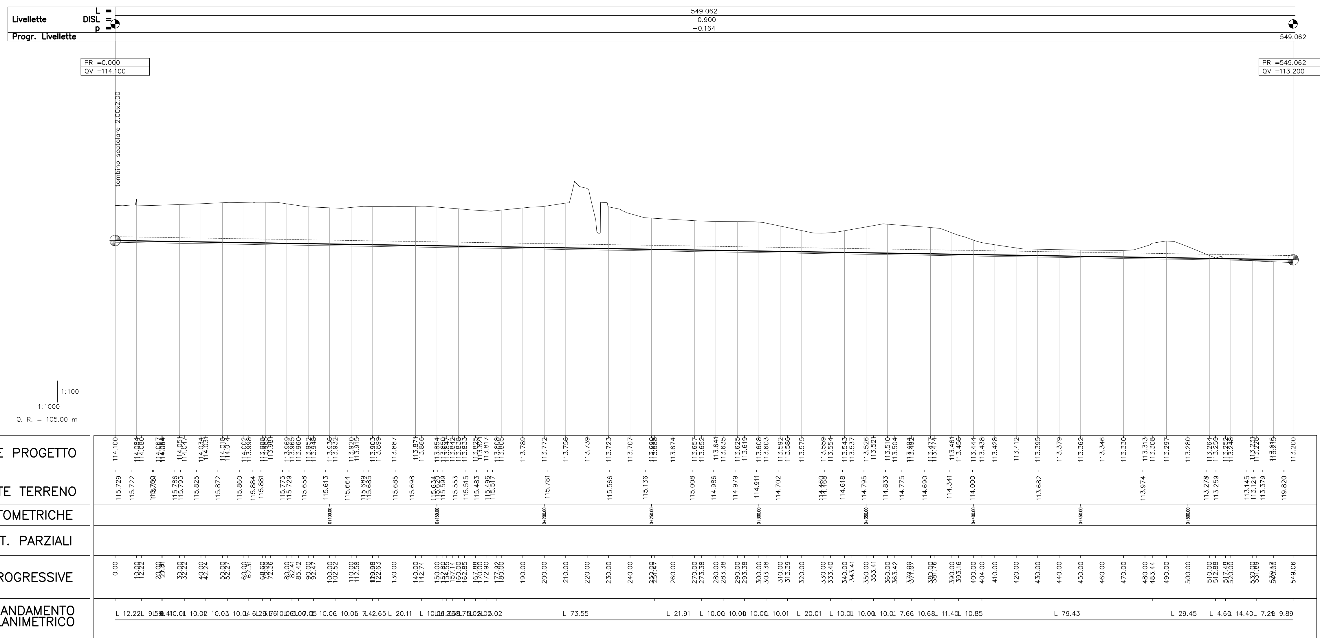
PROFILO LONGITUDINALE TRATTO 2 sc 1:1000
