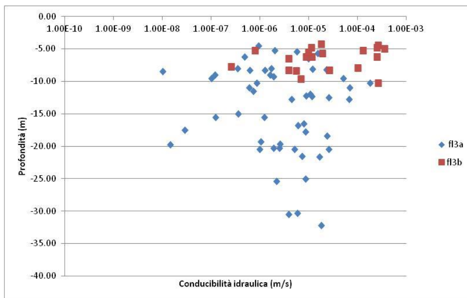
Figura 8. Grafico delle conducibilità idrauliche per i depositi alluvionali attuali (fl3), in cui vengono distinte le sub-unità fl3a ed fl3b da prove sui sondaggi del Progetto preliminare (R065, R067, R068, R069, R070, R071, R072, R073, R074, R075, R076, R087, R088, R088, R089, R092, R093, R094, R099, R100, R102, R103, R104, R106, R107, R109), del Progetto definitivo (SI07, SI09, SI10, SI13, SI14, SI47) e del Progetto esecutivo (L2-S32, L2-S34, L2-S32, L2-S43, L2-S47, L2-S48, L2-S50, L2-S52, L2-S15).
