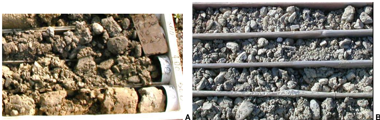
Figura 6 - Dettaglio dell'unità fl3b: (A): sondaggio XA301C070, (B): sondaggio XA301C087.
