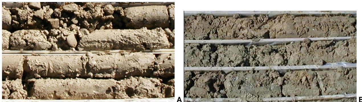
Figura 5 - Dettaglio dell'unità fl3a: (A): sondaggio XA301C072, (B): sondaggio XA301C087.
