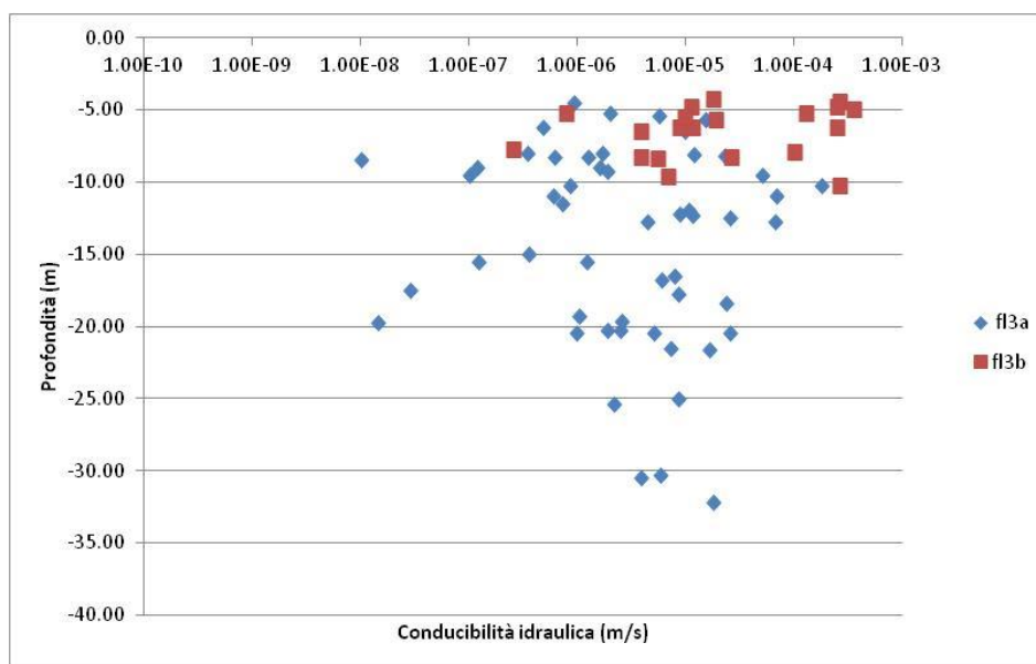
Figura 8. Grafico delle conducibilità idrauliche per i depositi alluvionali attuali (f13), in cui vengono distinte le sub-unità f13a ed f13b da prove sui sondaggi del Progetto preliminare (R065, R067, R068, R069, R070, R071, R072, R073, R074, R075, R076, R087, R088, R088, R089, R092, R093, R094, R099, R100, R102, R103, R104, R106, R107, R109), del Progetto definitivo (SI07, SI09, SI10, SI13, SI14, SI47) e del Progetto esecutivo (L2-S32, L2-S34, L2-S32, L2-S43, L2-S47, L2-S48, L2-S50, L2-S52, L2-S15).
