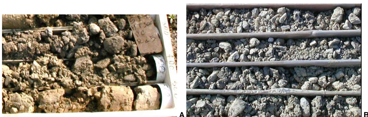
Figura 6 - Dettaglio dell'unità f13a: (A): sondaggio XA301C070, (B): sondaggio XA301C087.
