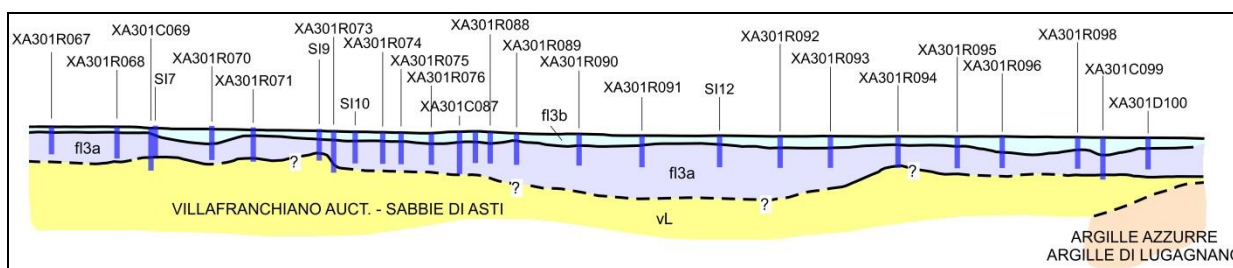
Figura 5 – Andamento dei principali limiti stratigrafici desunto dai dati dei sondaggi realizzati in fase di progetto preliminare. I sondaggi rappresentati hanno lunghezza di 30-40 m.
